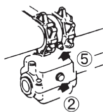
ギヤボックス (ビータ) コンベヤ軸
