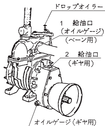
ポンプ(ベーン, ギャ)(TVC3832)
