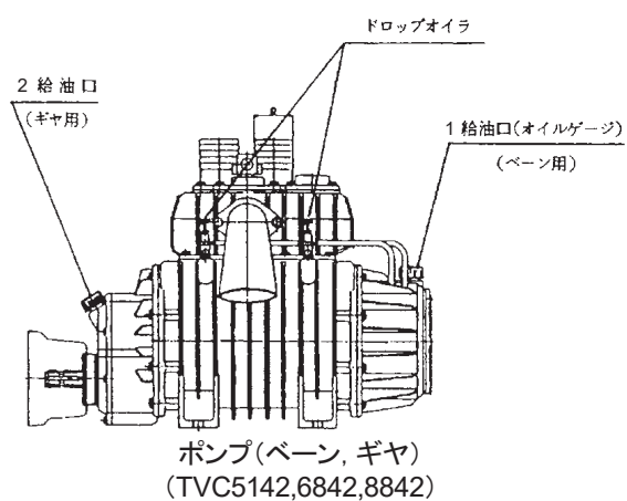
オイル (ベーン用) レベル
