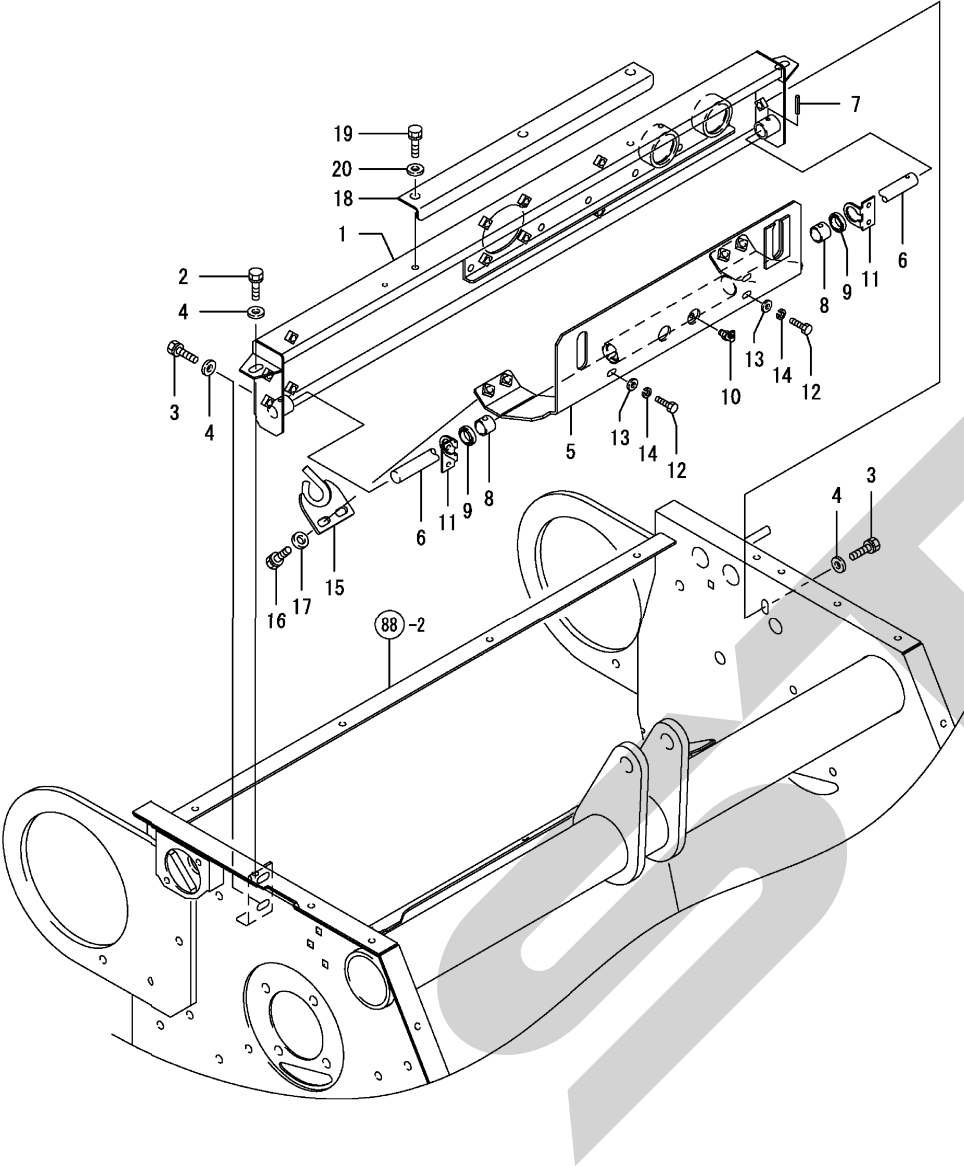
Fig. 95. バインディング
