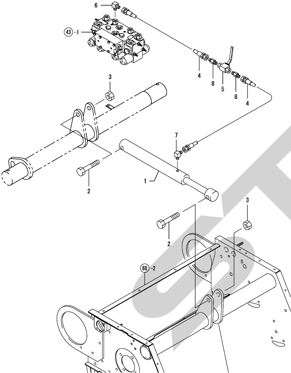
Fig.108. 油圧（ゲート）
