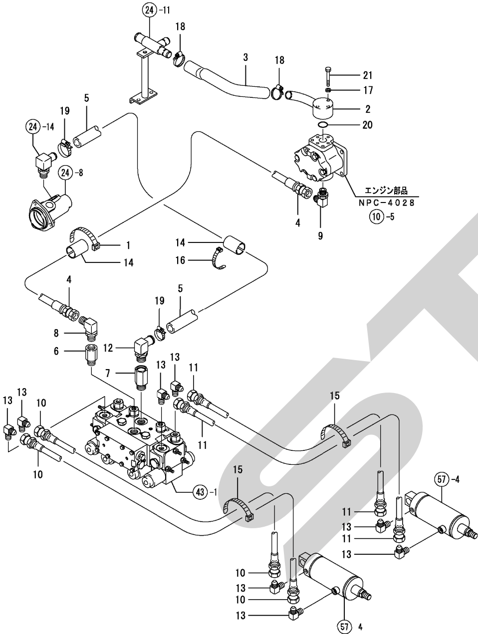
Fig. 41. 配 管
