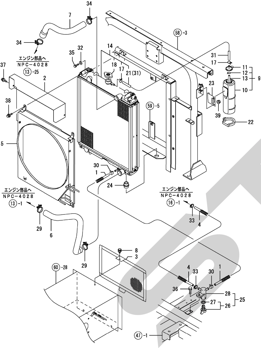
Fig. 7. ラジエータ
