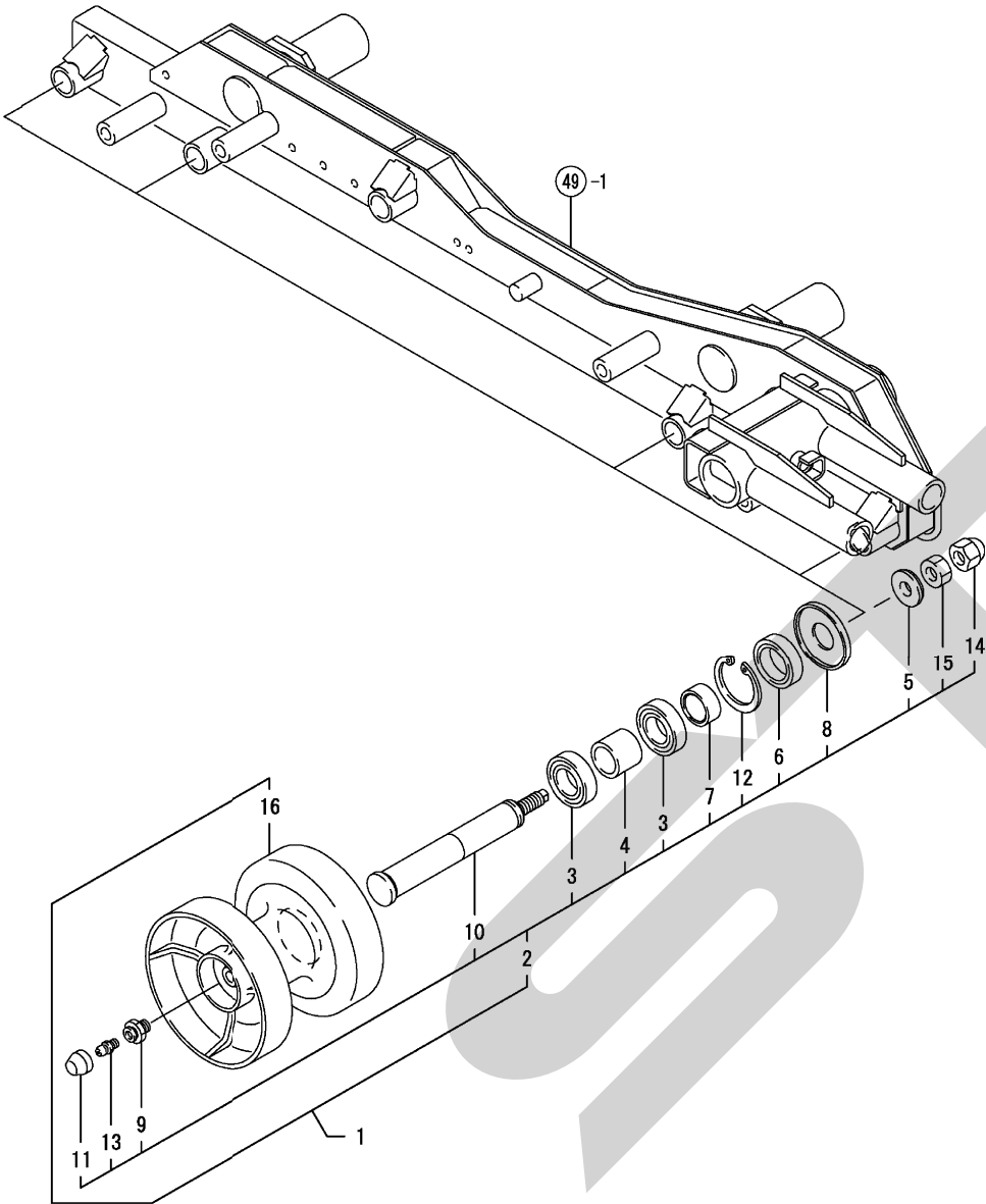
Fig. 51. トラックローラ
