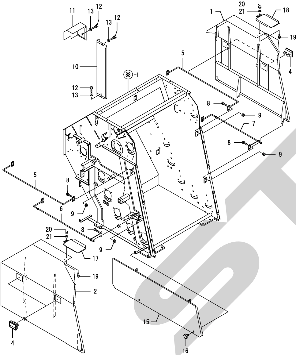
Fig. 78. カバ ー
