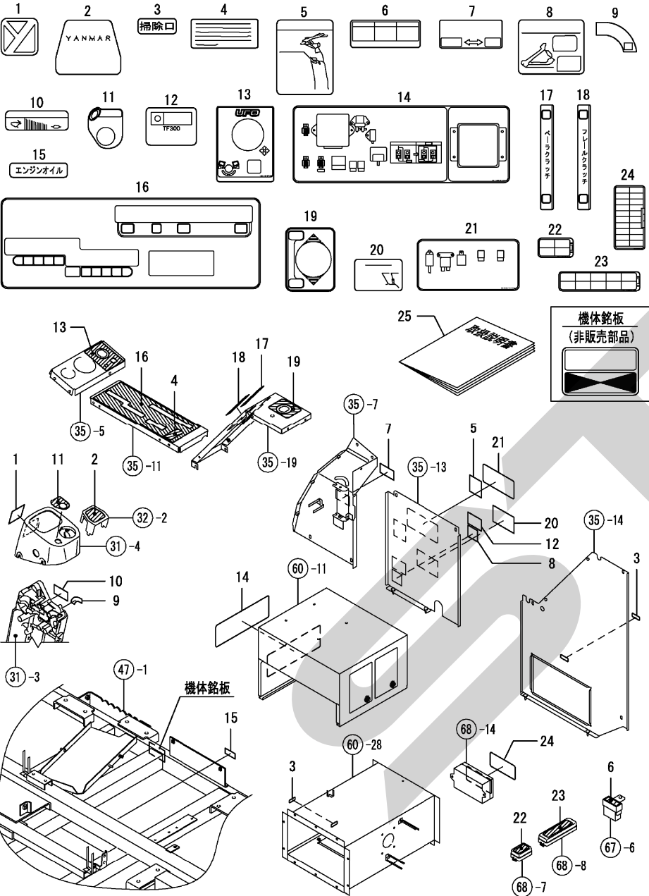
Fig. 71. 銘板, 付属品
