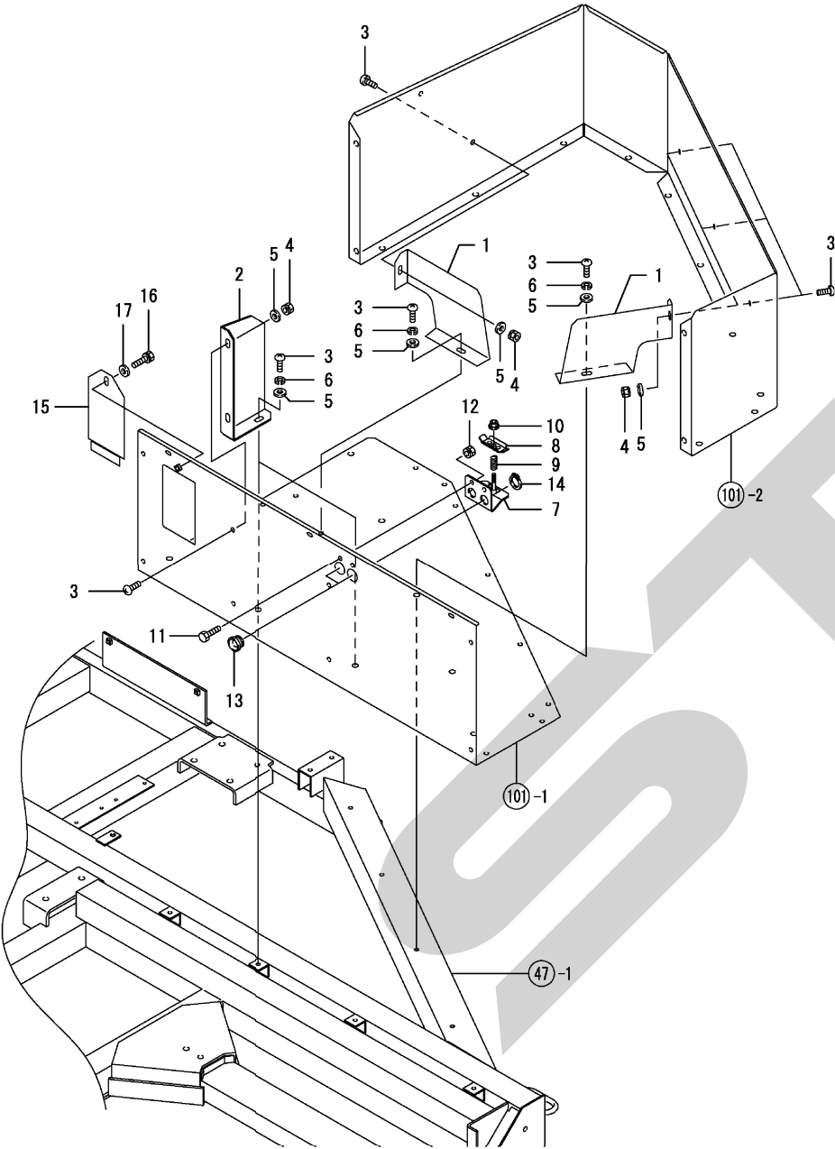
Fig. 102. トワインケーシング
