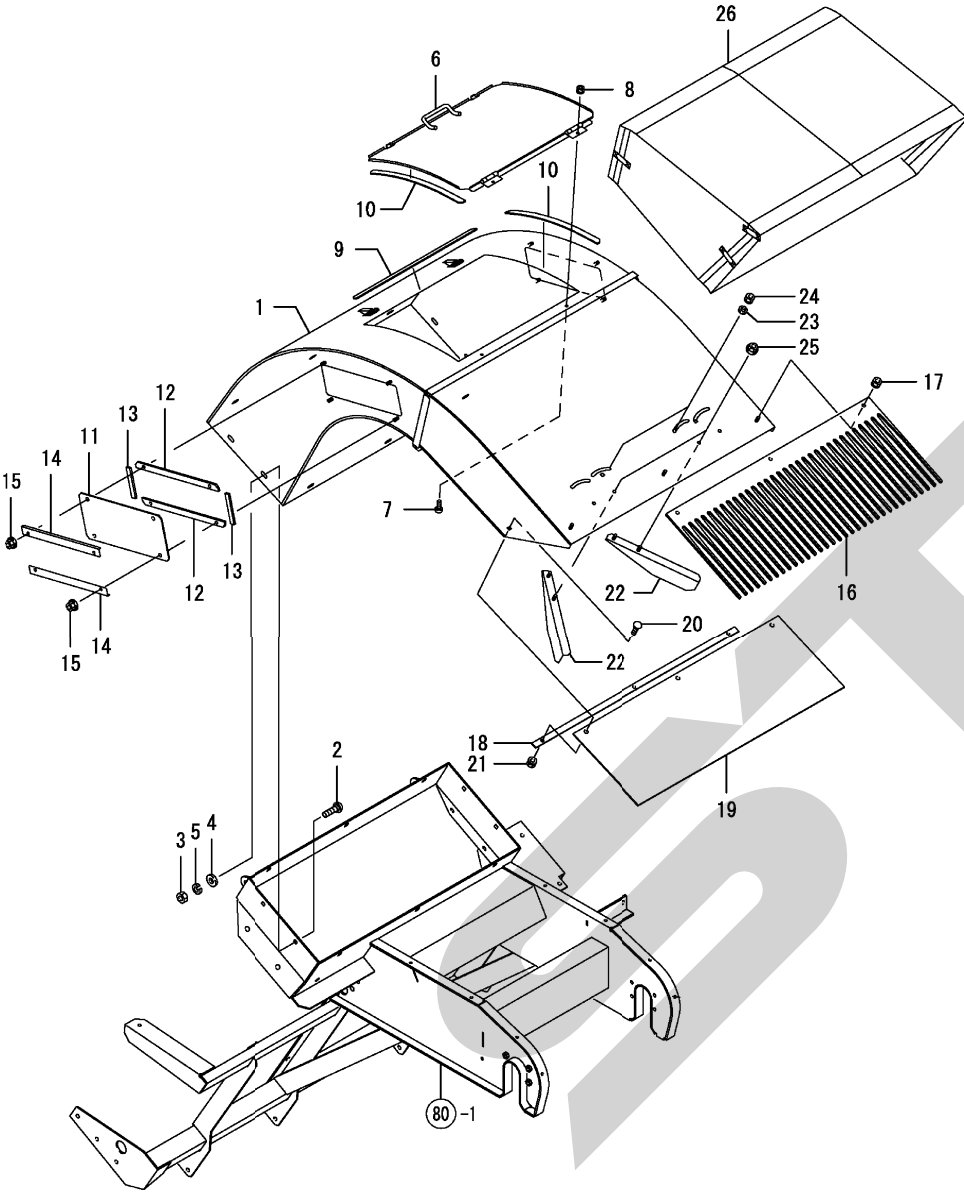
NPC-4029 Fig. 75. シュート
