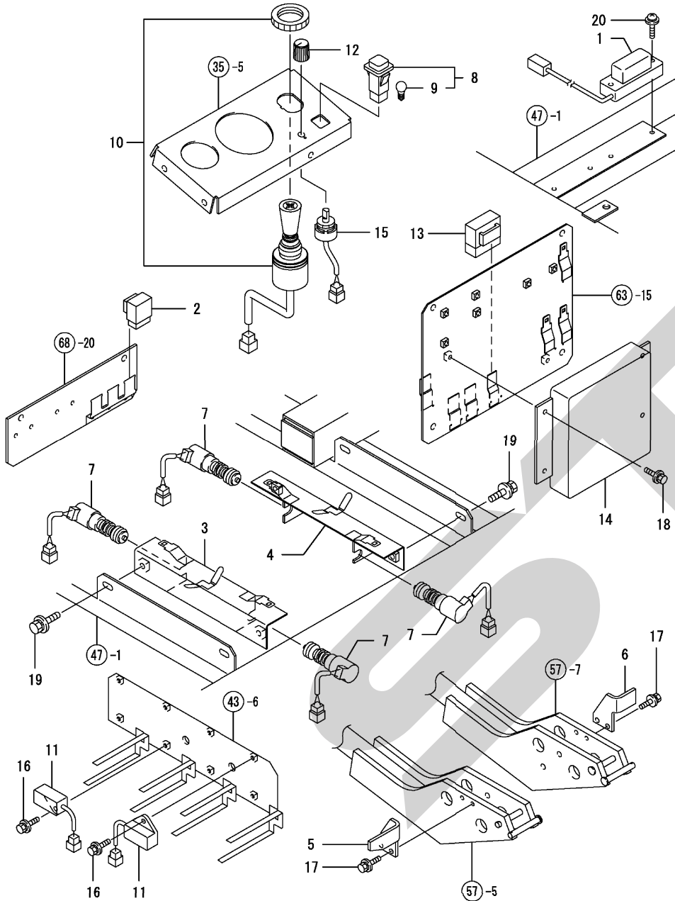
NPC-4029 Fig. 70. 水平制御
