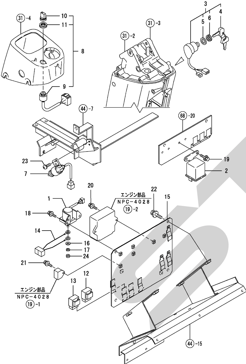
Fig. 63. エンジン電装
