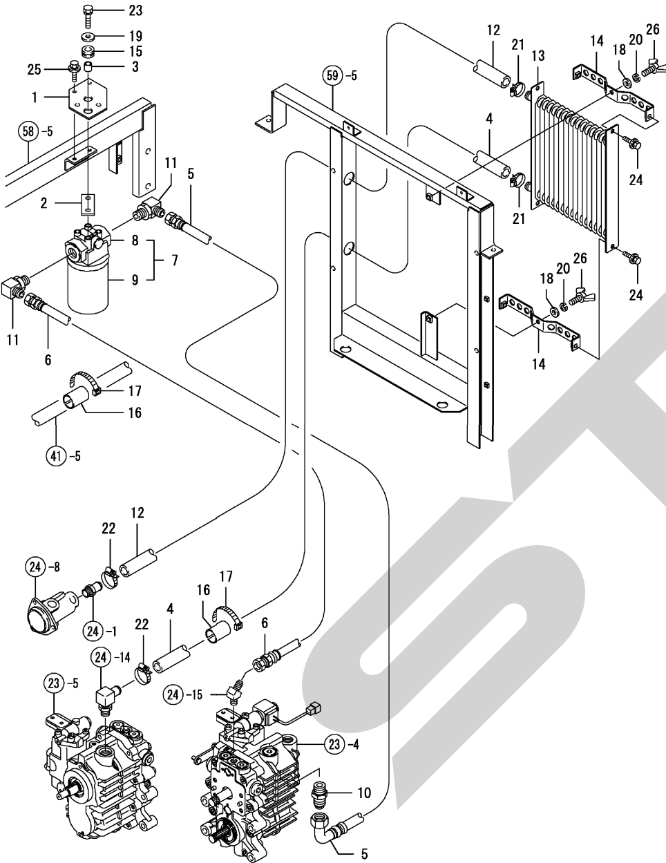
Fig. 42. 配管 (HST)
