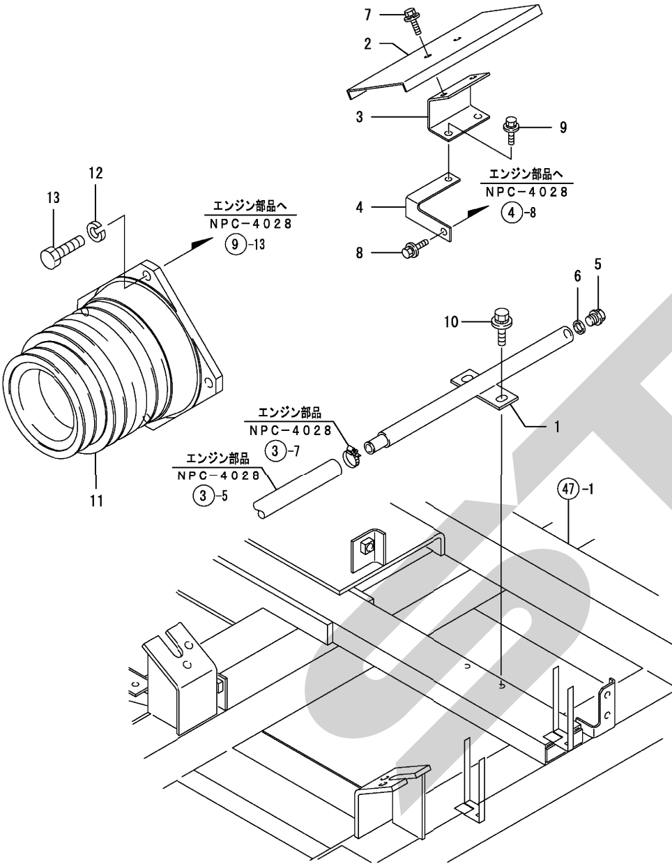
NPC-4029 Fig.1. エンジン関連
