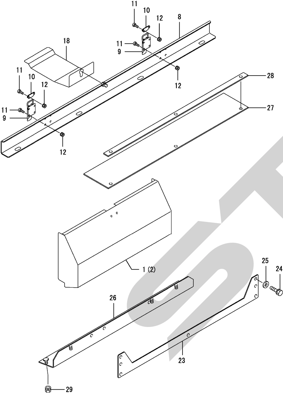
Fig. 110. トワインカバー
