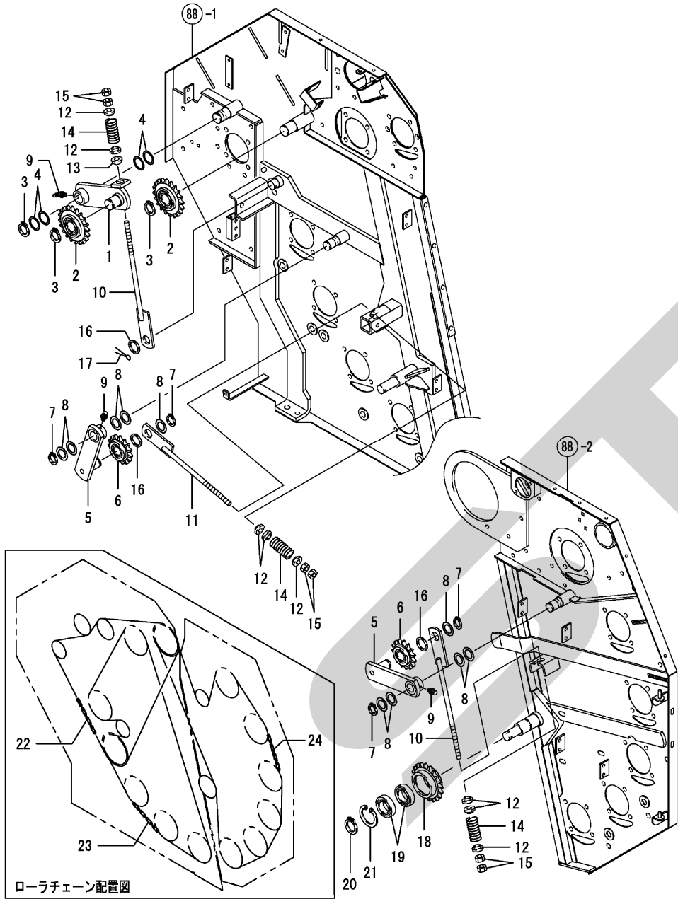
Fig. 92. ローラ駆動
