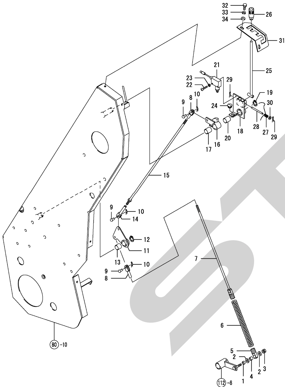
Fig. 113. OKリフト
