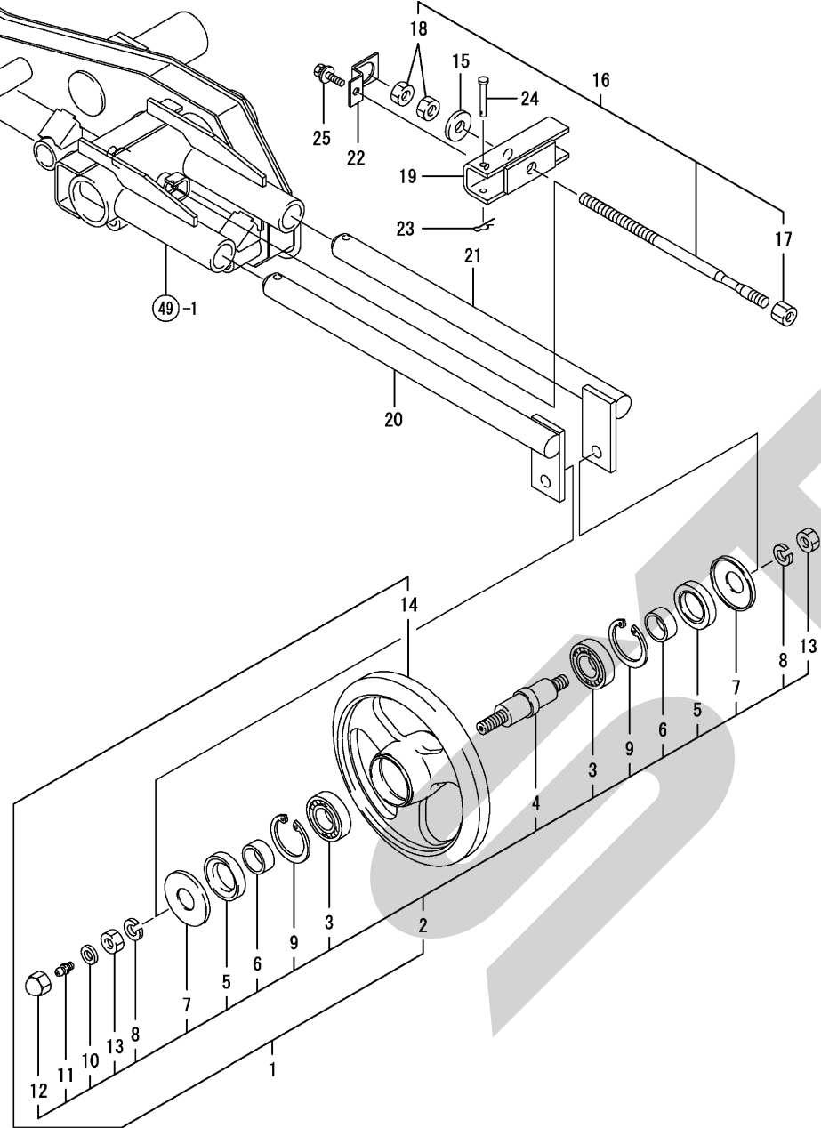
NPC-4029 Fig. 50. アイドラ
