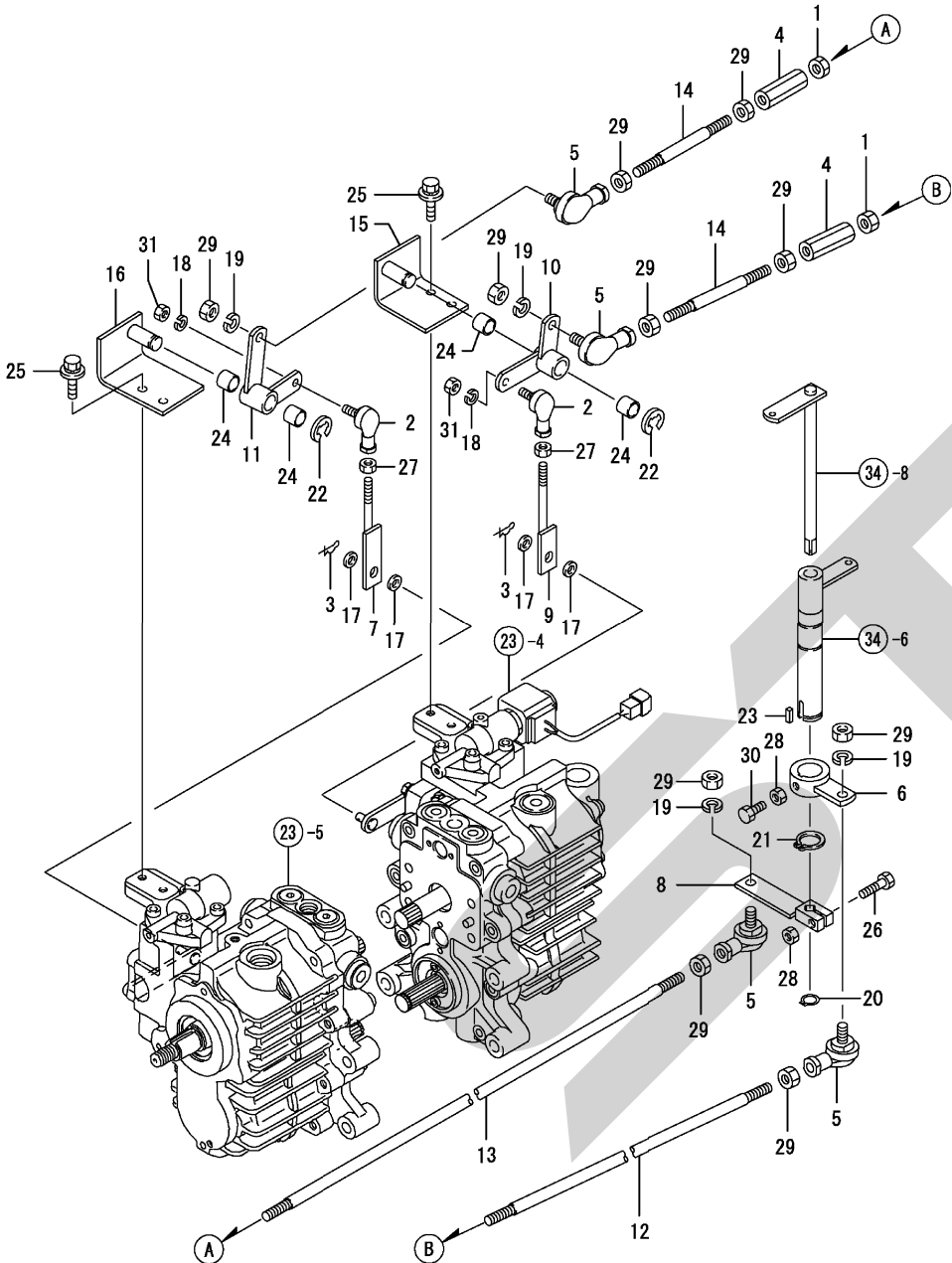
Fig. 39. 操作ロッド
