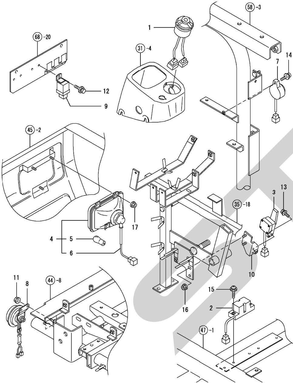
Fig. 64. 保安作業灯
