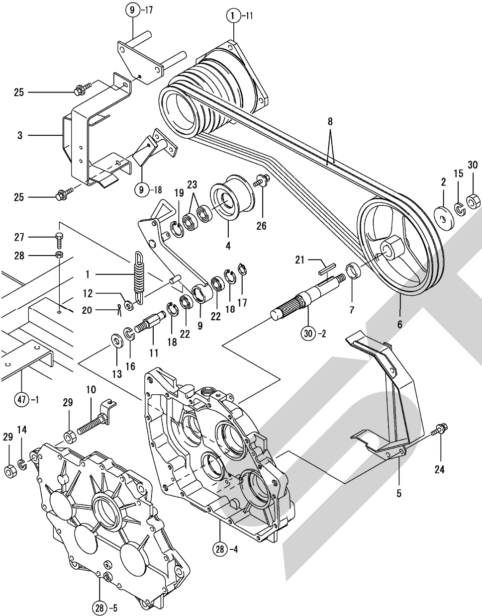
Fig. 27. ベーラベルト
