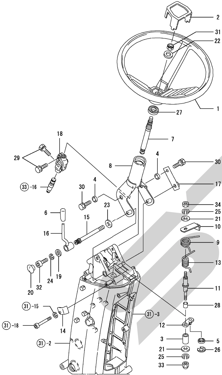
Fig. 32. ステアリング
