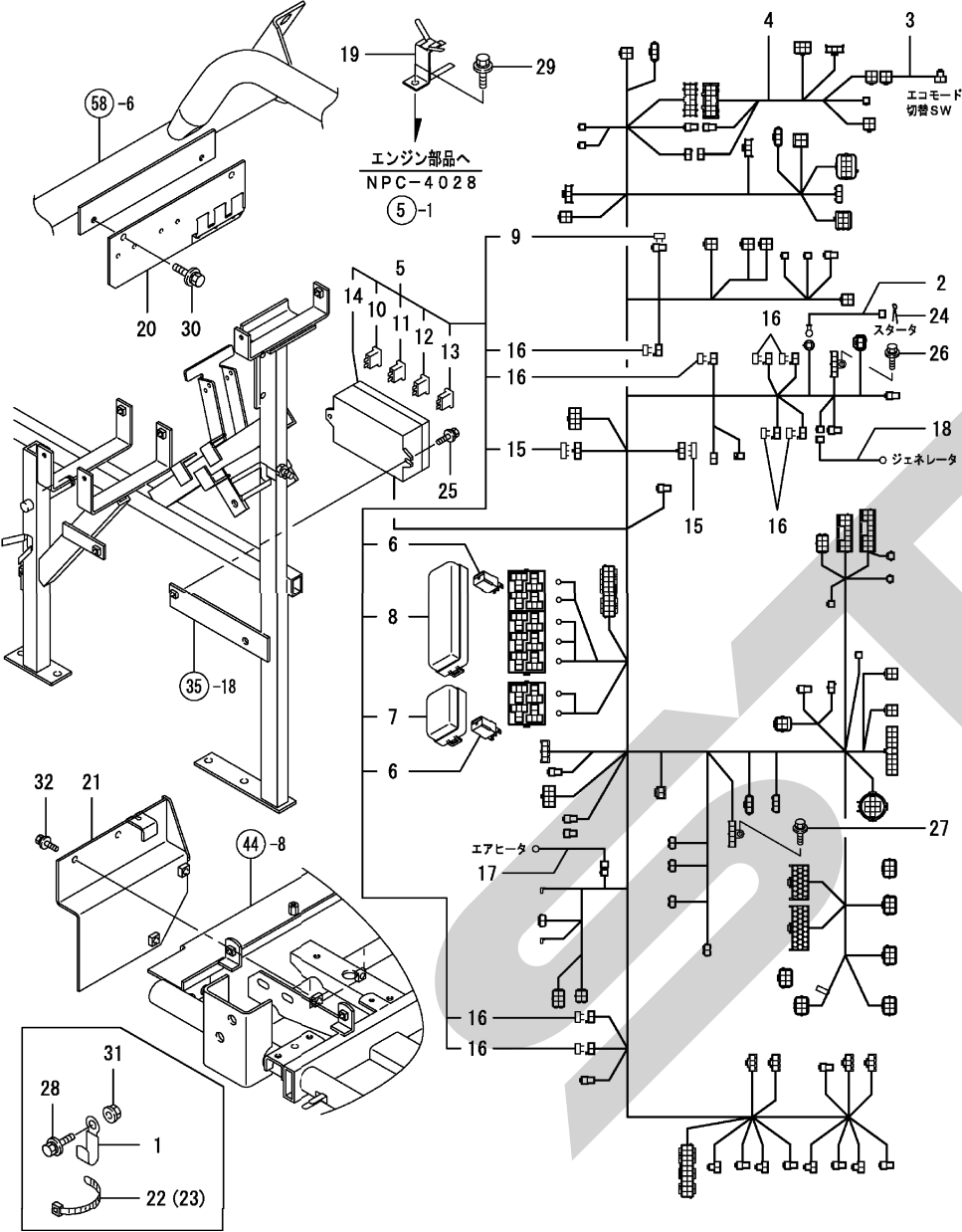
Fig. 68. ワイヤーハーネス
