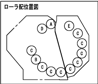
Fig. 89. ローラ
