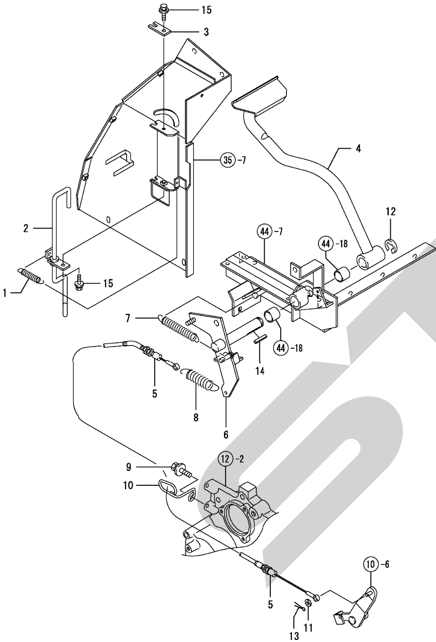
Fig. 36. ブレーキ操作
