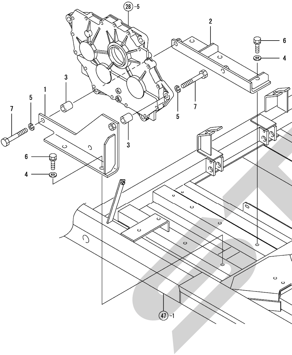
Fig. 29. ケース取付
