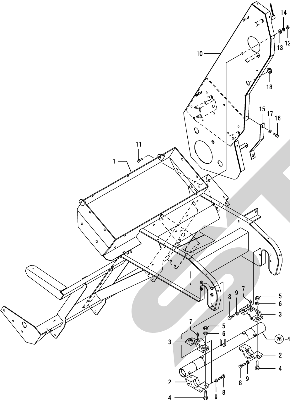
Fig. 80. 刈取りフレーム
