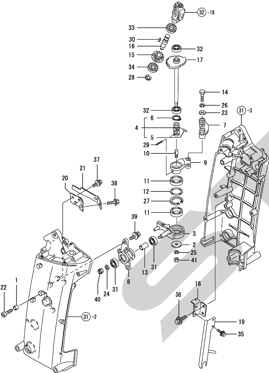
Fig. 33. ステアリング操作（１）
