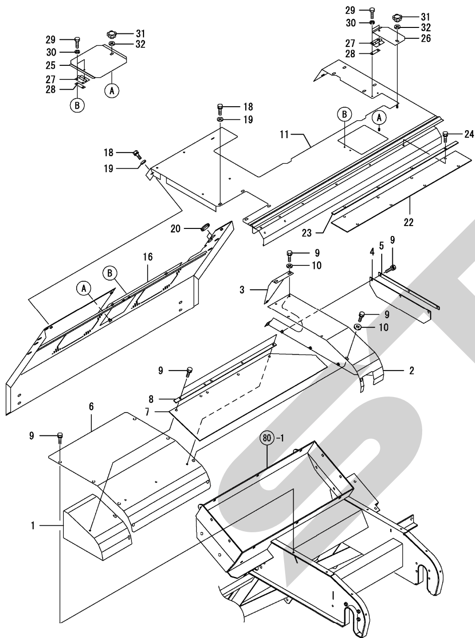
Fig.103. カバー
