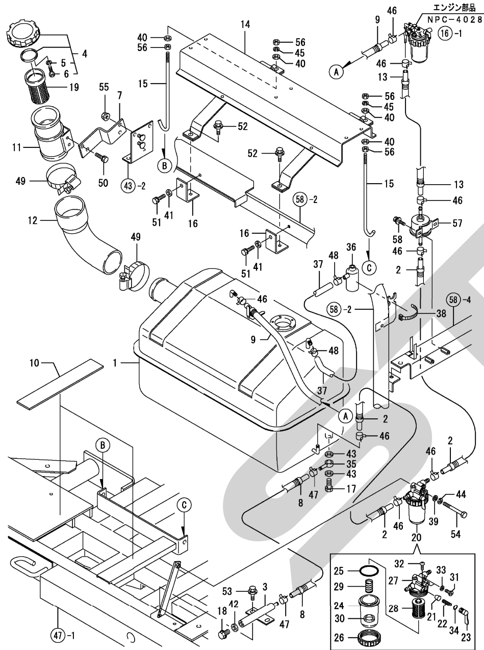
Fig. 4. 燃料タンク、フィードポンプ
