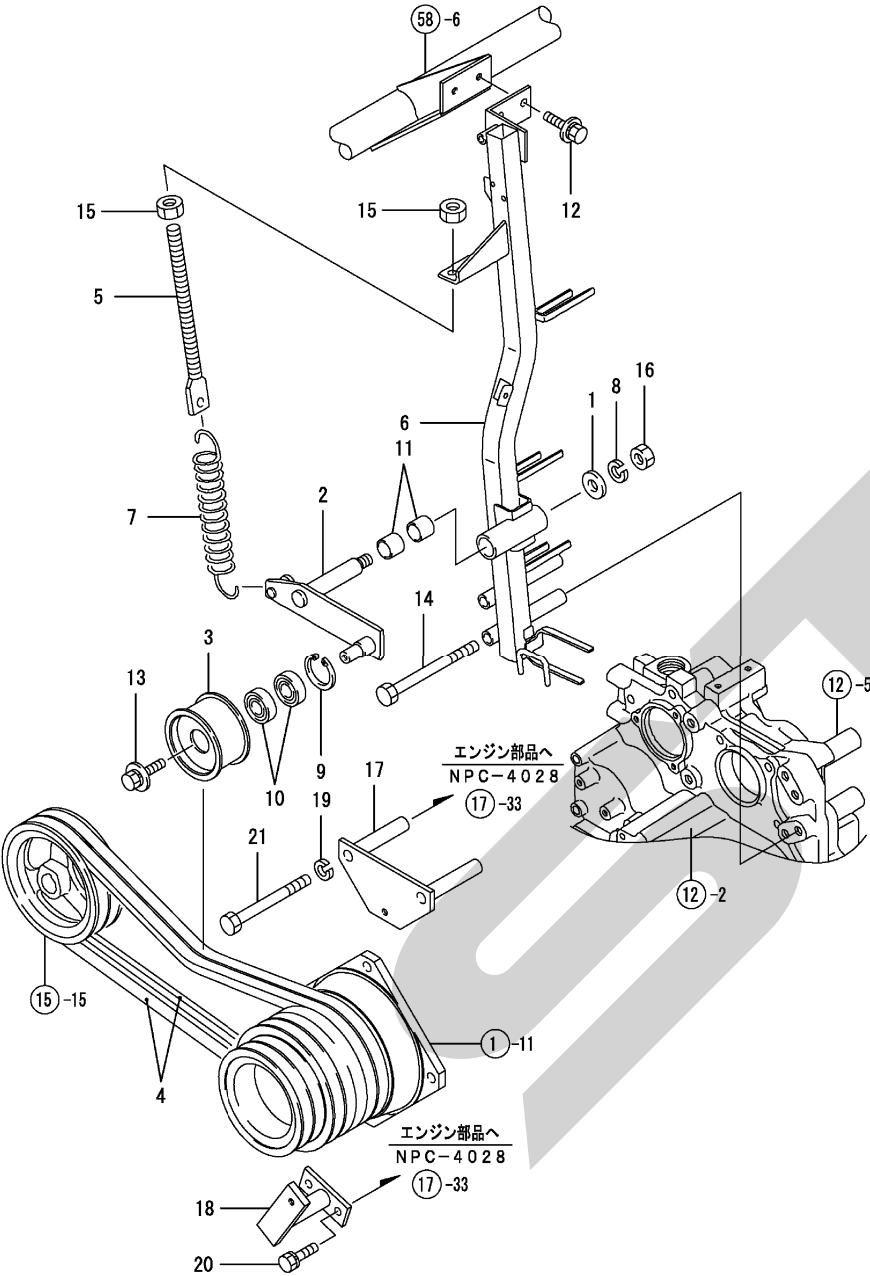
Fig. 9. 走行ベルト、ベルト押え
