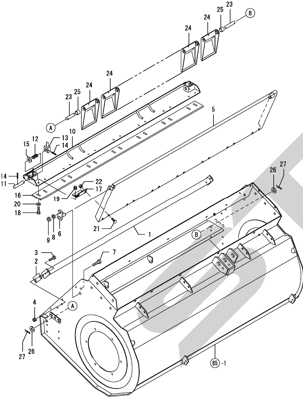
Fig. 86. ケーシング
