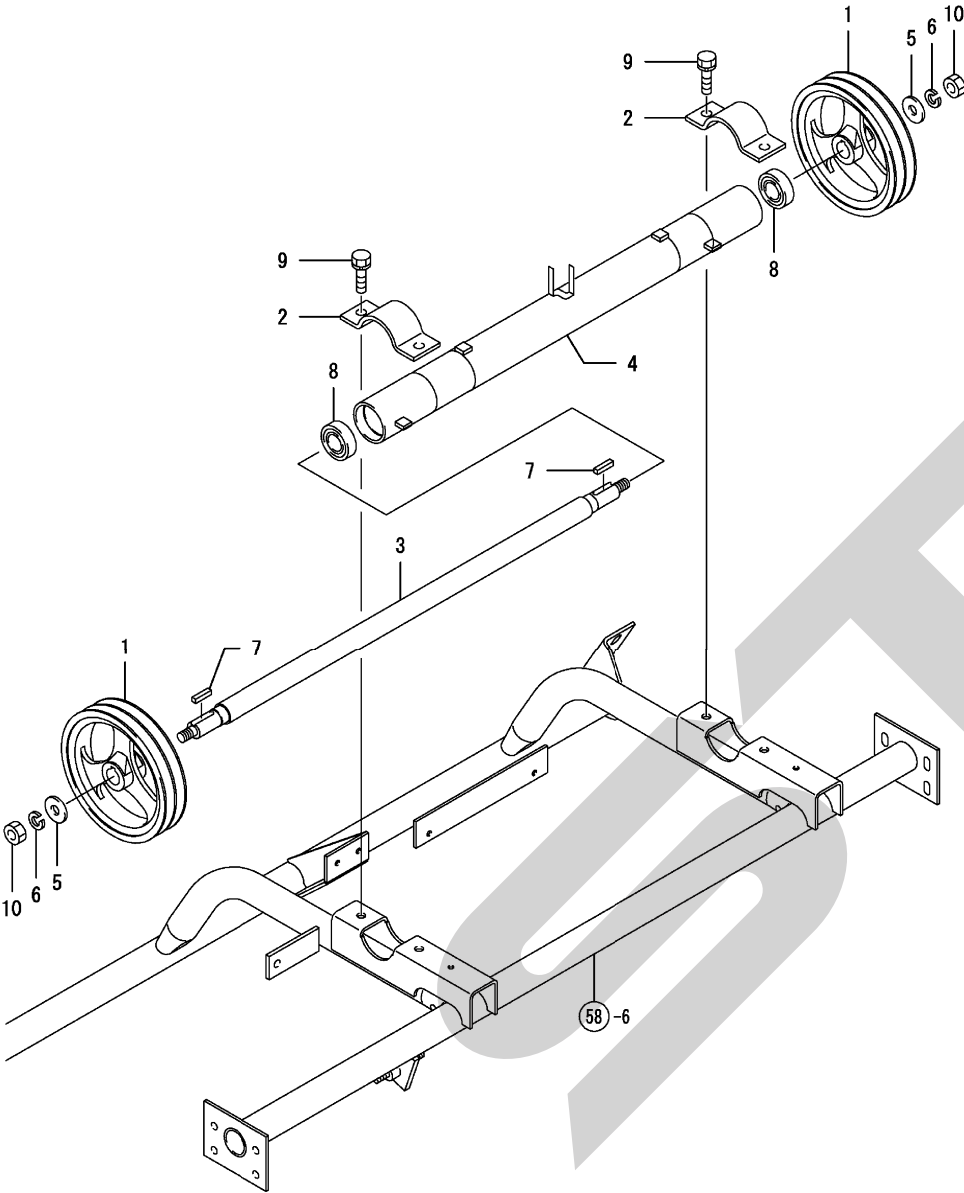
Fig. 26. フレールケース
