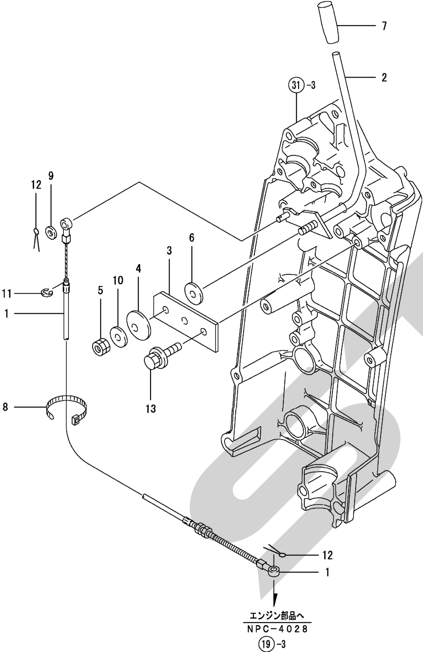
Fig. 3. エンジンコントロール
