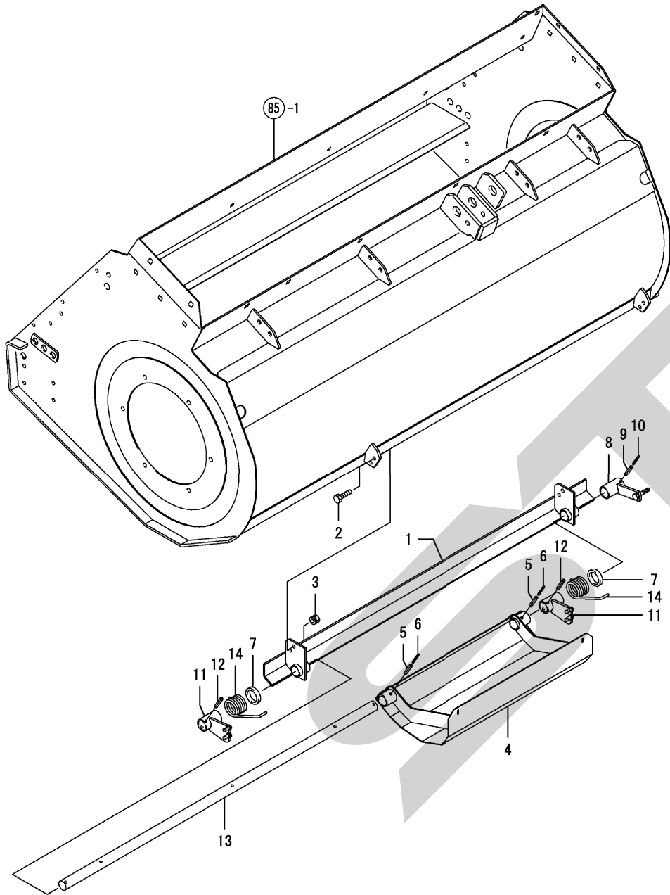
Fig. 112. OKリフト
