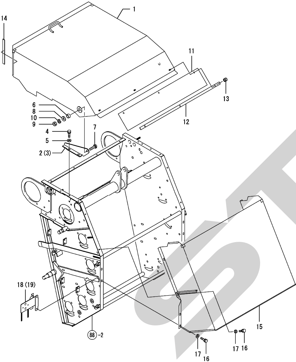
Fig. 77. エアシュート
