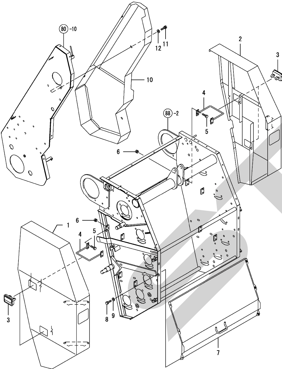
NPC-4029 Fig. 79. カバー
