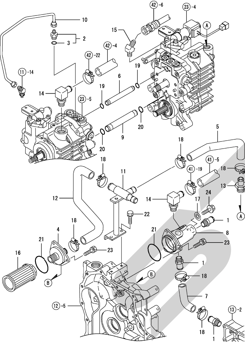
Fig. 24. 配 管
