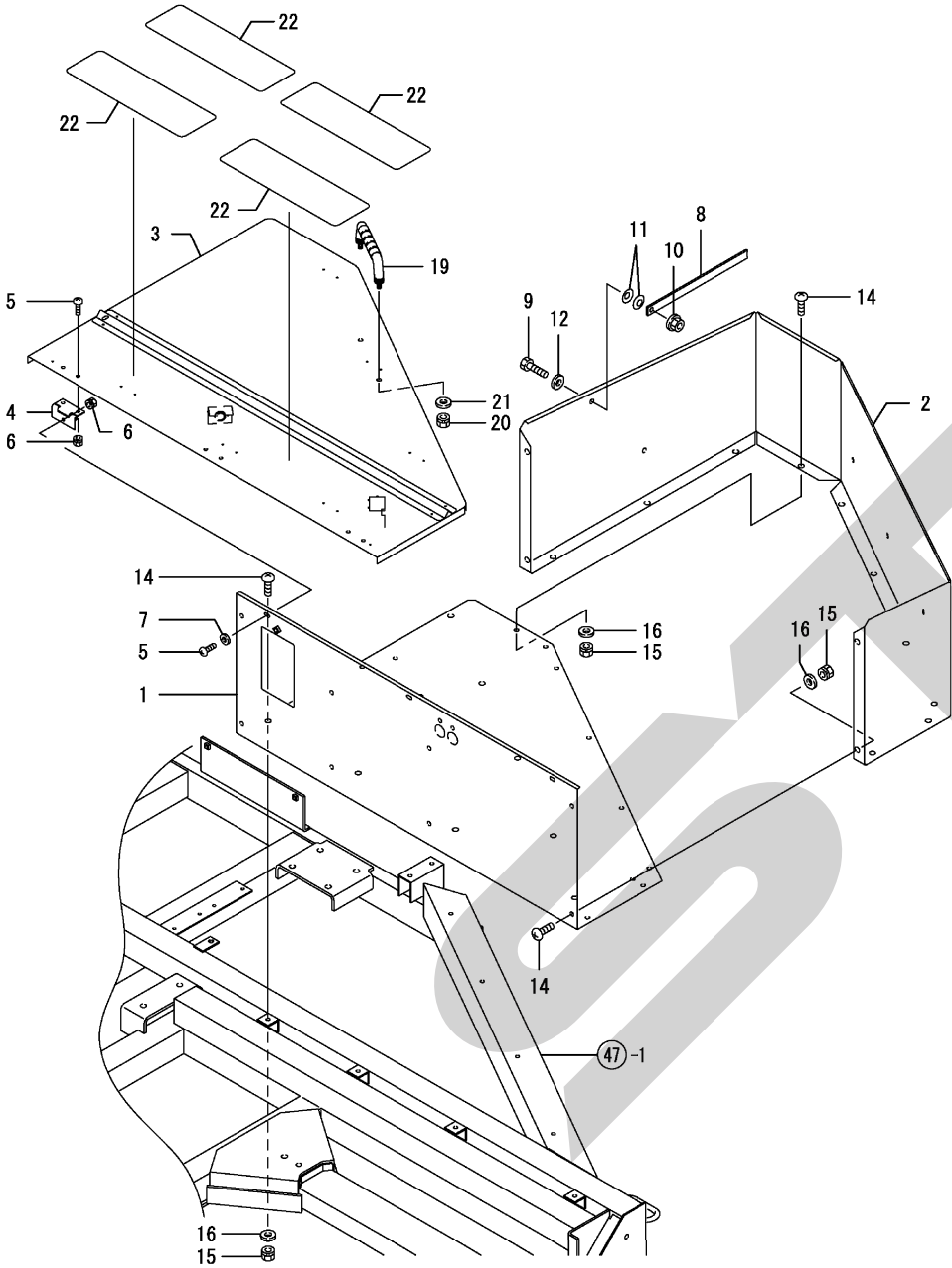
Fig. 101. トワインケーシング
