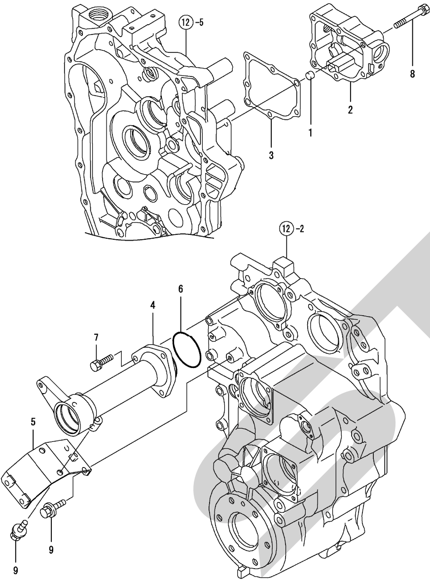
Fig. 13. サイドケース
