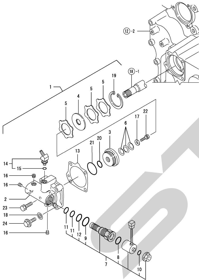
Fig. 11. ステアリングブレーキ
