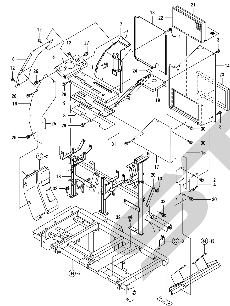
Fig. 35. サイドコラム
