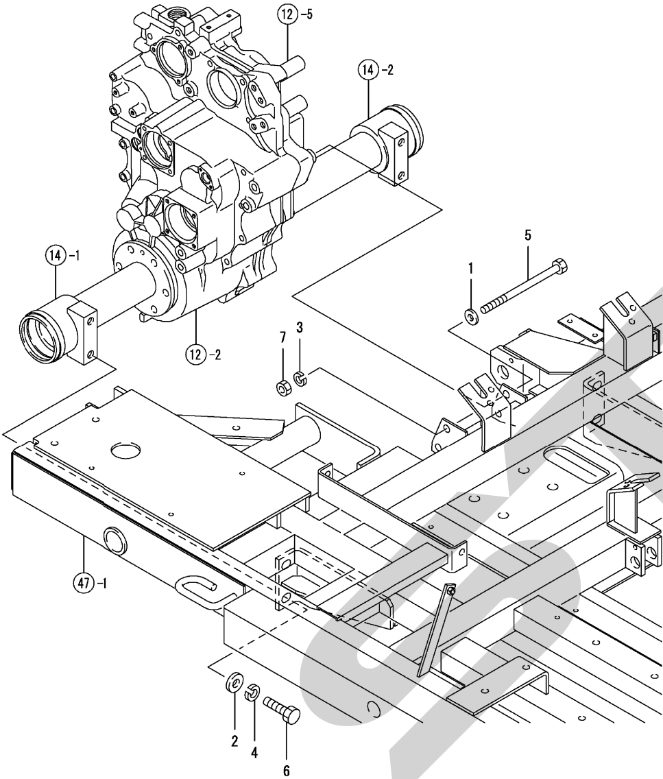
Fig. 48. ミッション取付
