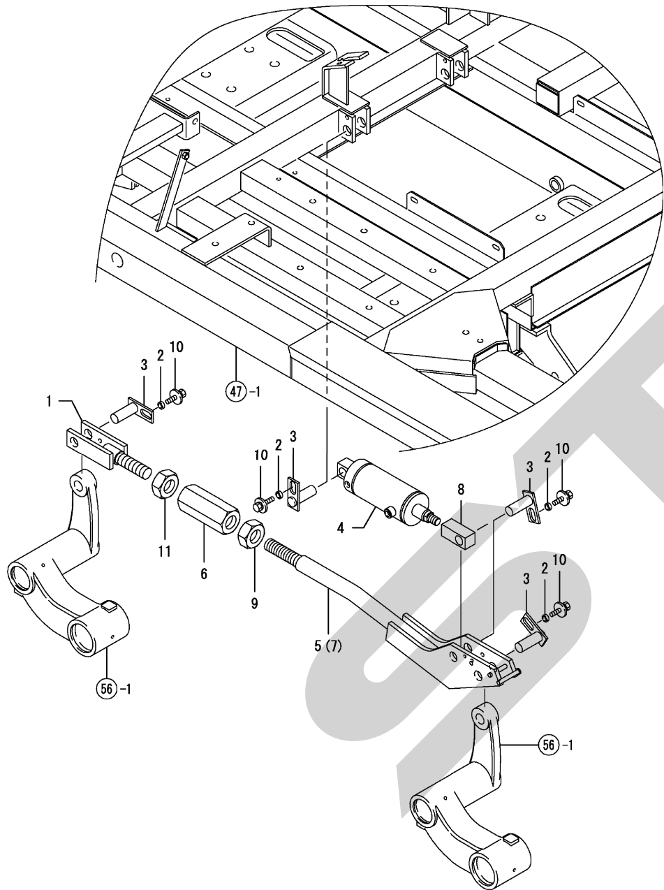
Fig. 57. スイング（２）
