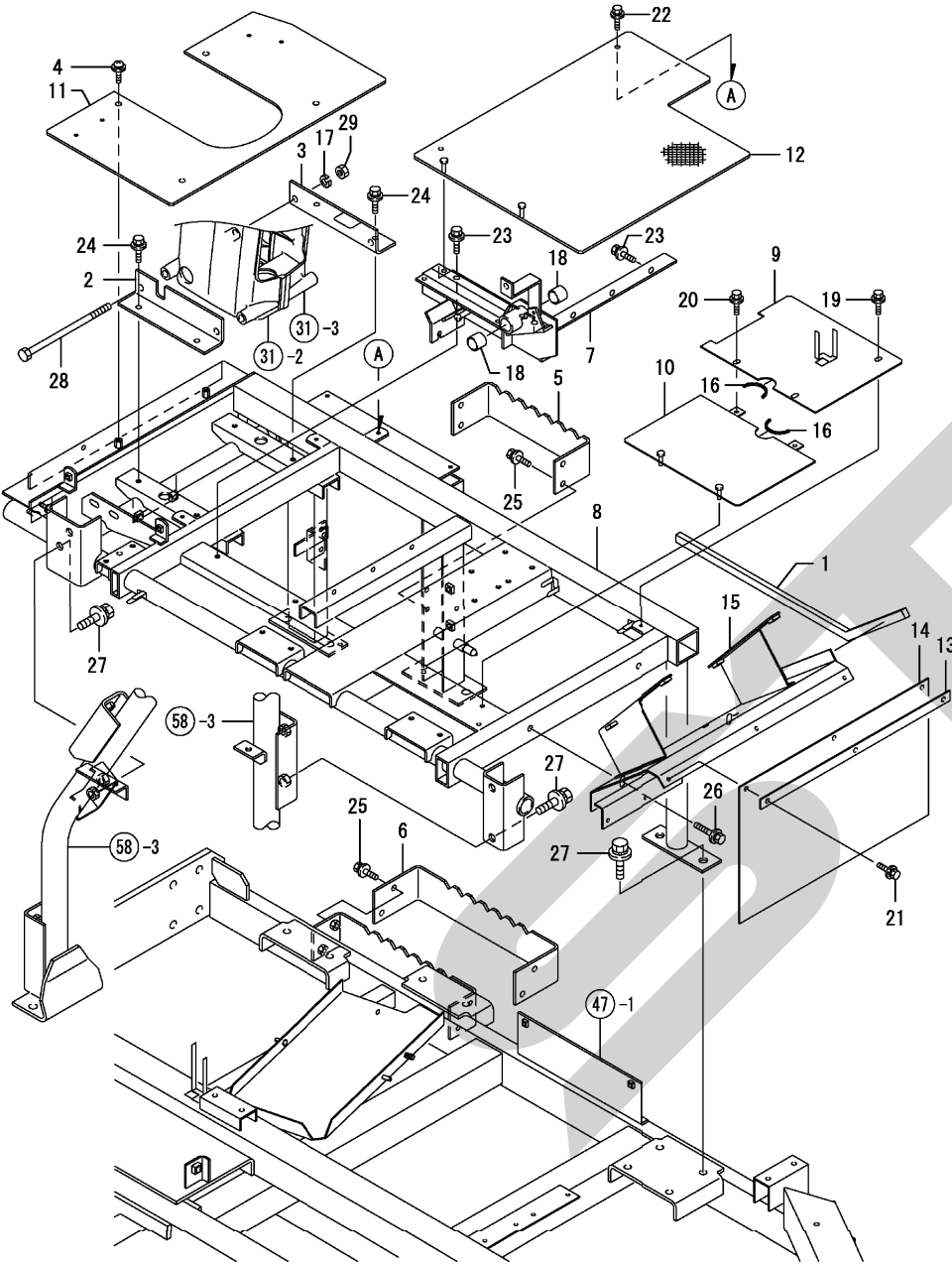
Fig. 44. ステップフレーム
