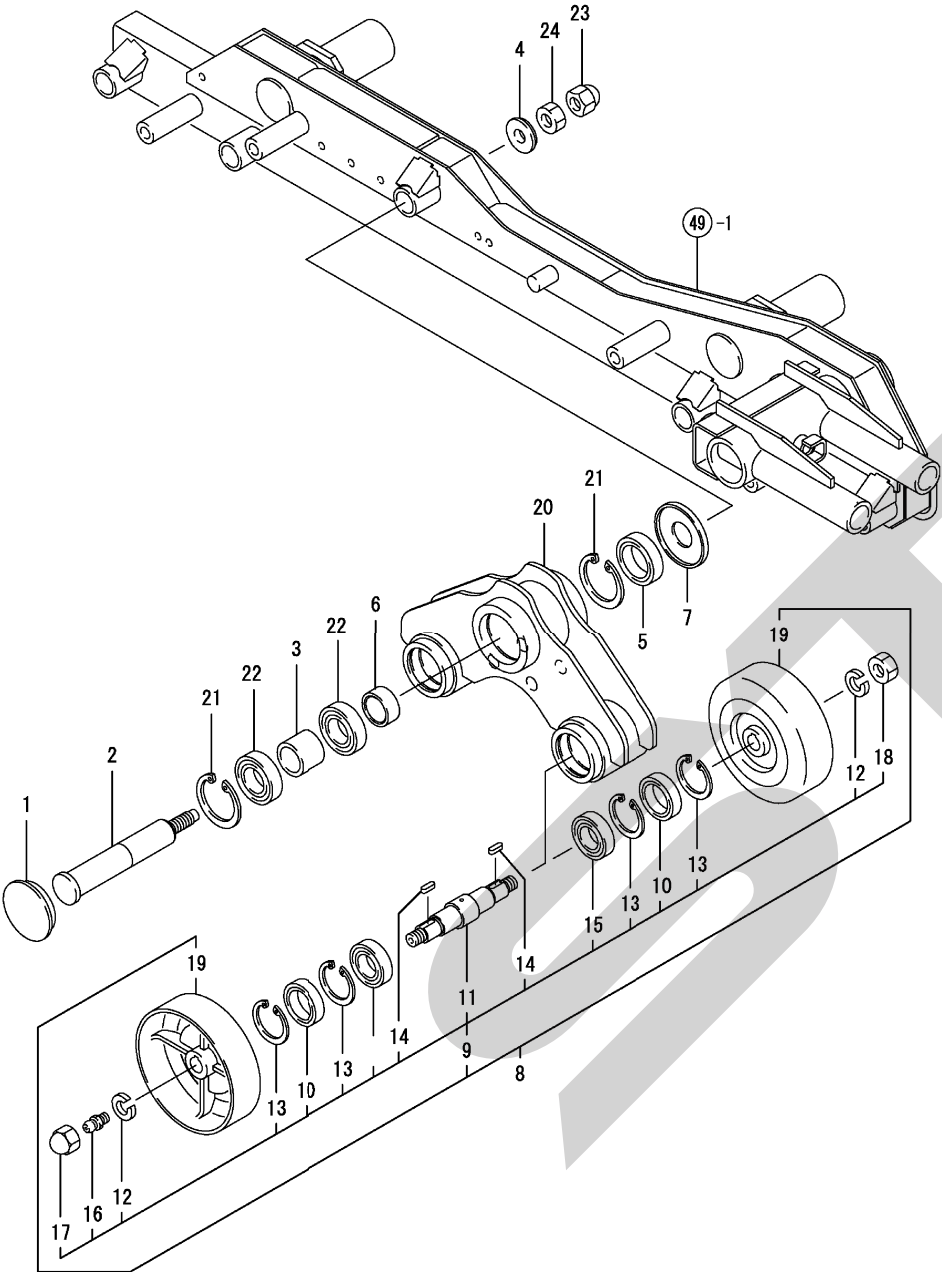
Fig. 52. イコライザー
