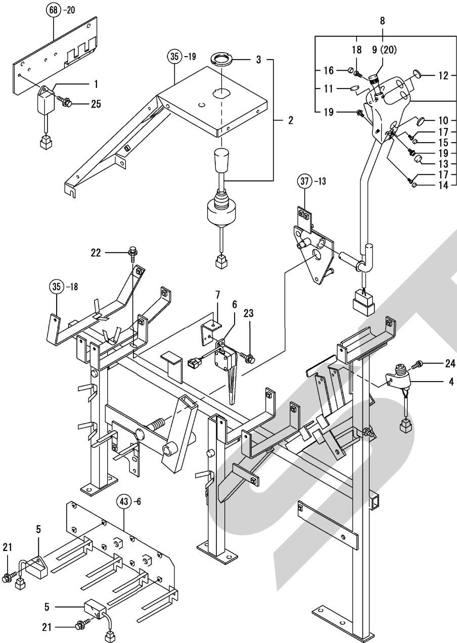
Fig. 69. 作業制御
