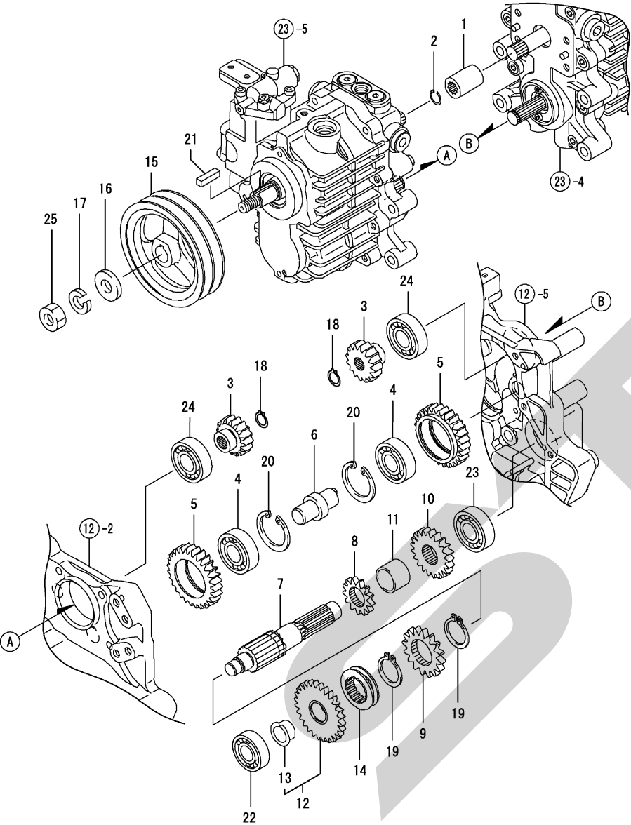
Fig.15. 入力軸
