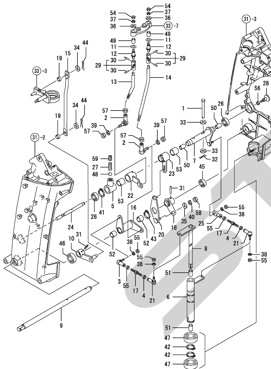
Fig. 34. ステアリング操作 (2)
