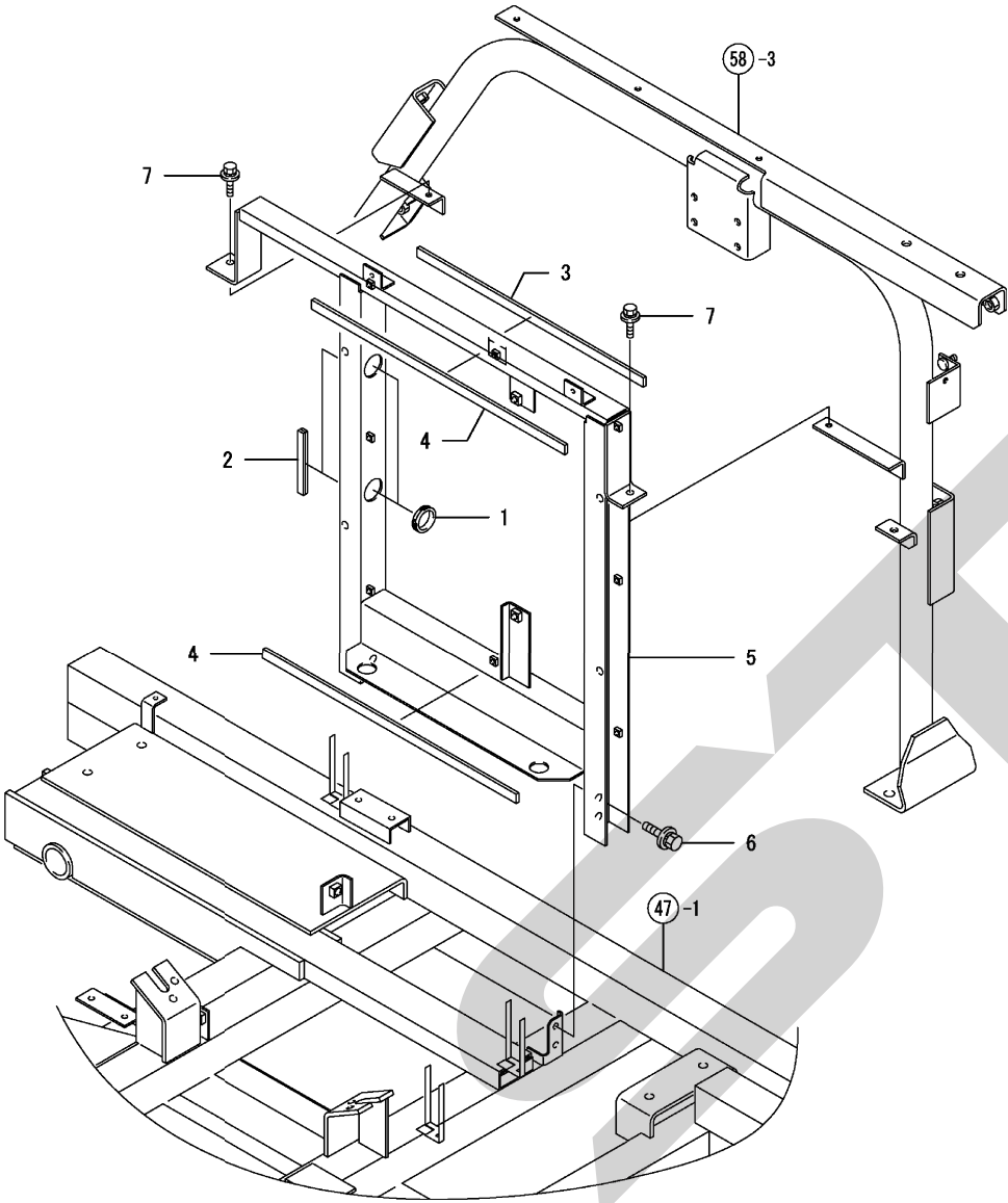
Fig. 59. エンジンルーム枠
