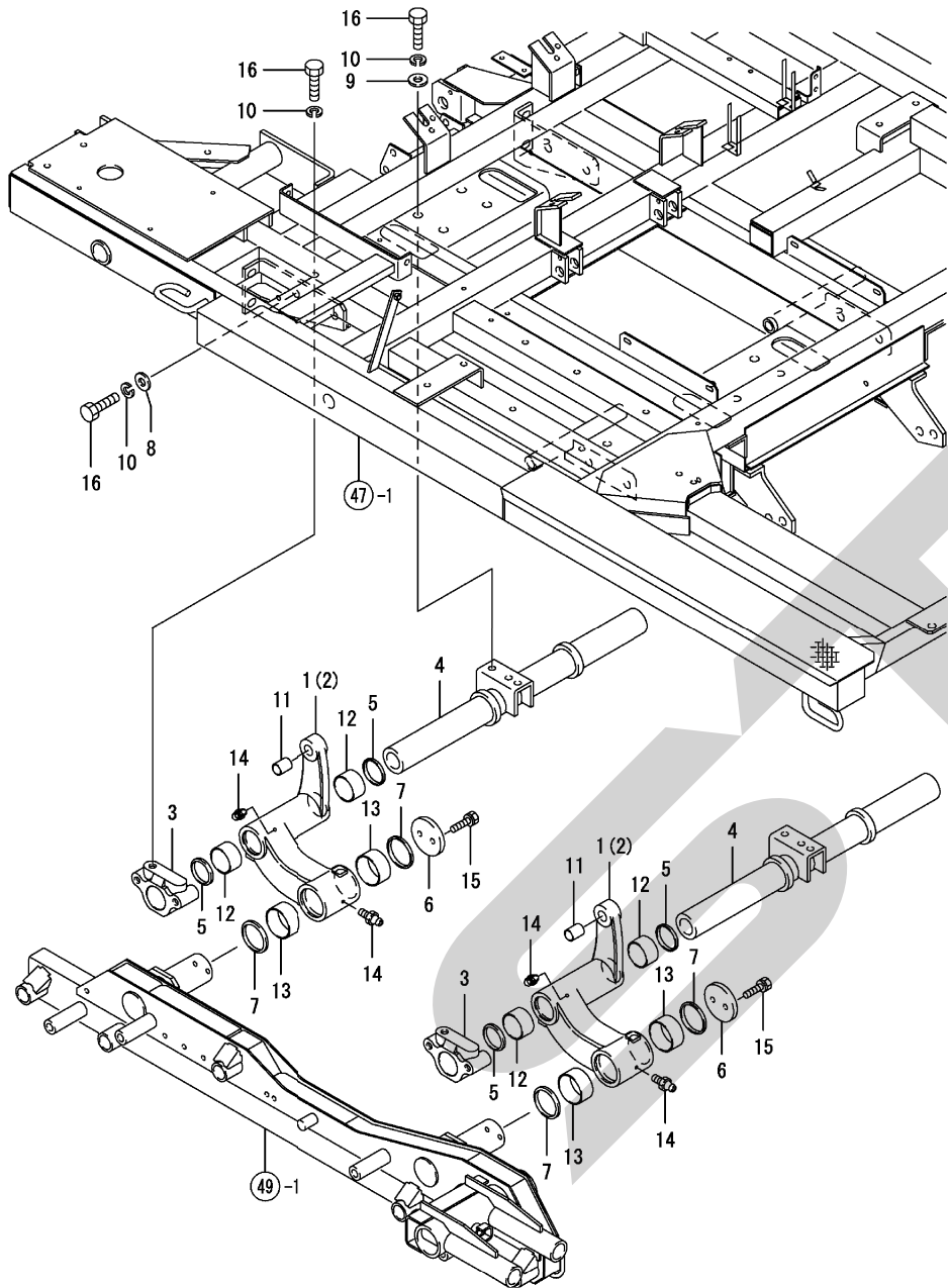
Fig. 56. スイング (1)
