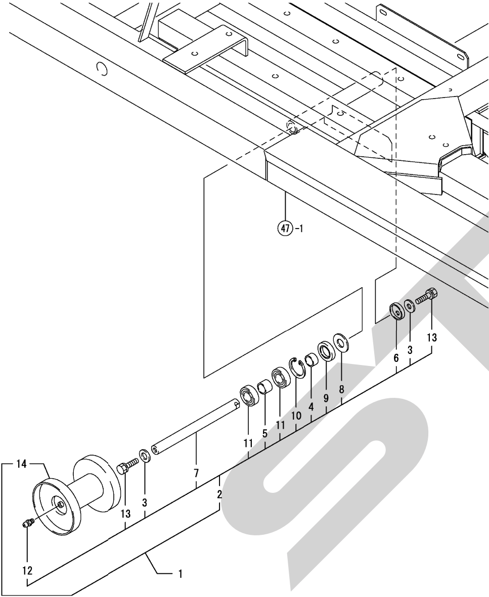
Fig. 54. キャリアローラ
