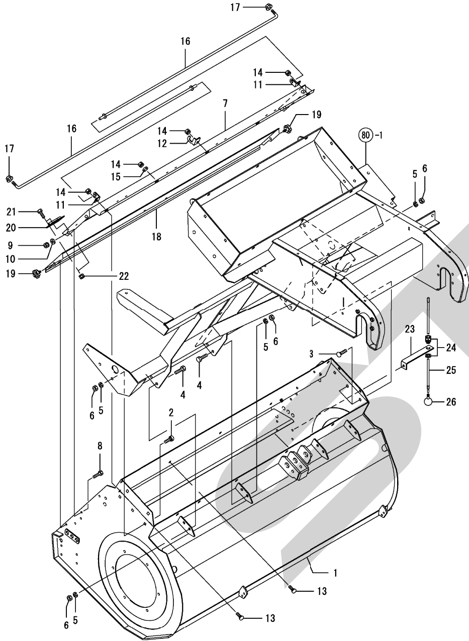
Fig. 85. ケーシング
