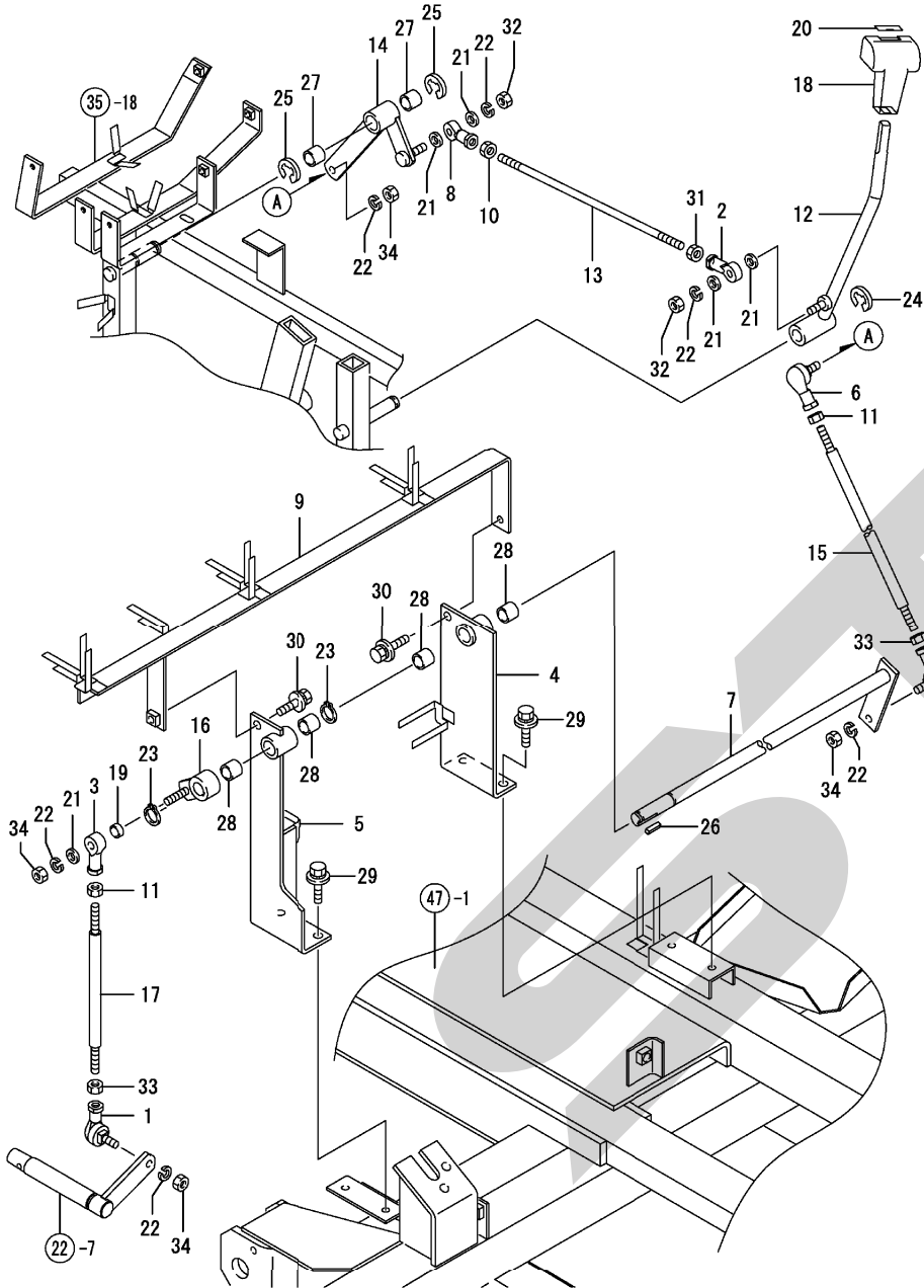
Fig. 38. 副変速操作
