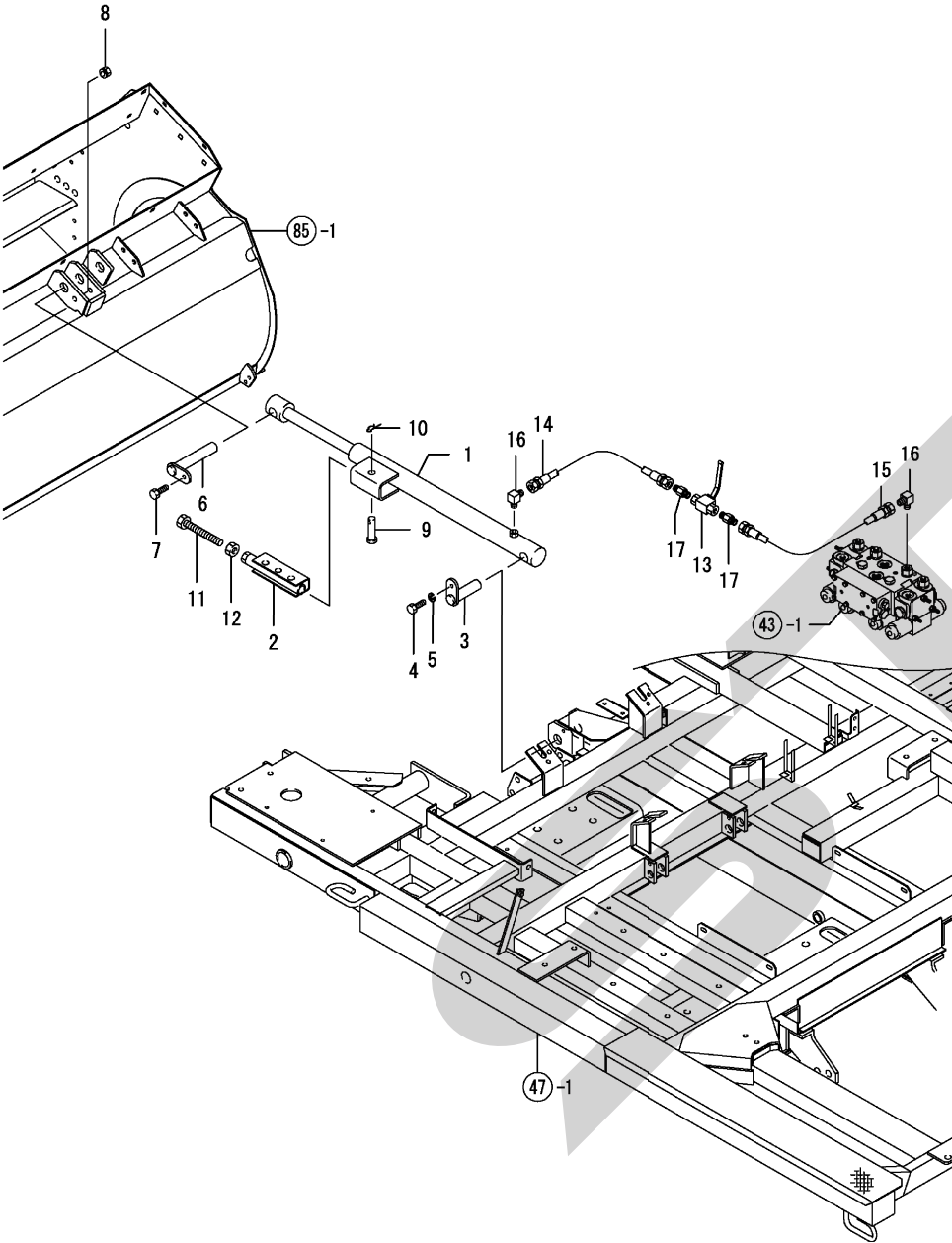
Fig.107. 油圧（フレール）
