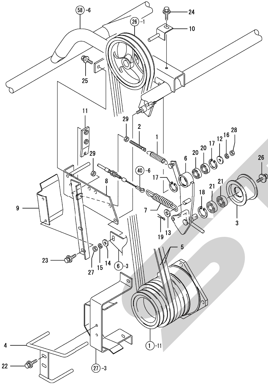
Fig. 25. フレールベルト
