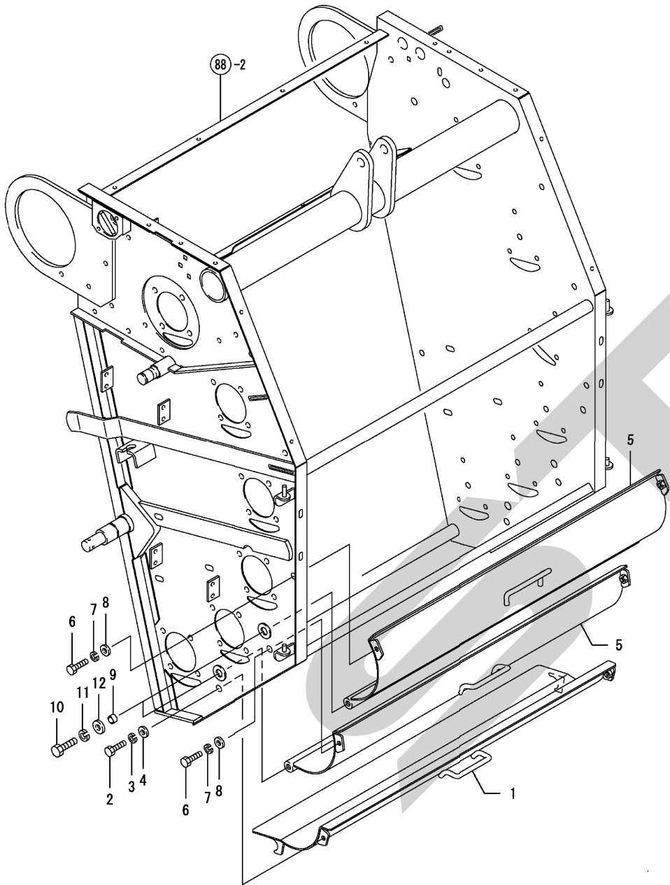
Fig. 106. ローラカバー
