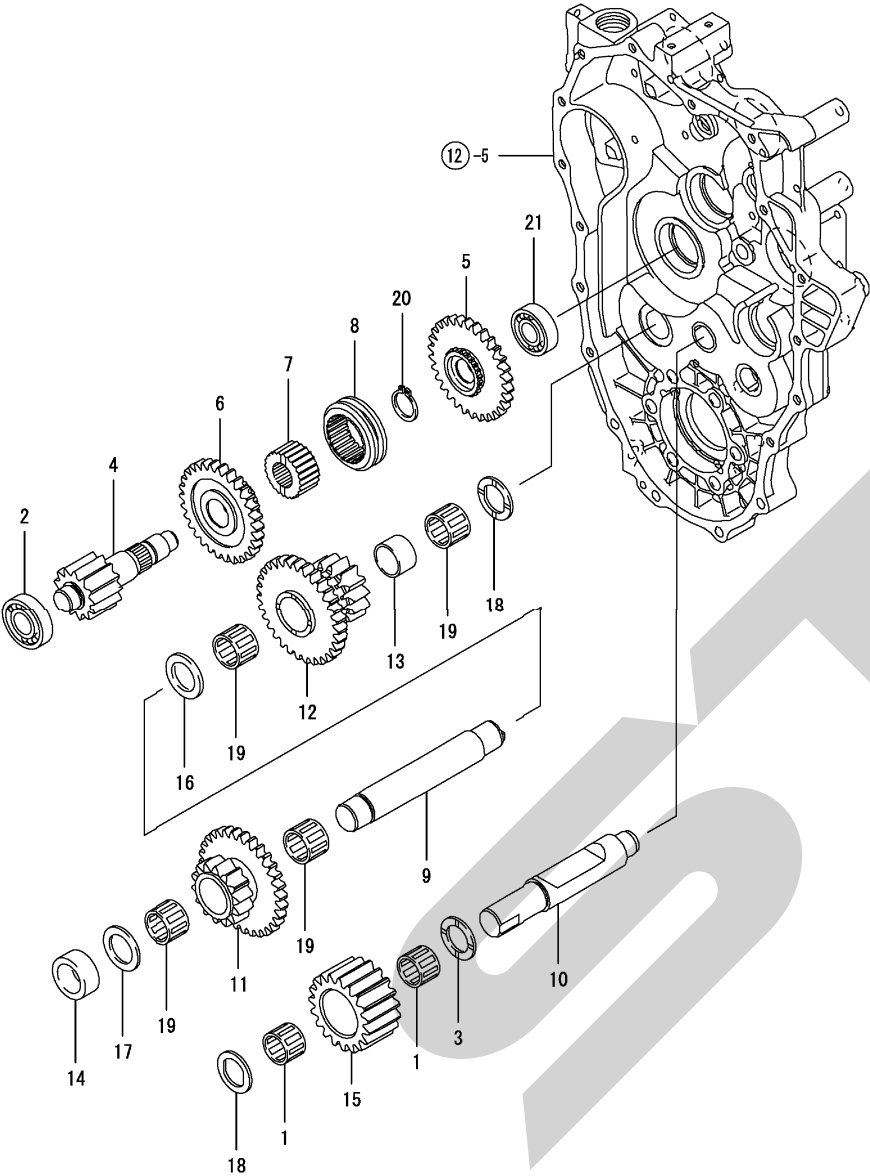
Fig. 19. Sカウンタシャフト
