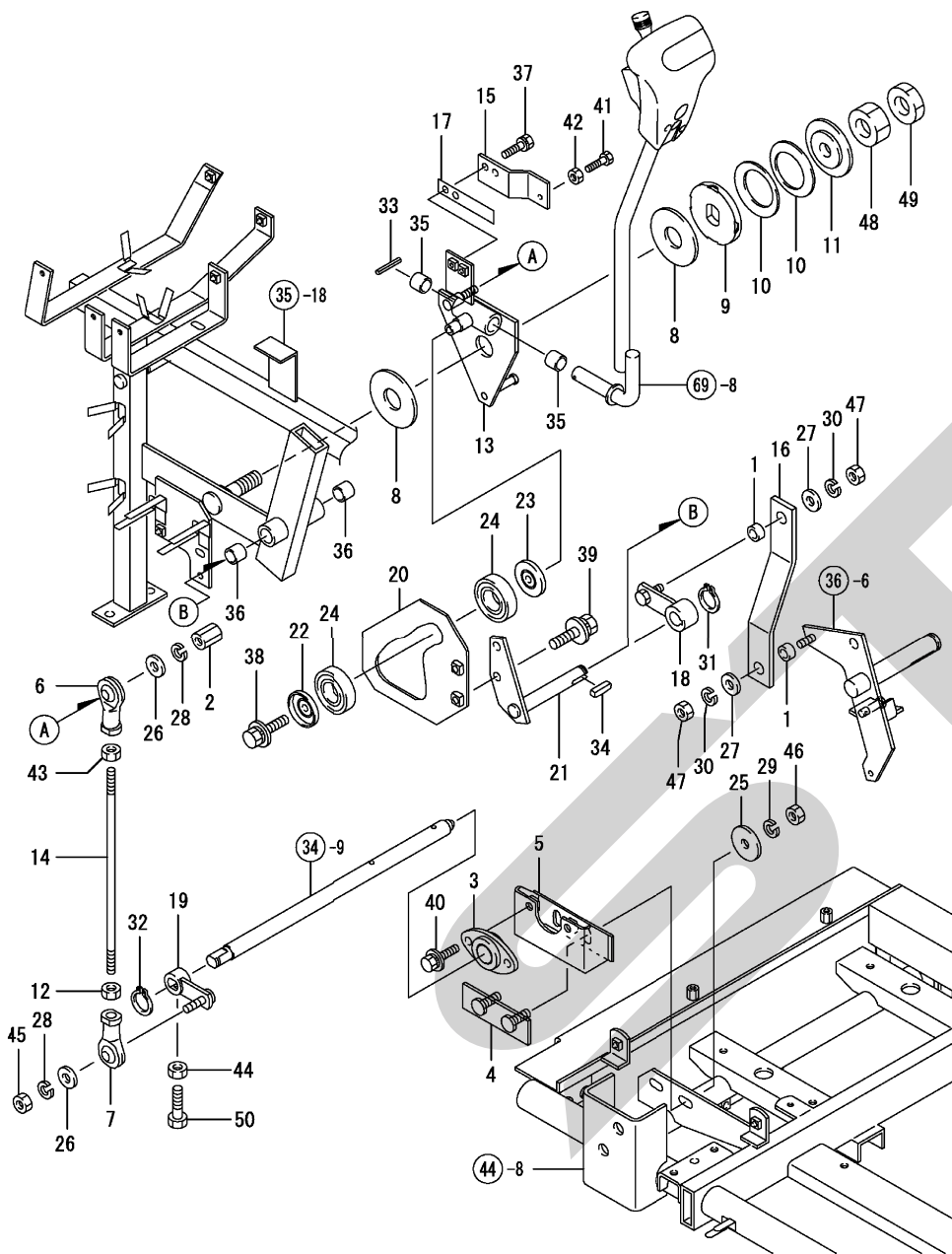
Fig. 37. 主変速操作
