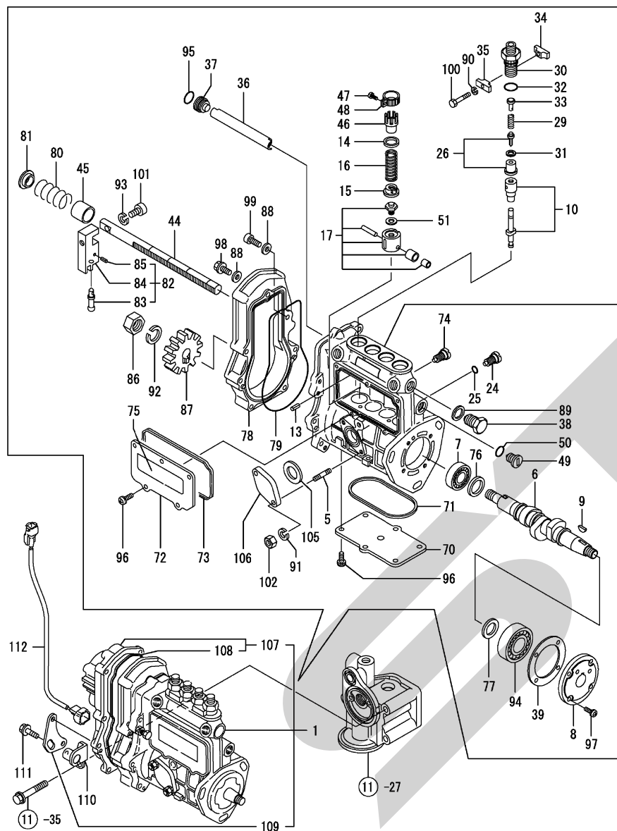
Fig. 14. F O 噴射ポンプ
