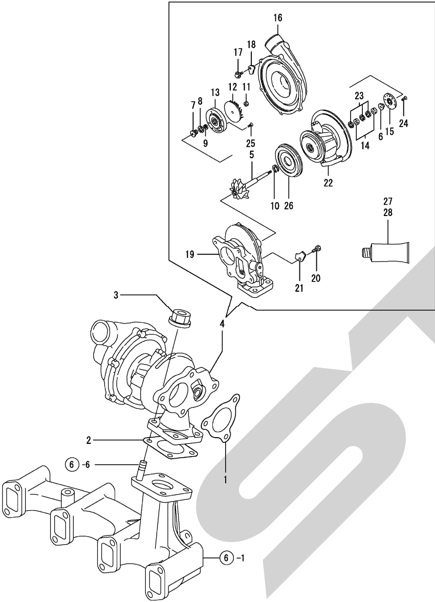
NPC-4028 Fig. 8. タービン
