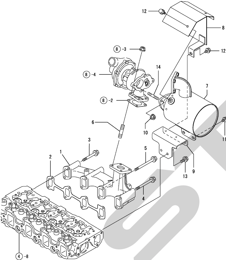
Fig. 6. 排気マニホールド & サイレンサ
