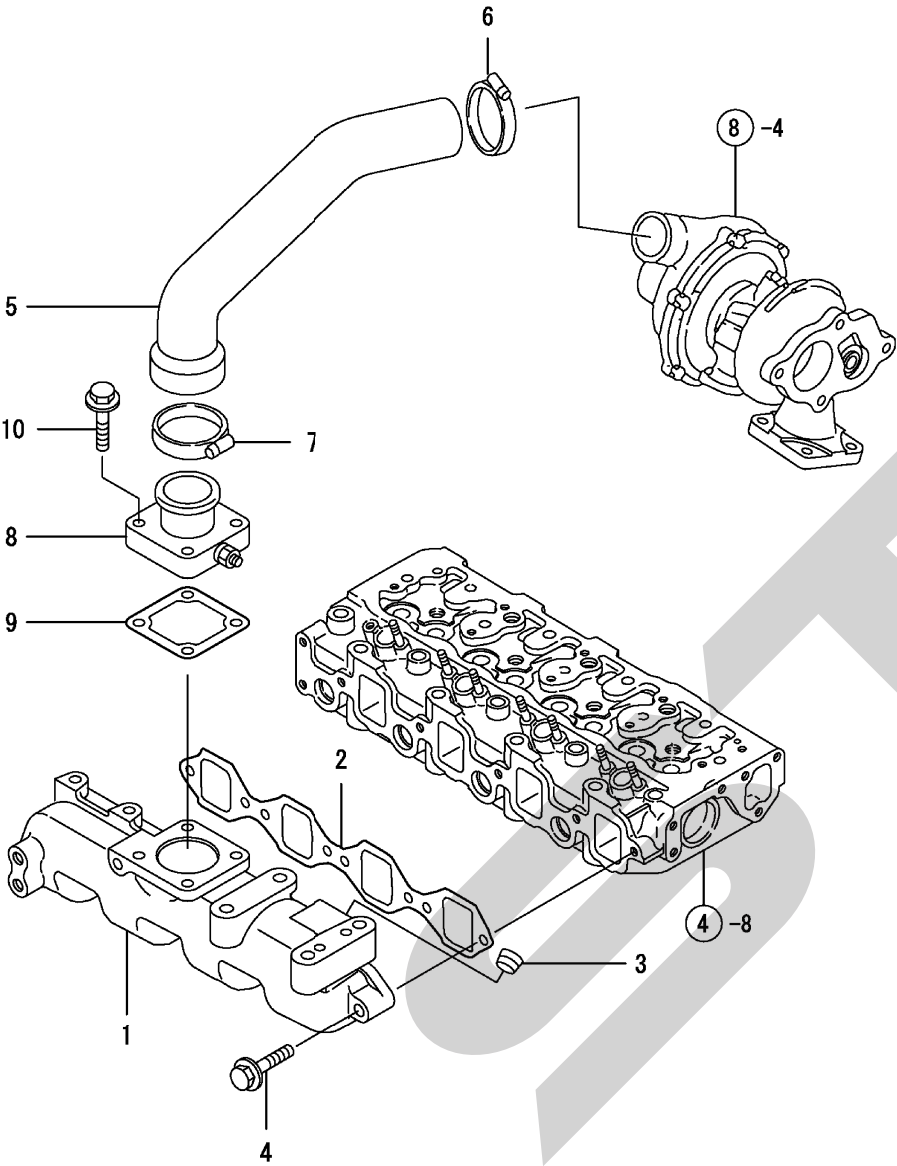
Fig. 5. 吸気マニホールド
