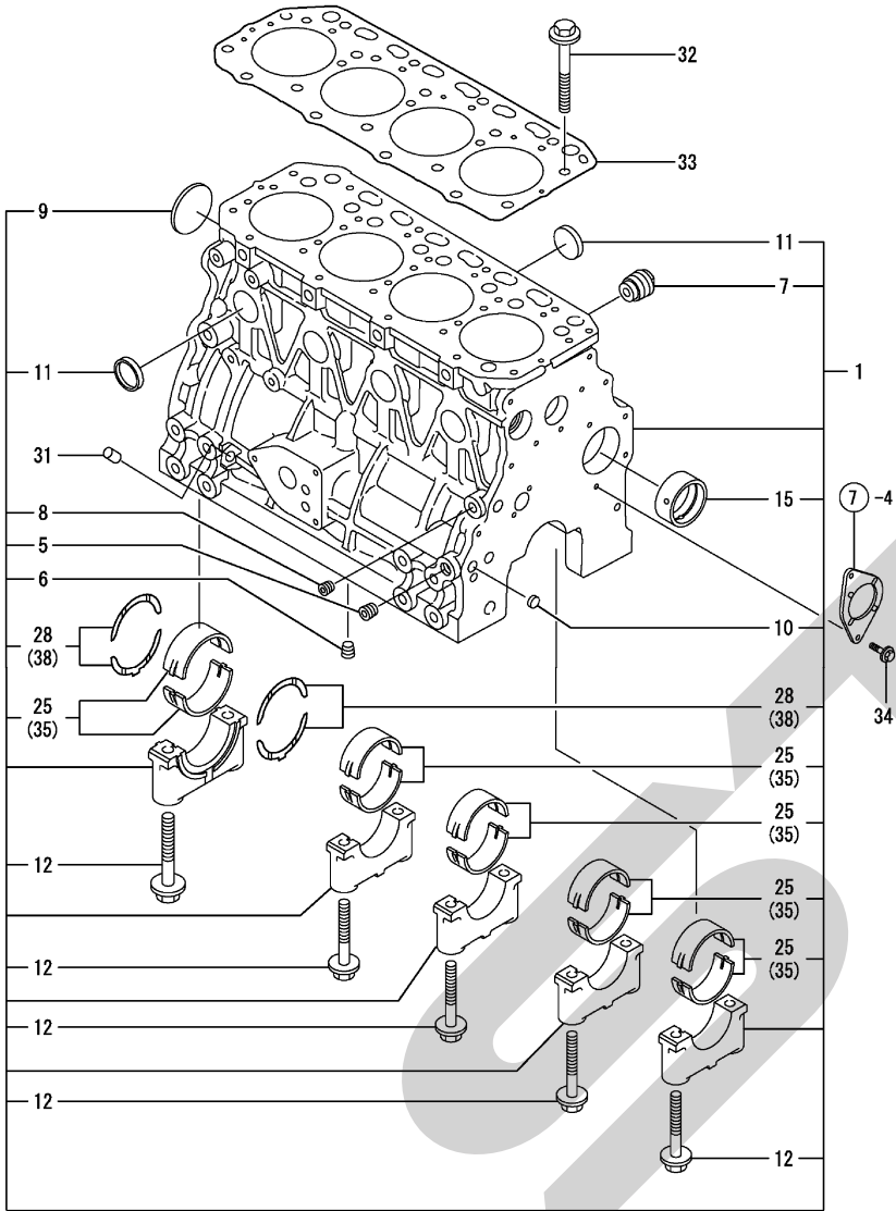
Fig.1. シリンダブロック
