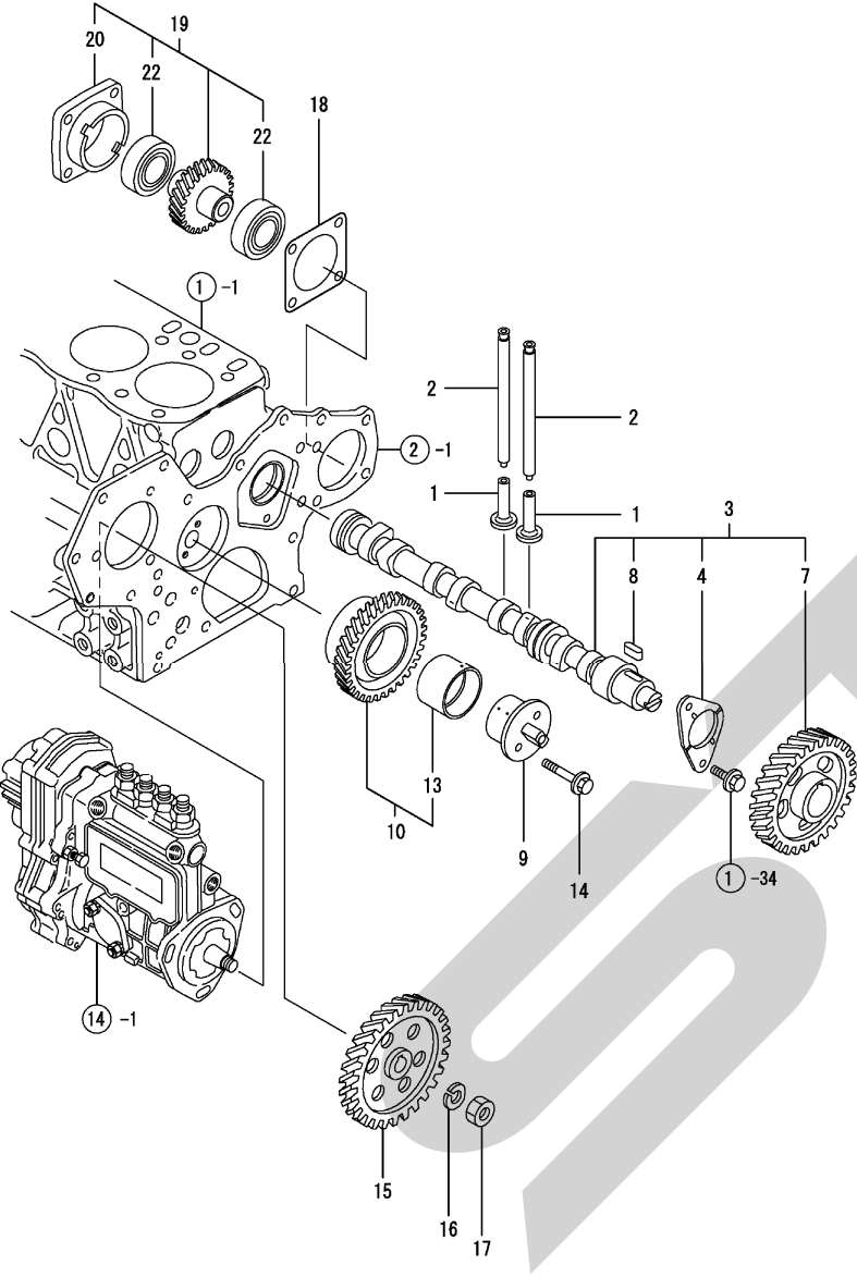
Fig.7. カムシャフト & 駆動ギヤ
