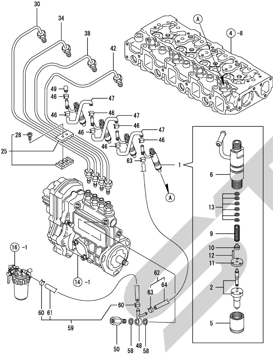
Fig. 15. F O 噴射弁
