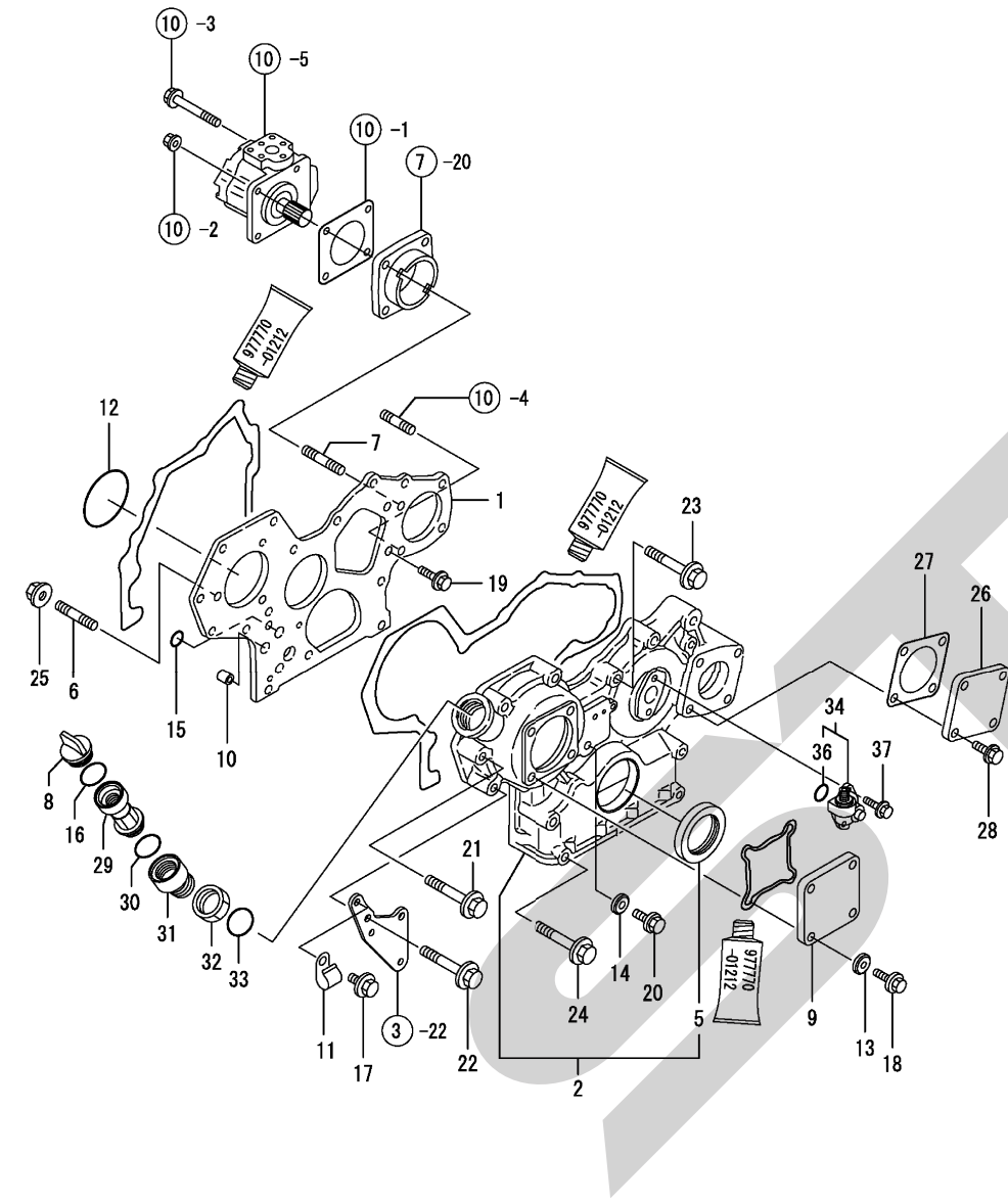
Fig. 2. ギヤケース
