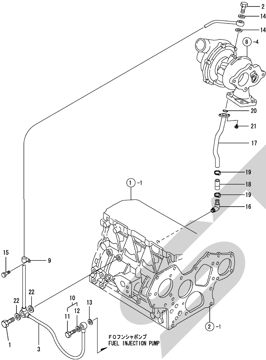
Fig. 12. L Oパイプ
