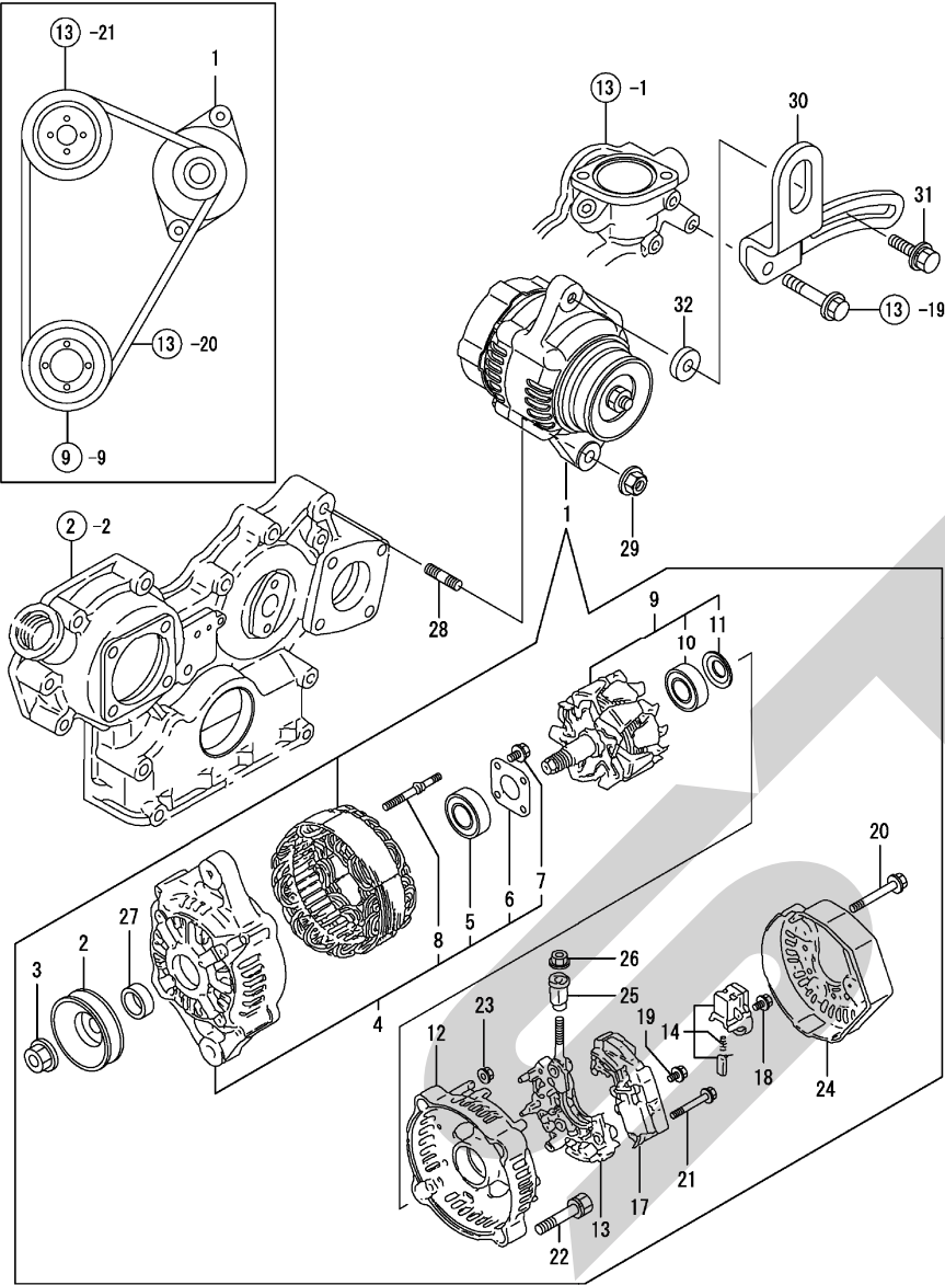
Fig. 18. ジェネレータ
