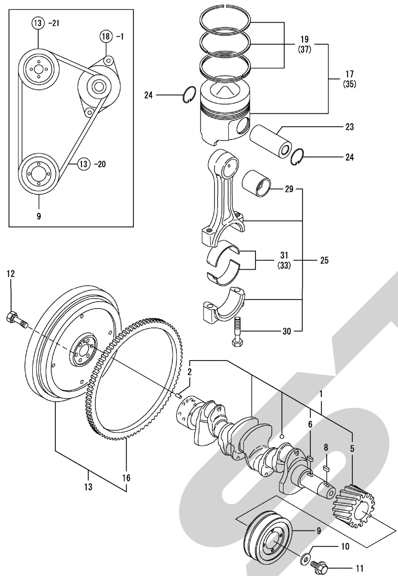
Fig. 9. クランクシャフト & ピストン
