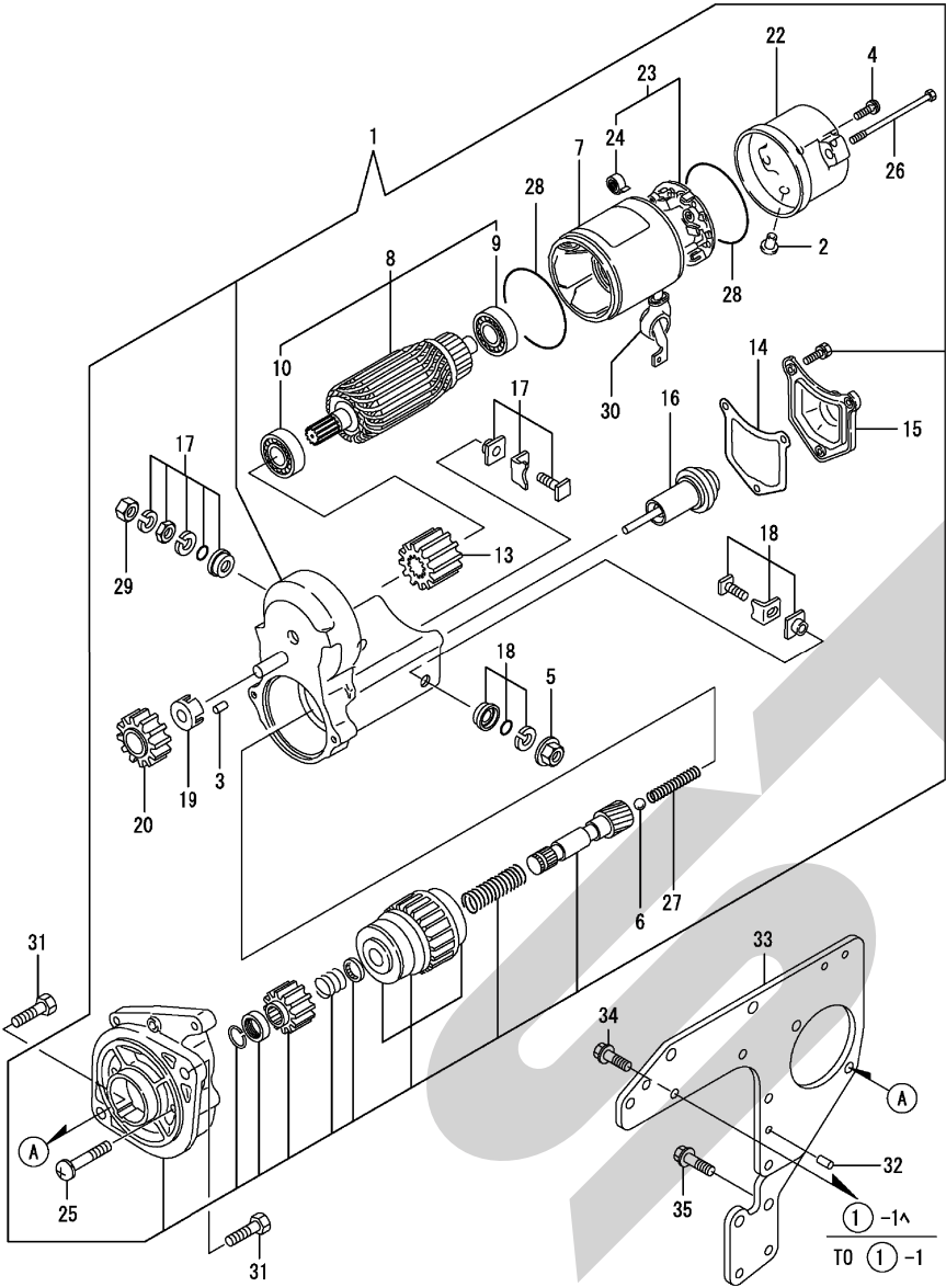
Fig. 17. スターティングモータ
