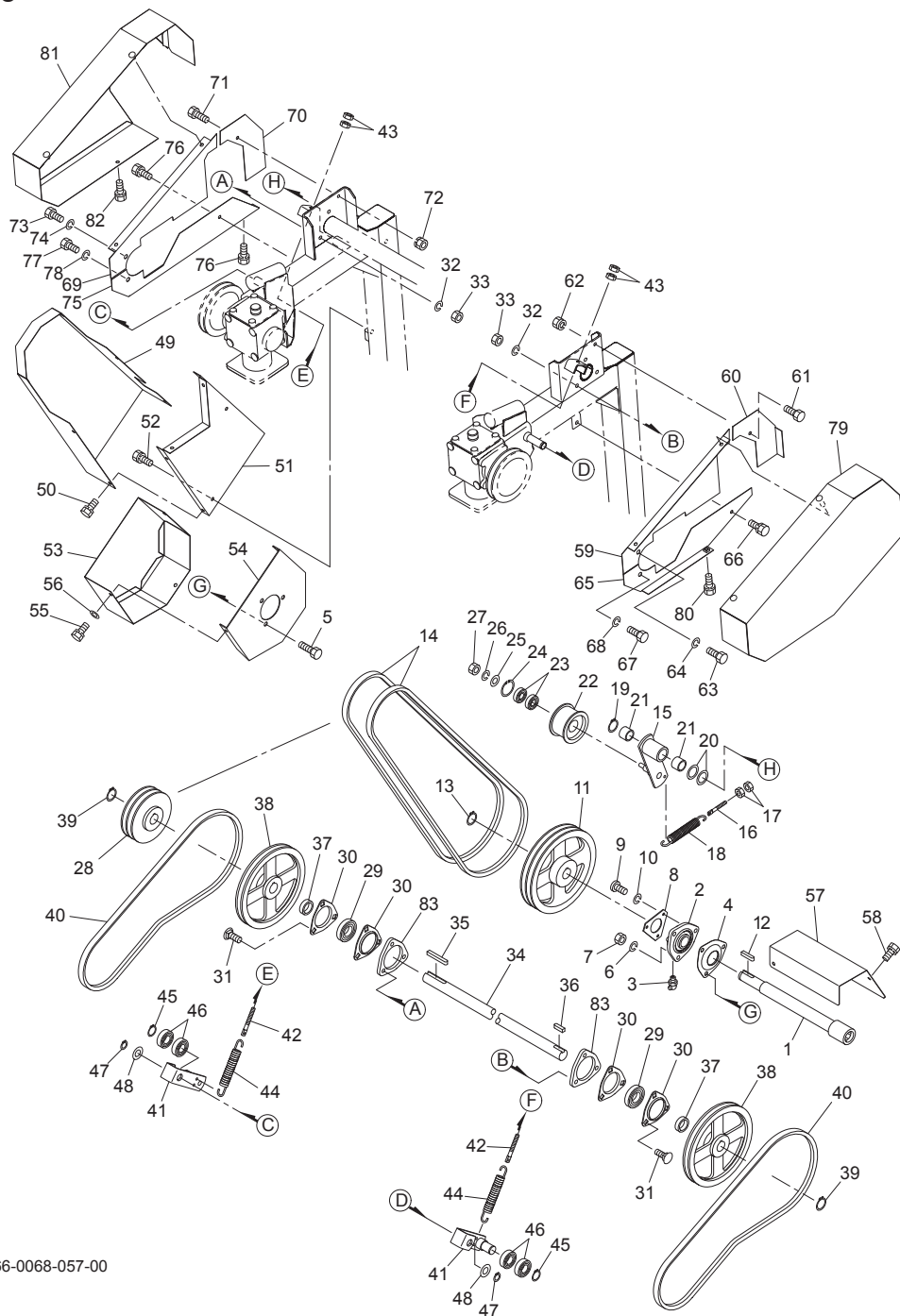
Fig.513. 駆動;ドラム
