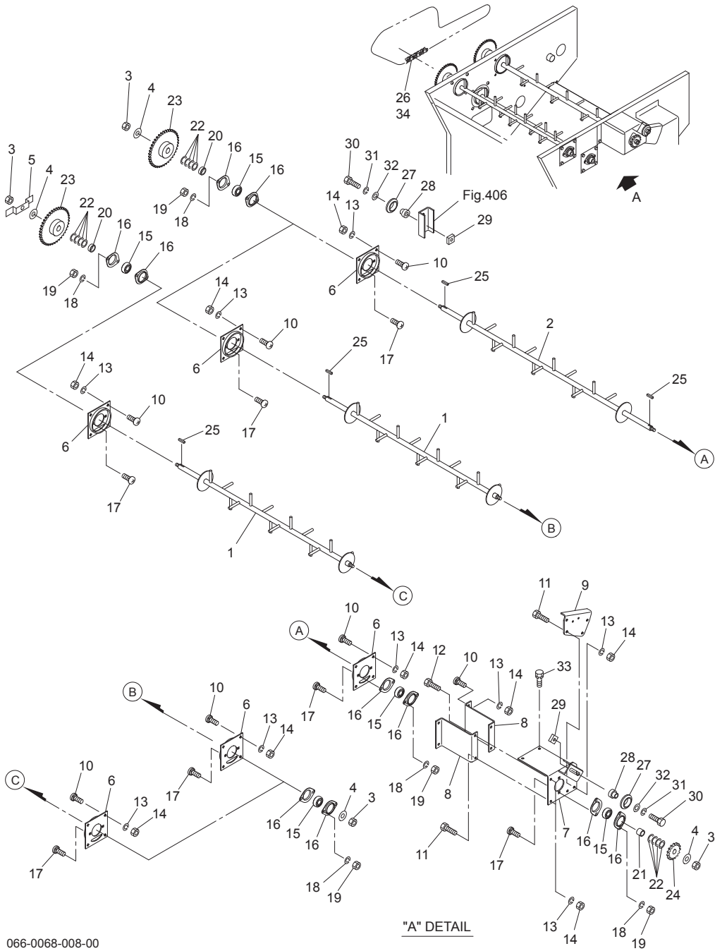
Fig.408. アジテータ
