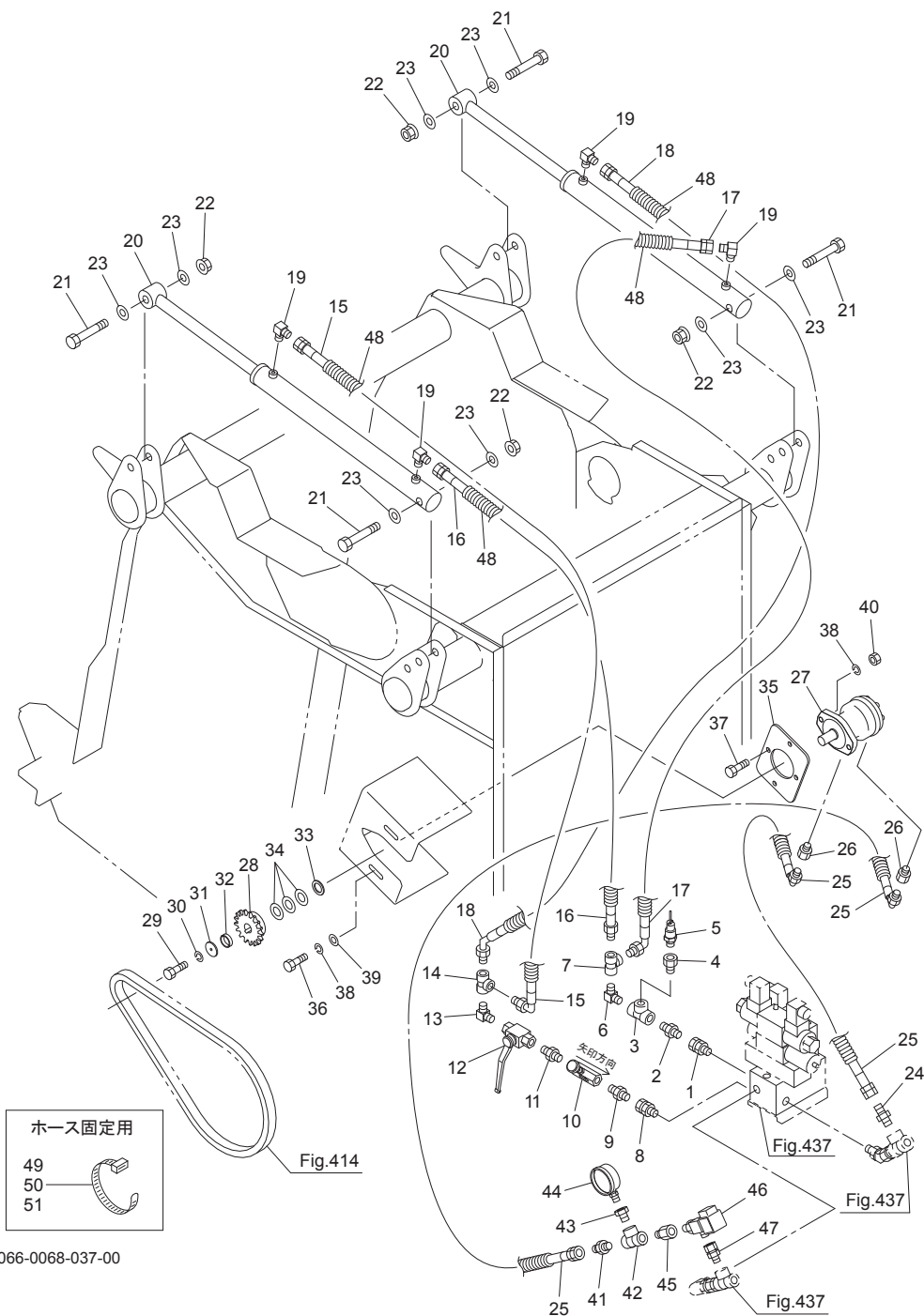
Fig.438. 油圧(ゲート)
