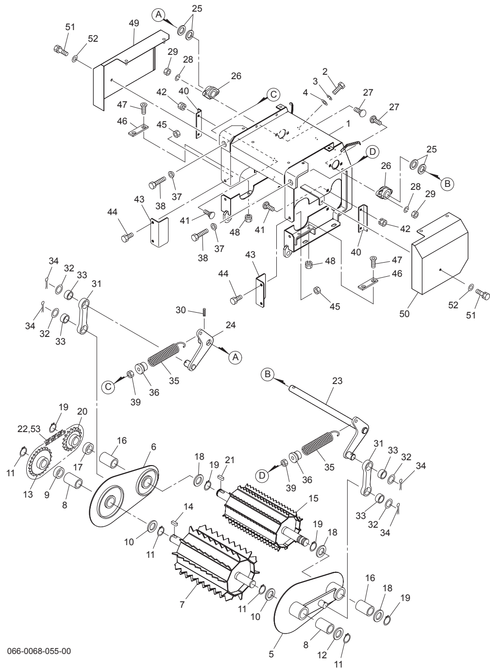
Fig.511. ロール; U
