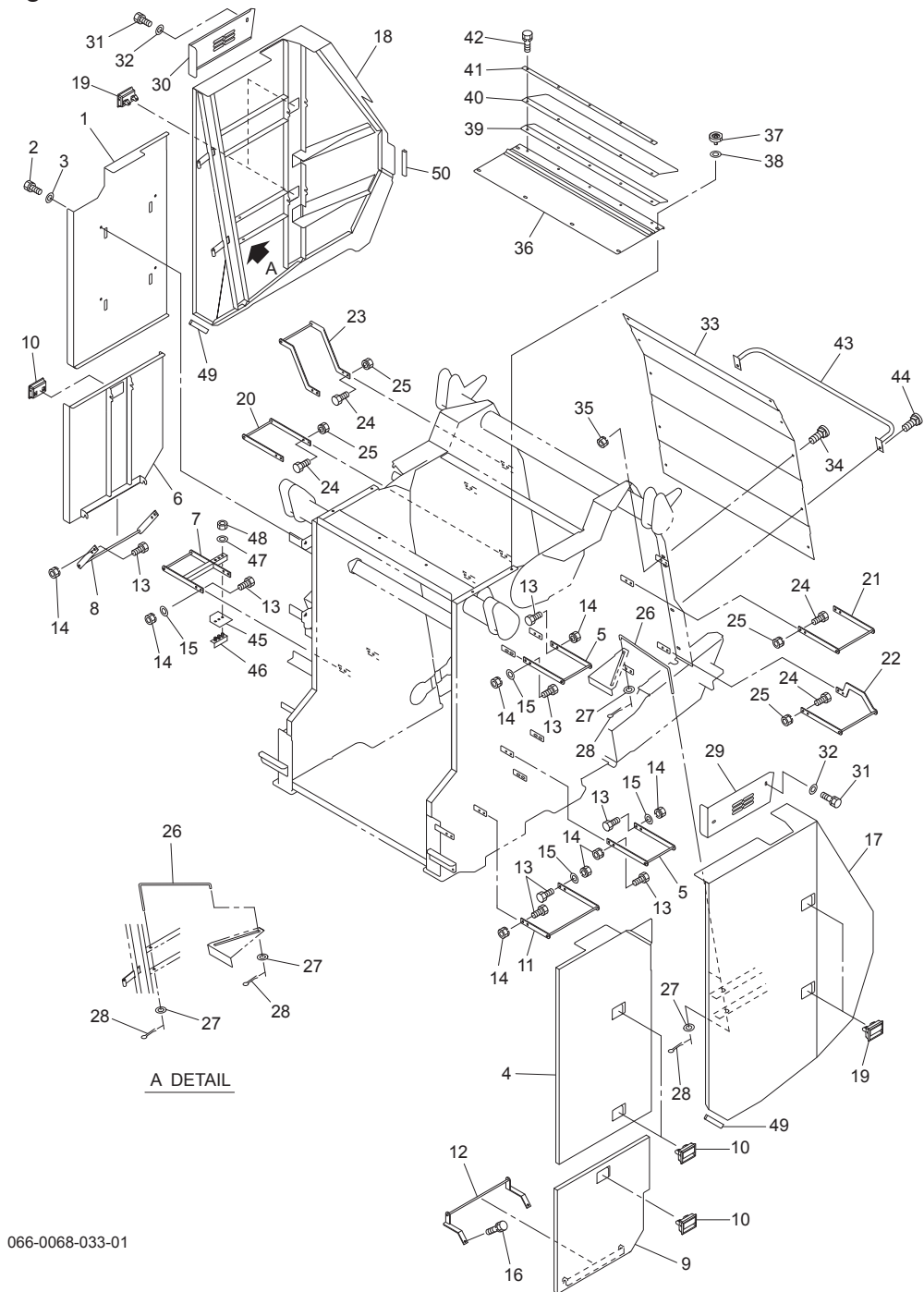
Fig.433. カバー(2)
