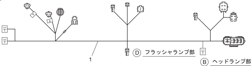
Fig.442. 電装(4)
