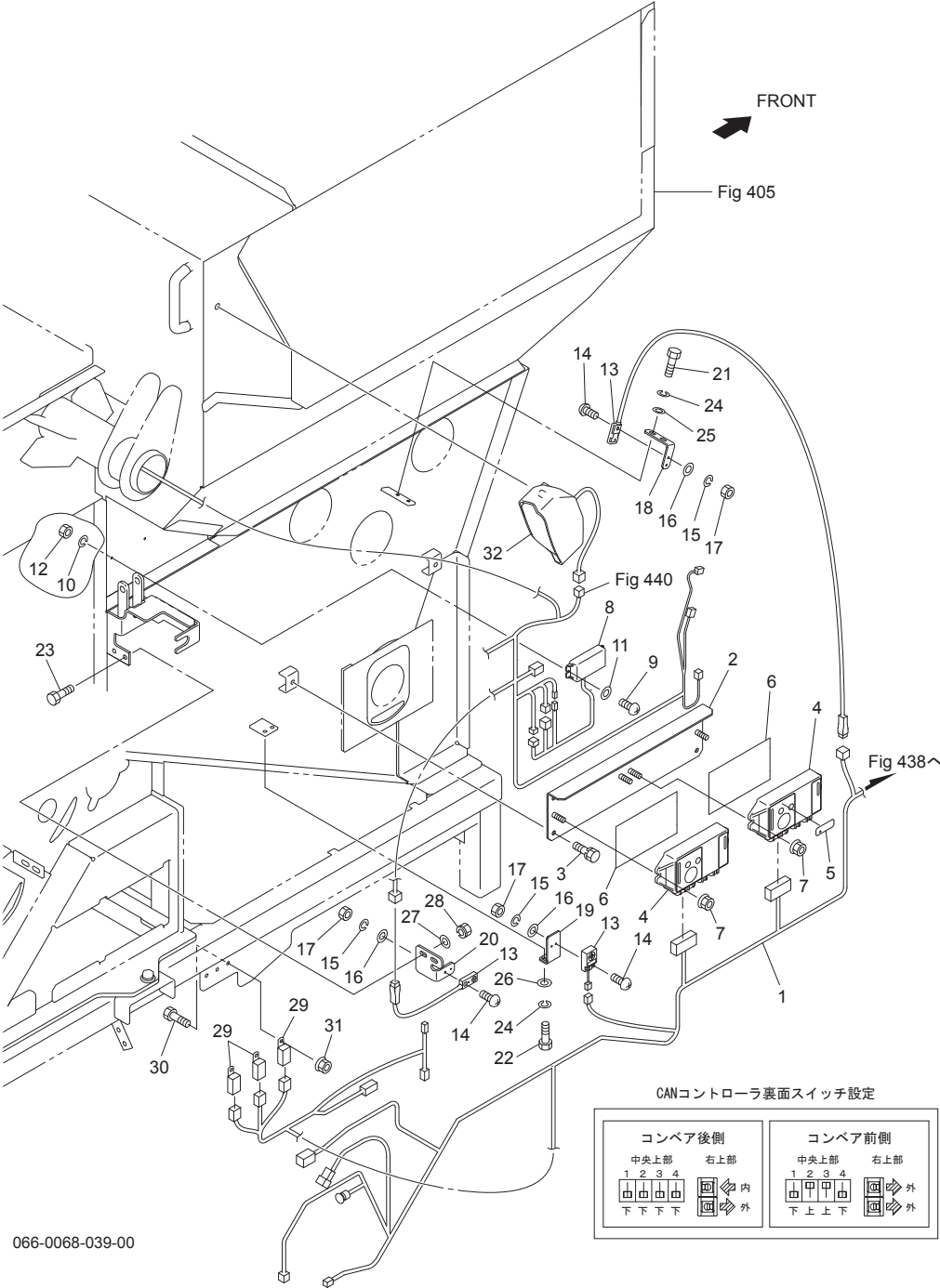
Fig.440. 電装(2)
