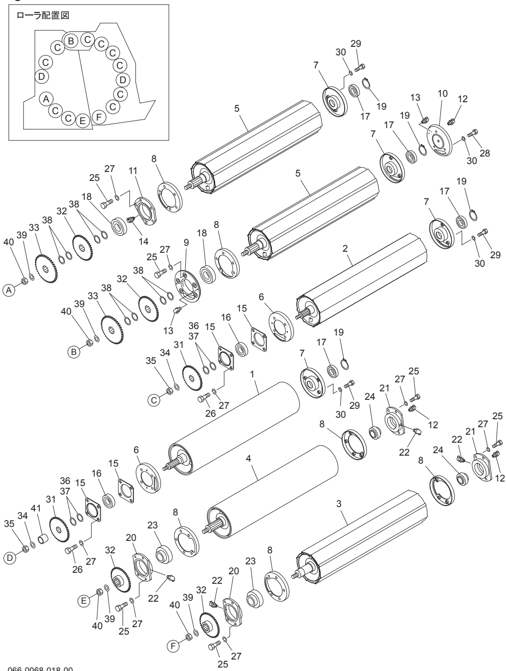
Fig.418. ローラ
