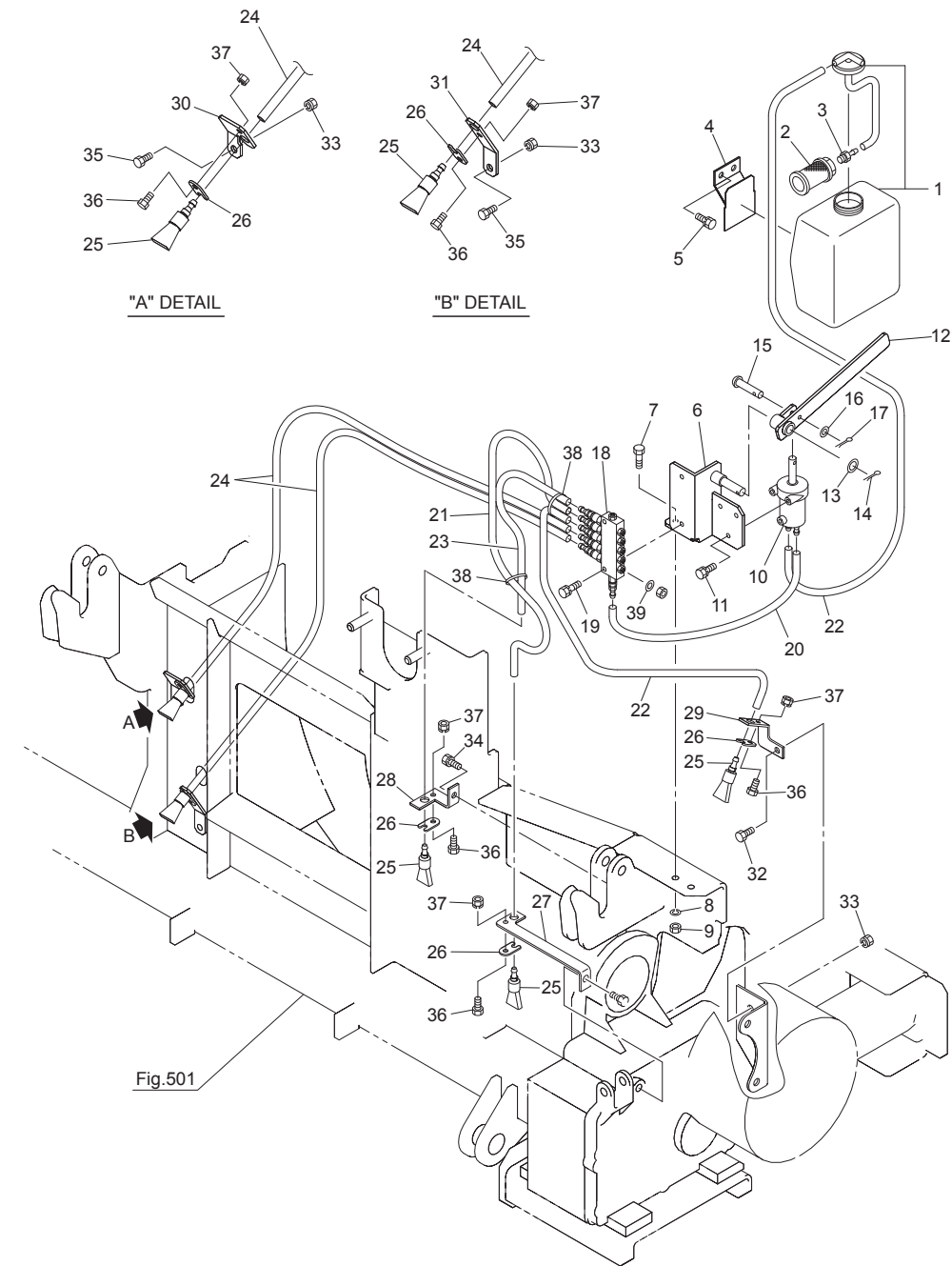
Fig.520. 給油
