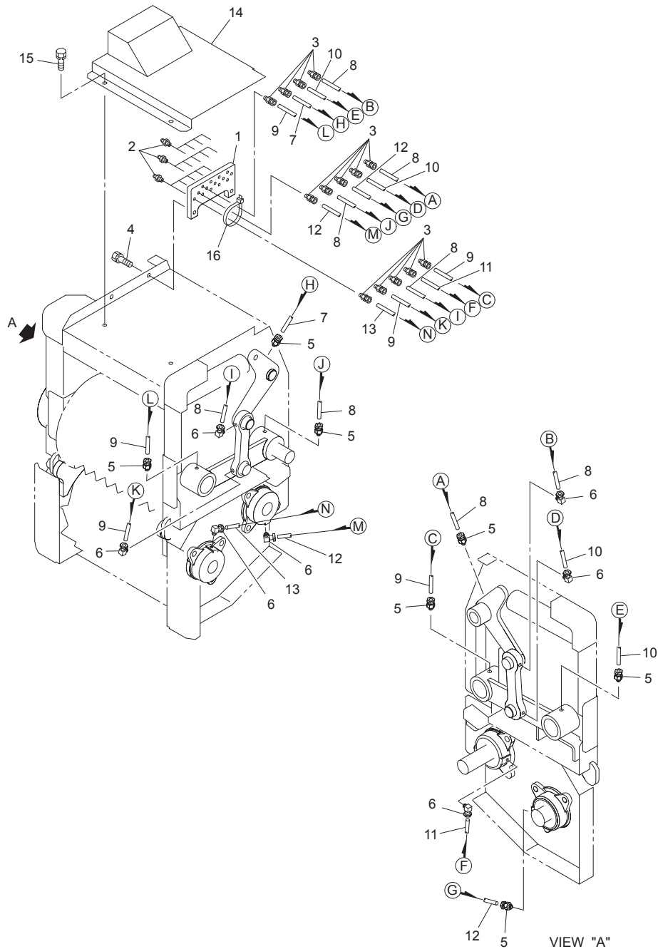
Fig.521. 給脂
