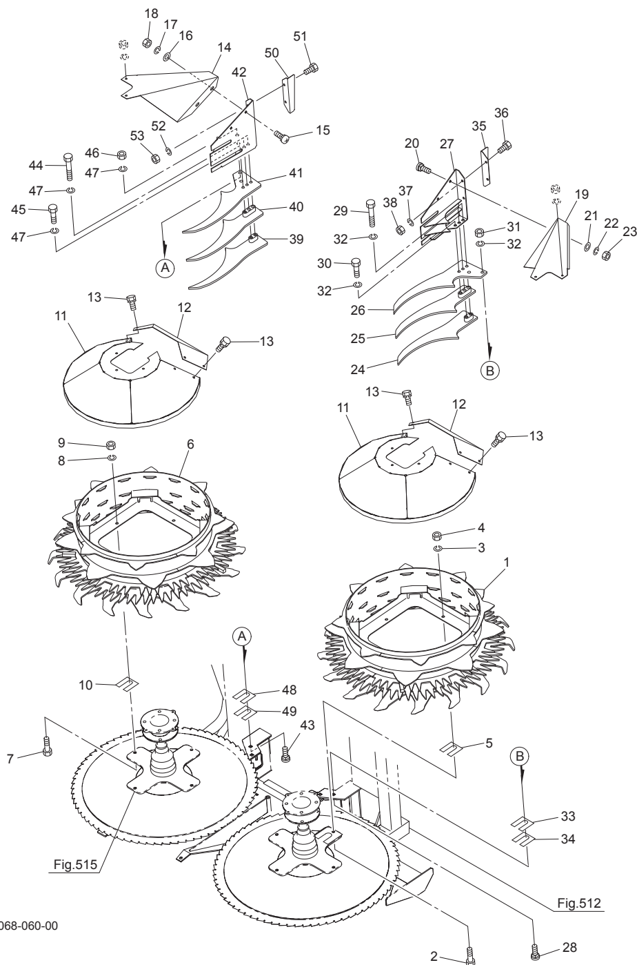
Fig.516. ドラム
