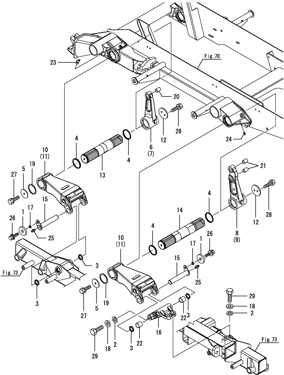
OCNP6-M03520 走行部(3) Fig.81. スイング(1)
