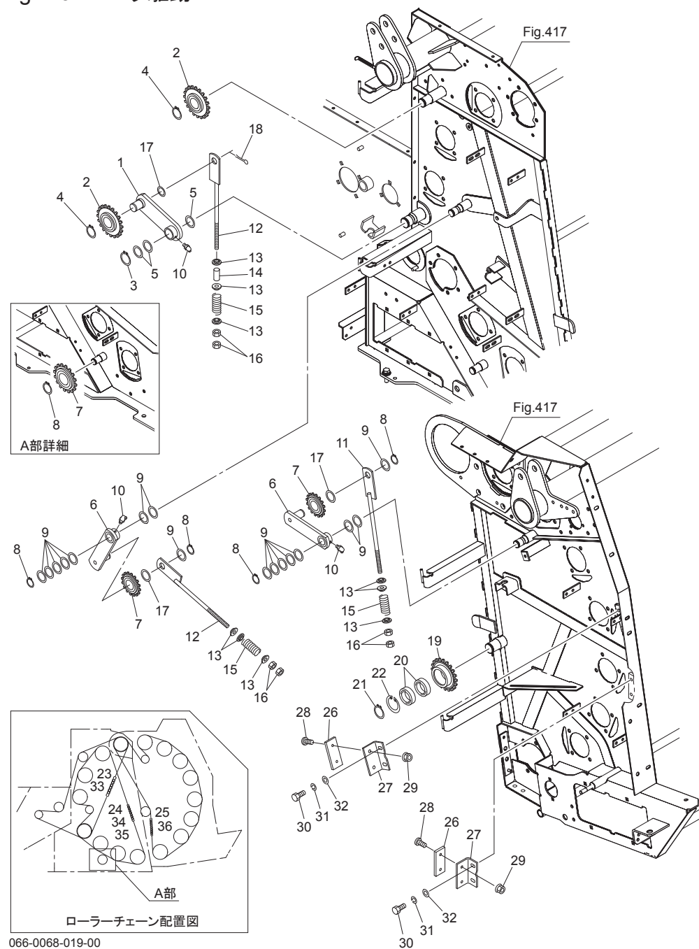
Fig.419. ローラ駆動
