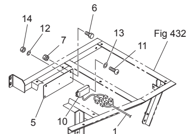
(C) モータコントロールユニット部
