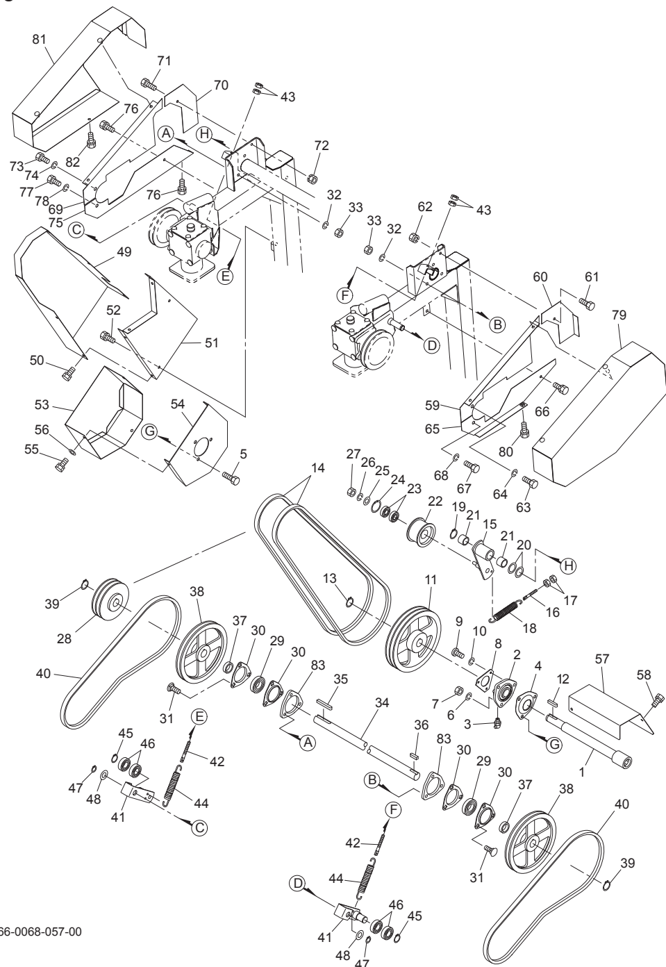
Fig.513. 駆動;ドラム
