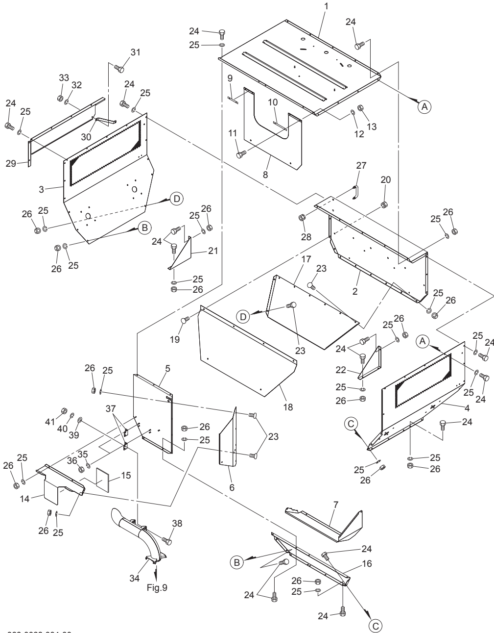
Fig.404. ホッパ
