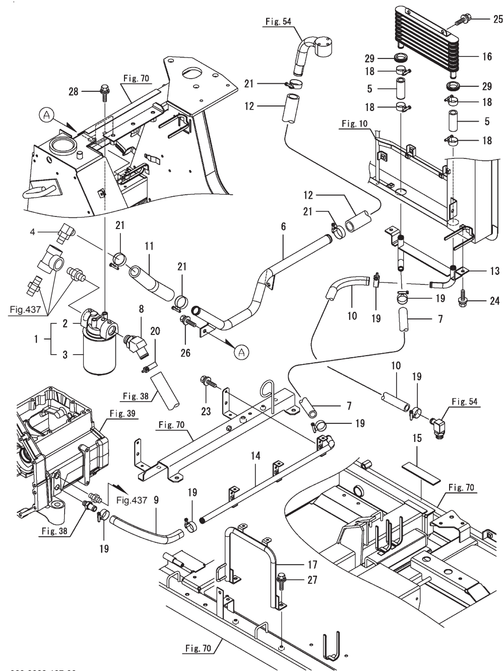
Fig.58. 配管(2)
