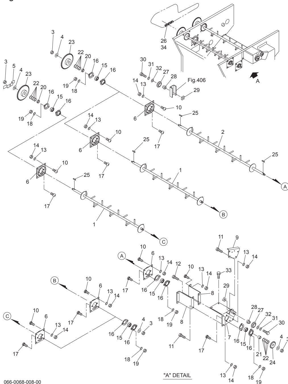
Fig.408. アジテータ
