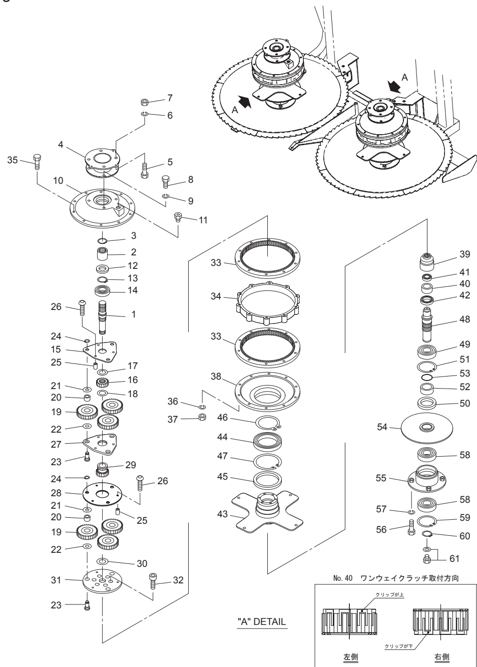
Fig.515. ユウセイボックス
