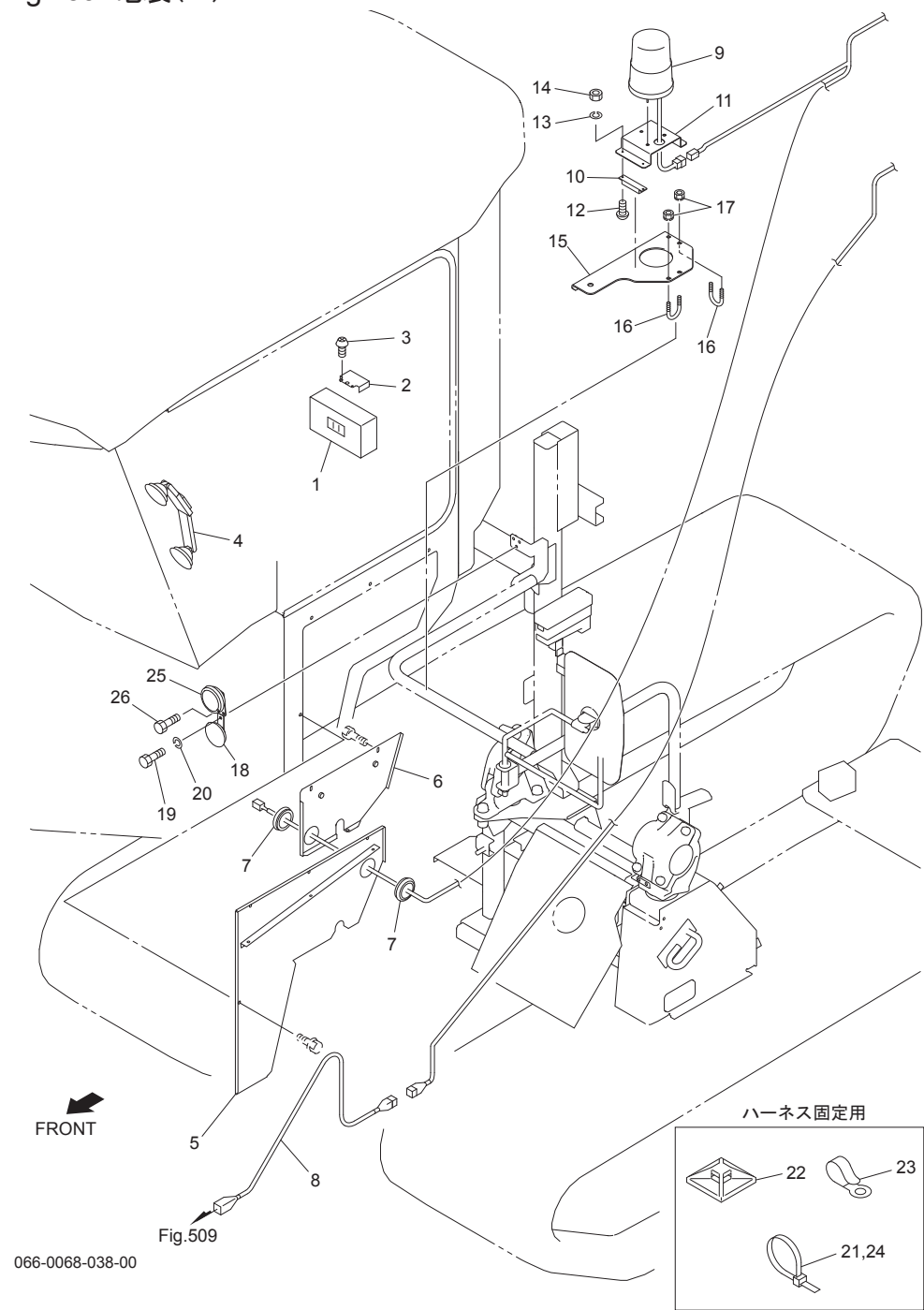
Fig.439. 電装(1)
