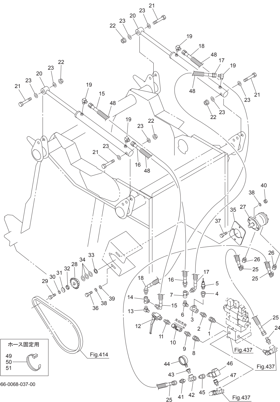
Fig.438. 油圧(ゲート)
