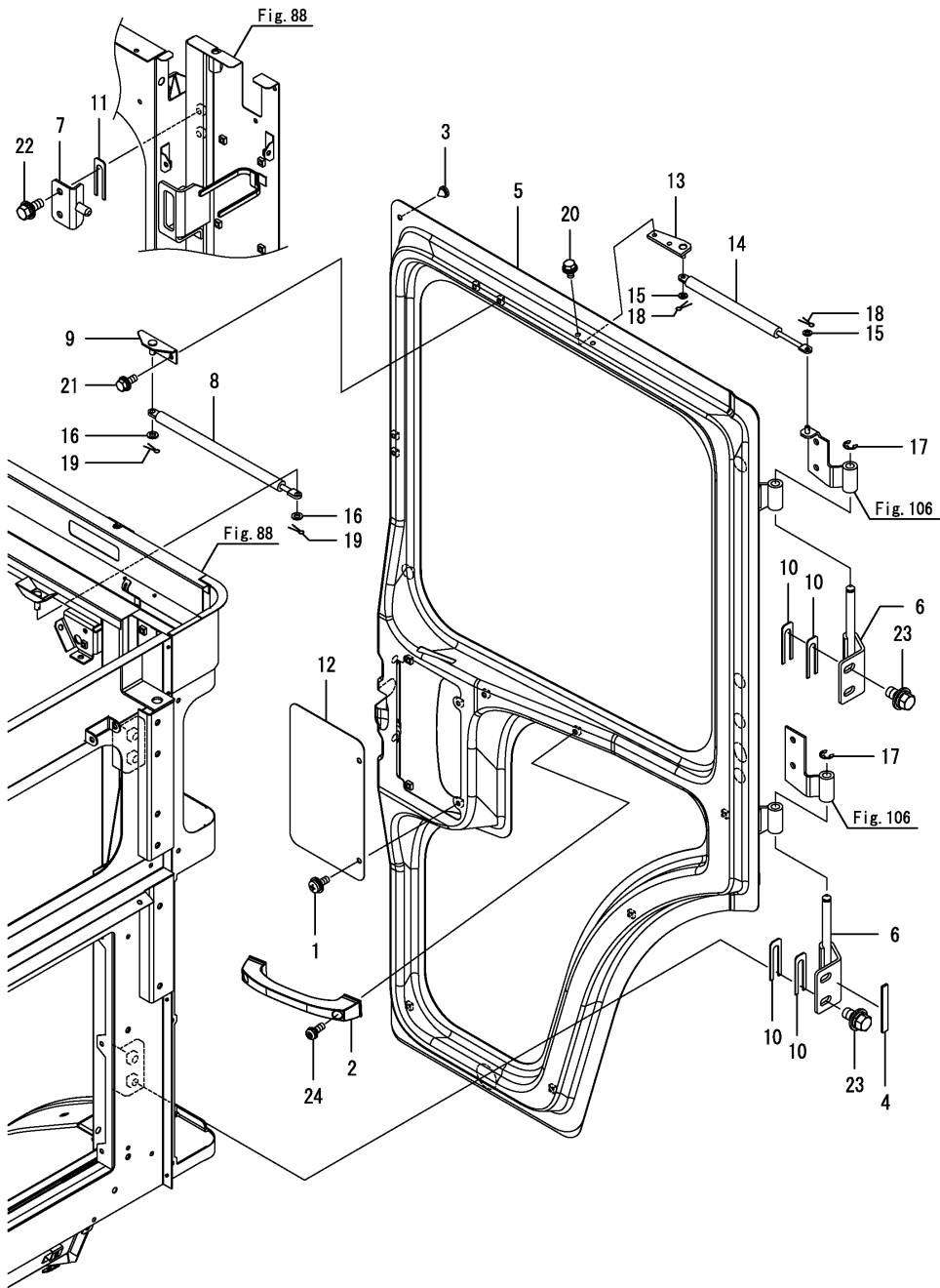
OCNP6-M03520 キャビン部 Fig.104. キャビンドア(1)
