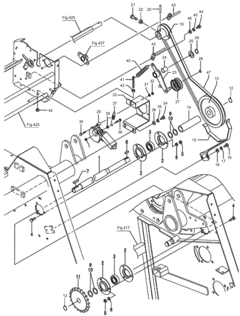
Fig.424. 駆動(ネット)
