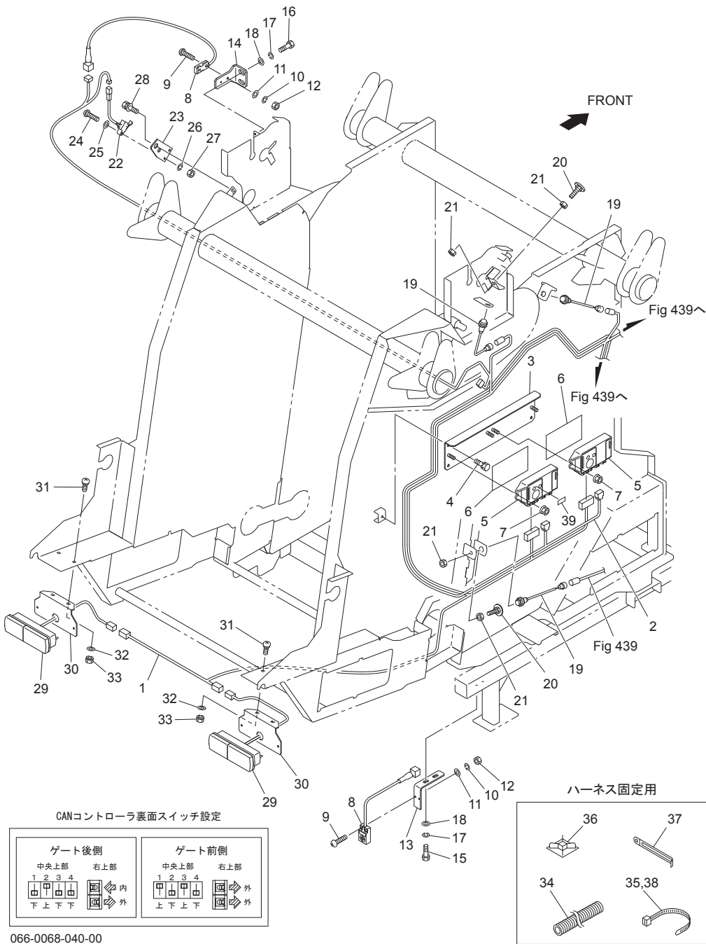
Fig.441. 電装(3)
