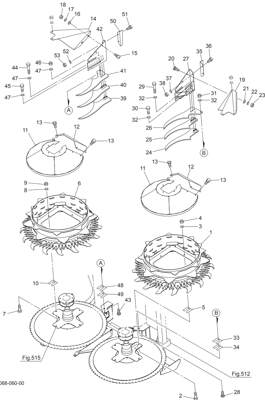
Fig.516. ドラム
