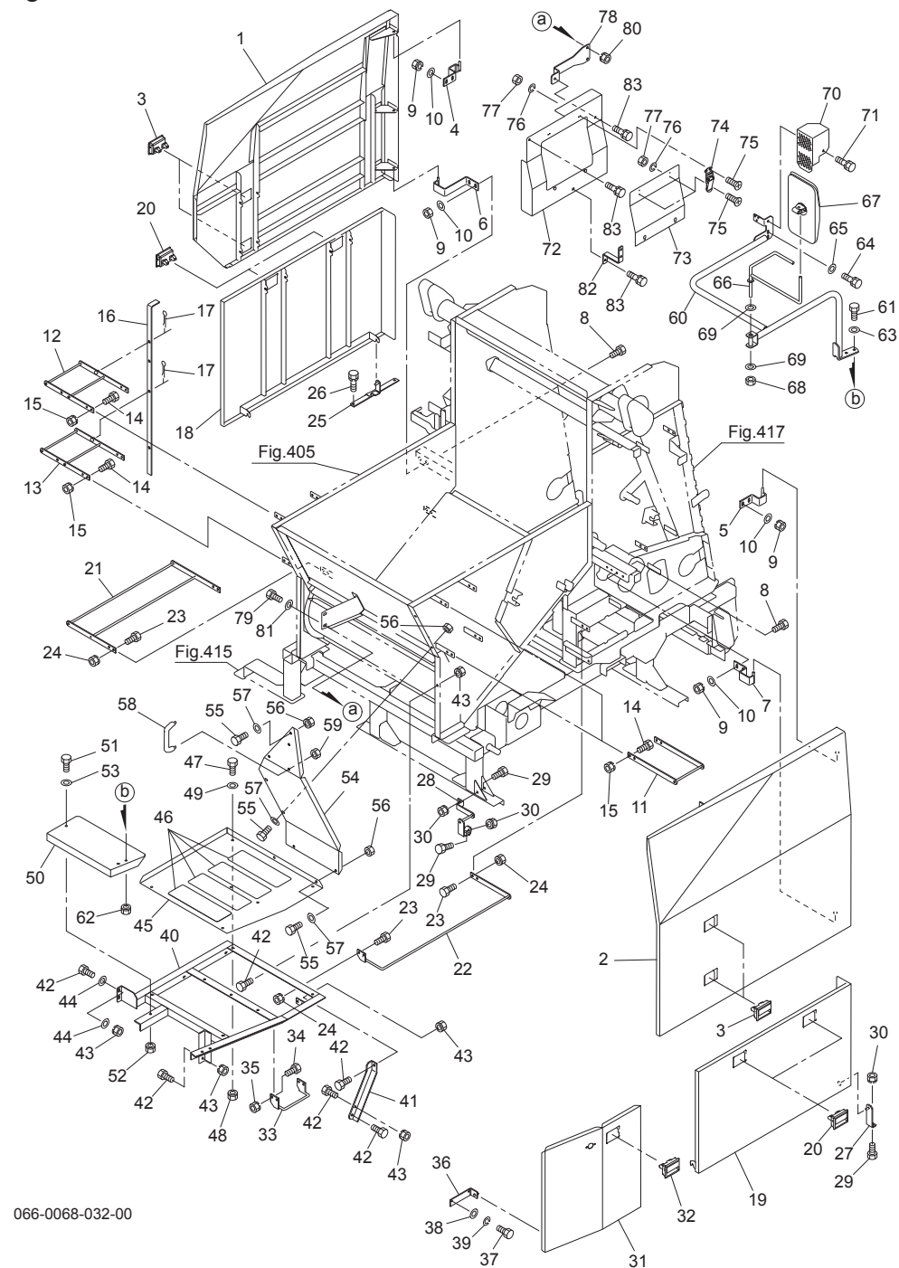
Fig.432. カバー(1)
