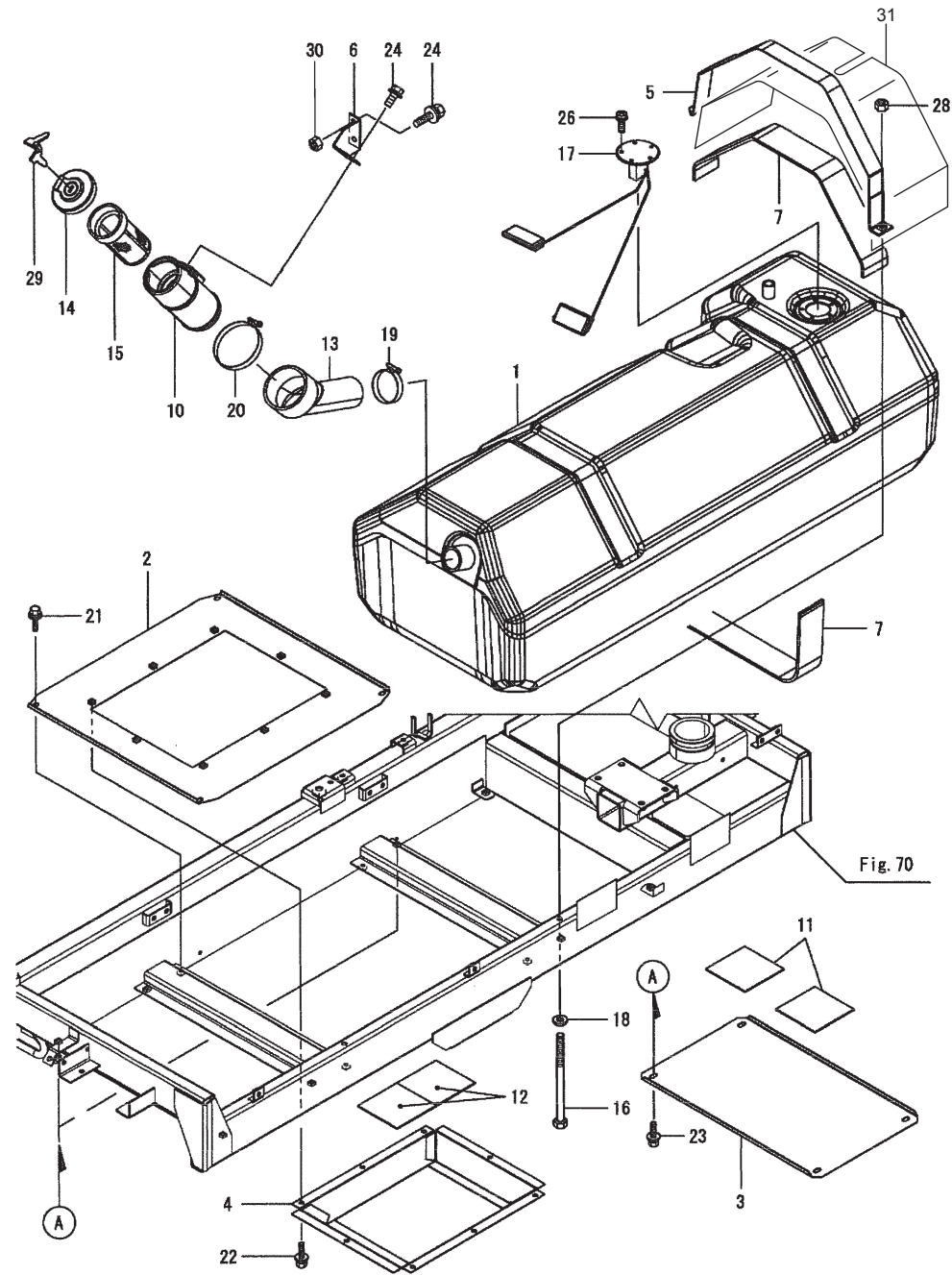
Fig.4. 燃料タンク(1)
