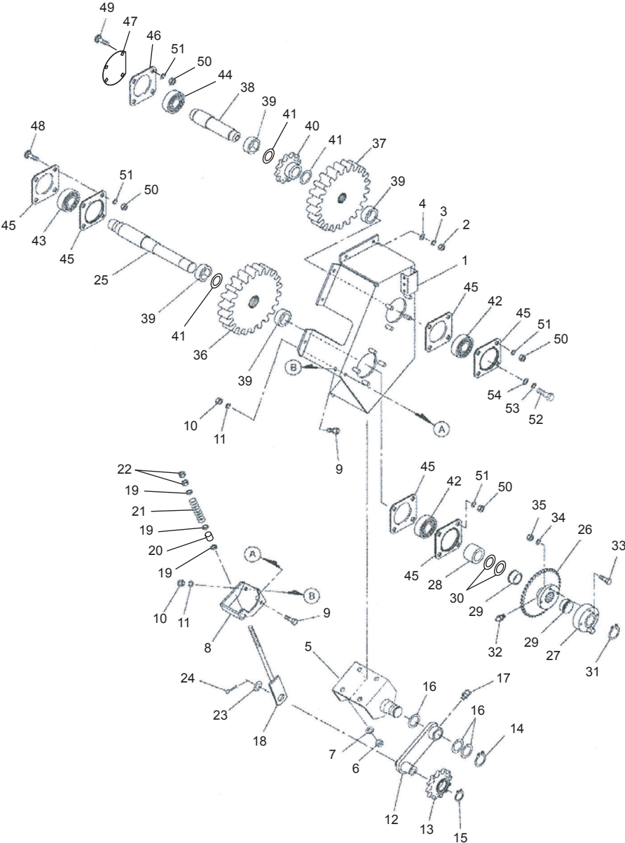
Fig.411. 駆動; 3
