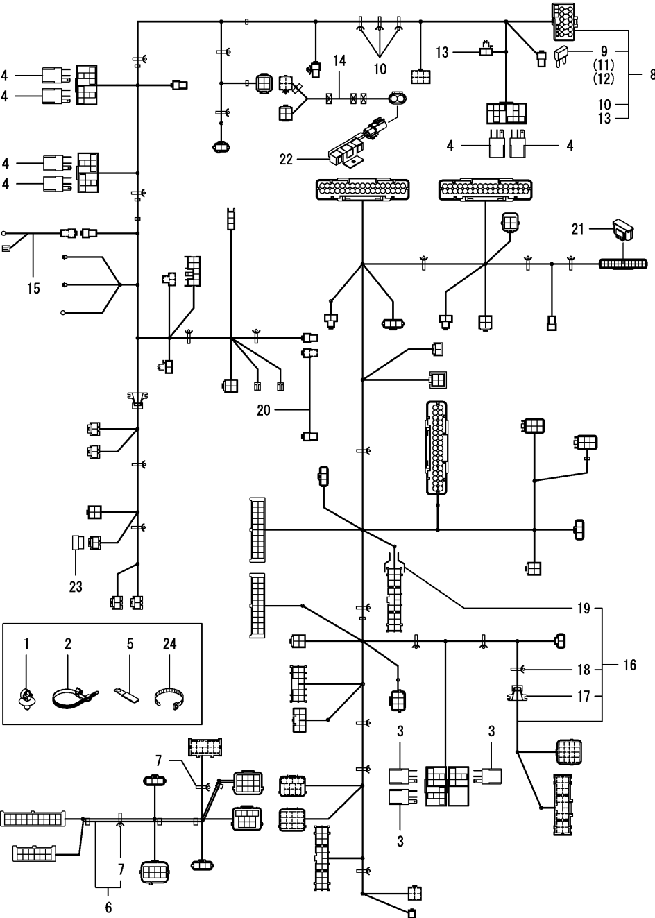
Fig.110. ワイヤーハーネス(キャビン)
