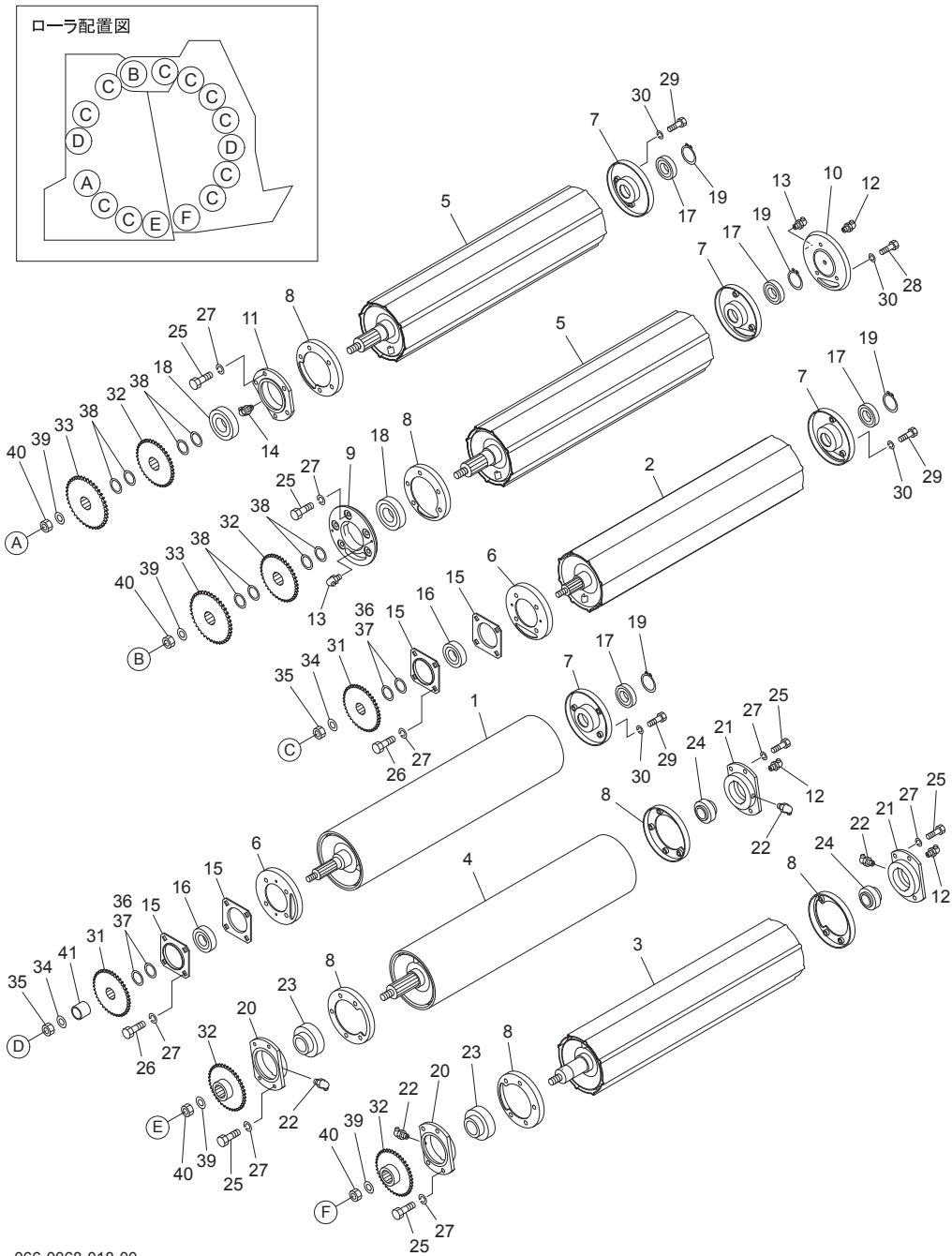
Fig.418. ローラ
