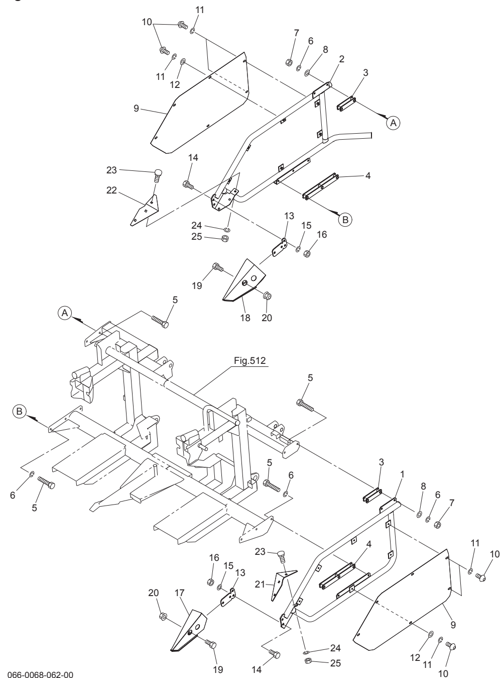
Fig.518. デバイダ
