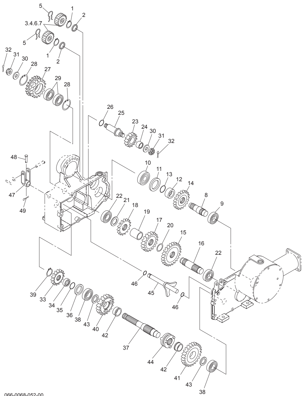
Fig.508. クラッチボックス(2)
