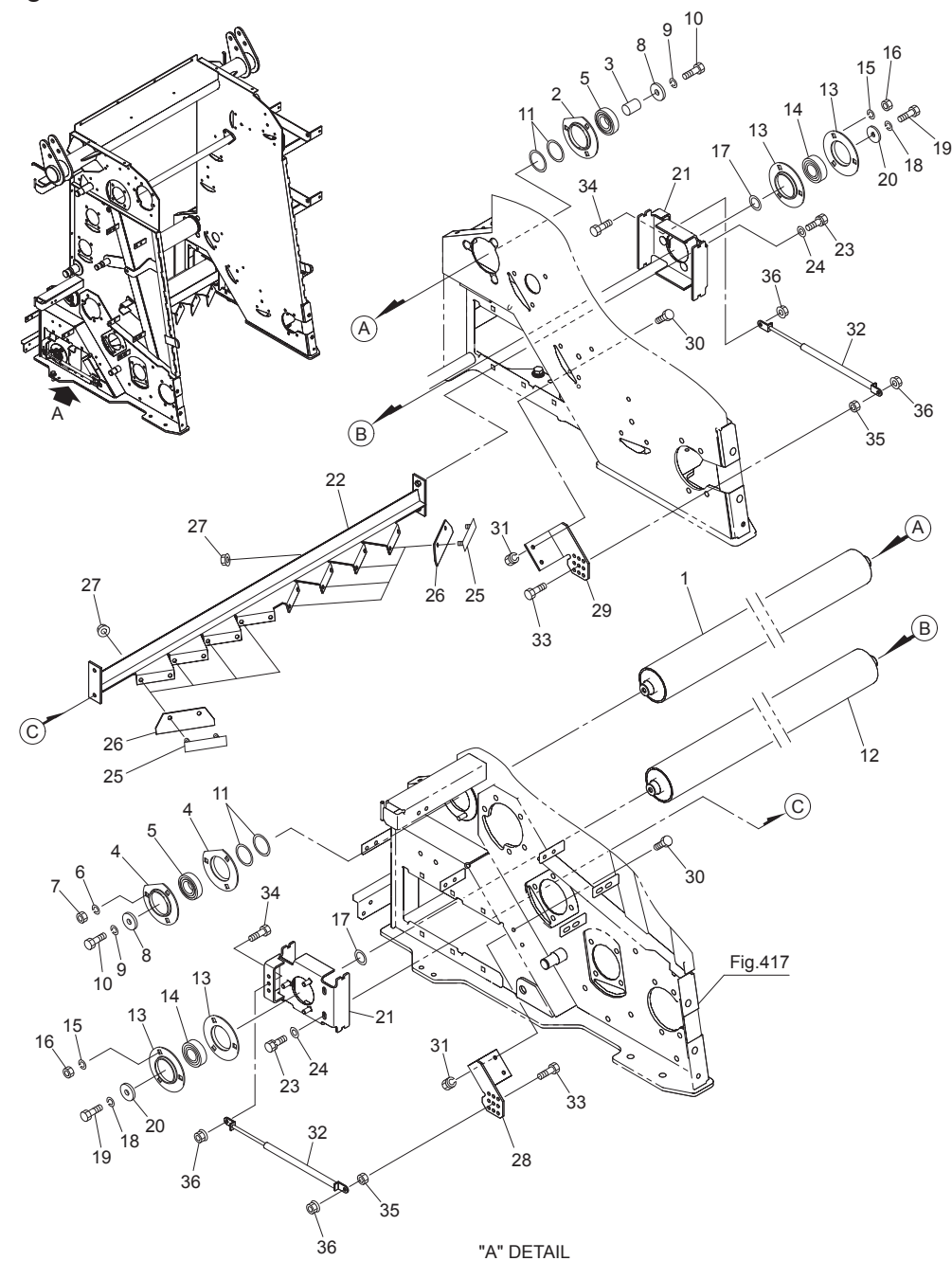
Fig.420. 成形ベルト(1)
