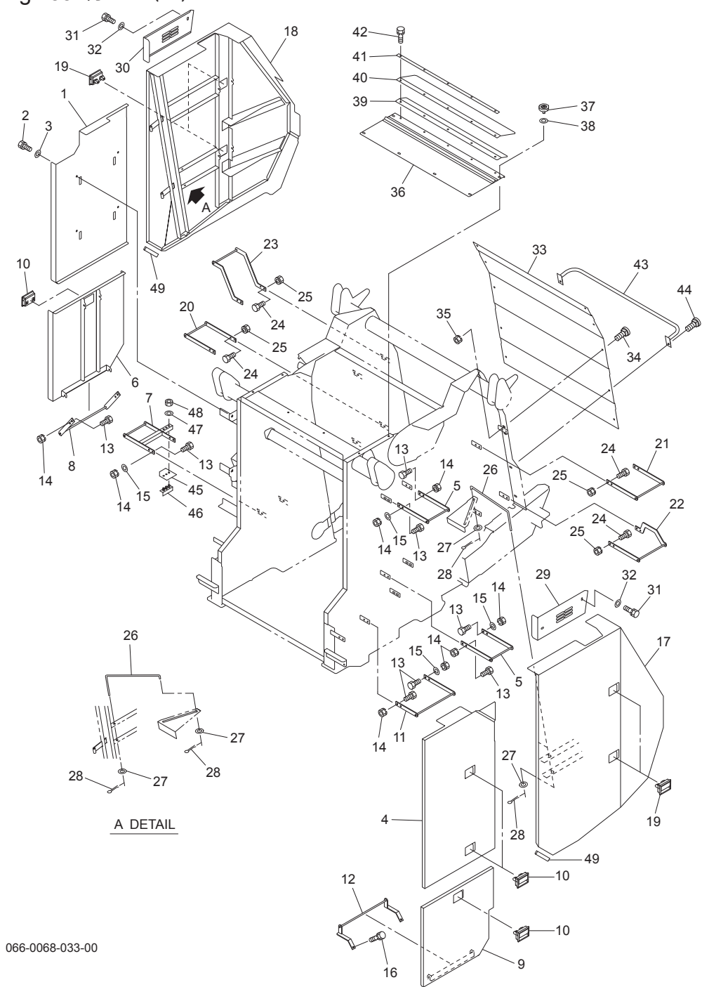
Fig.433. カバー(2)
