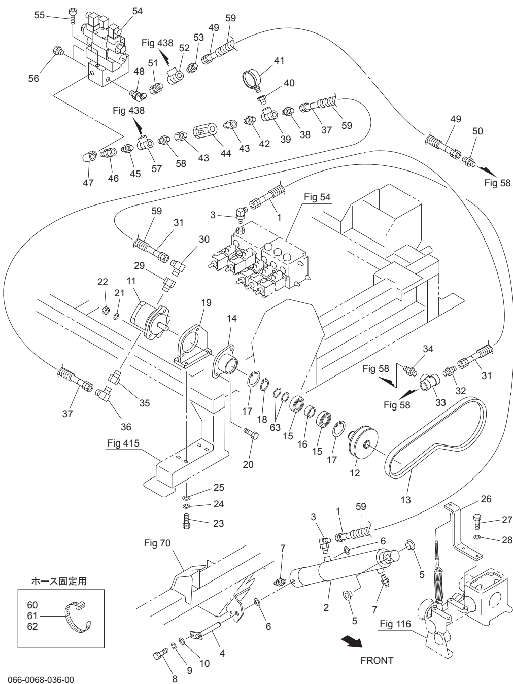
Fig.437. 油圧(メイン)
