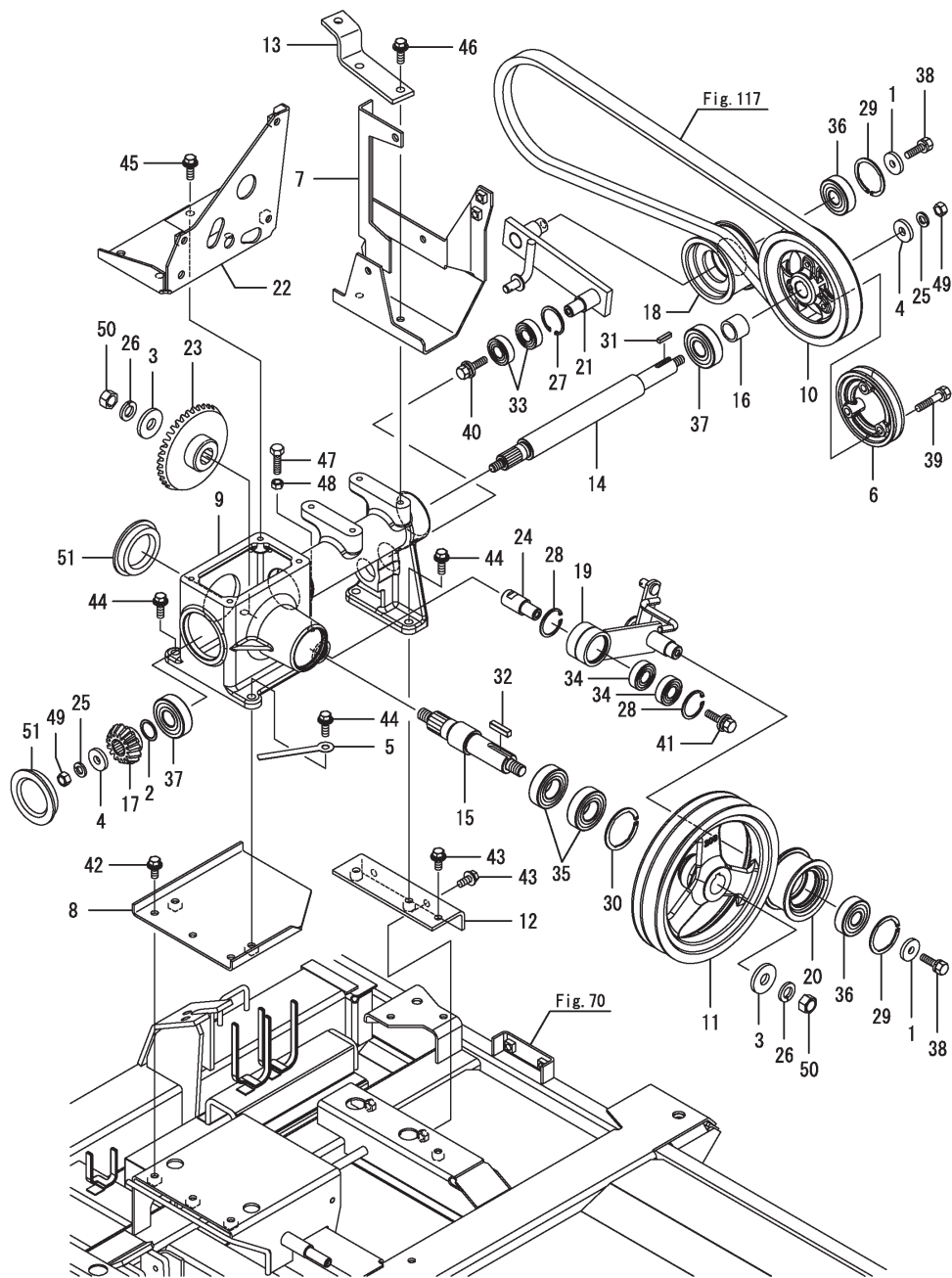
OCNP6-M03520 銘板&付属品部 Fig.116. ポンプ入力(キャビン)
