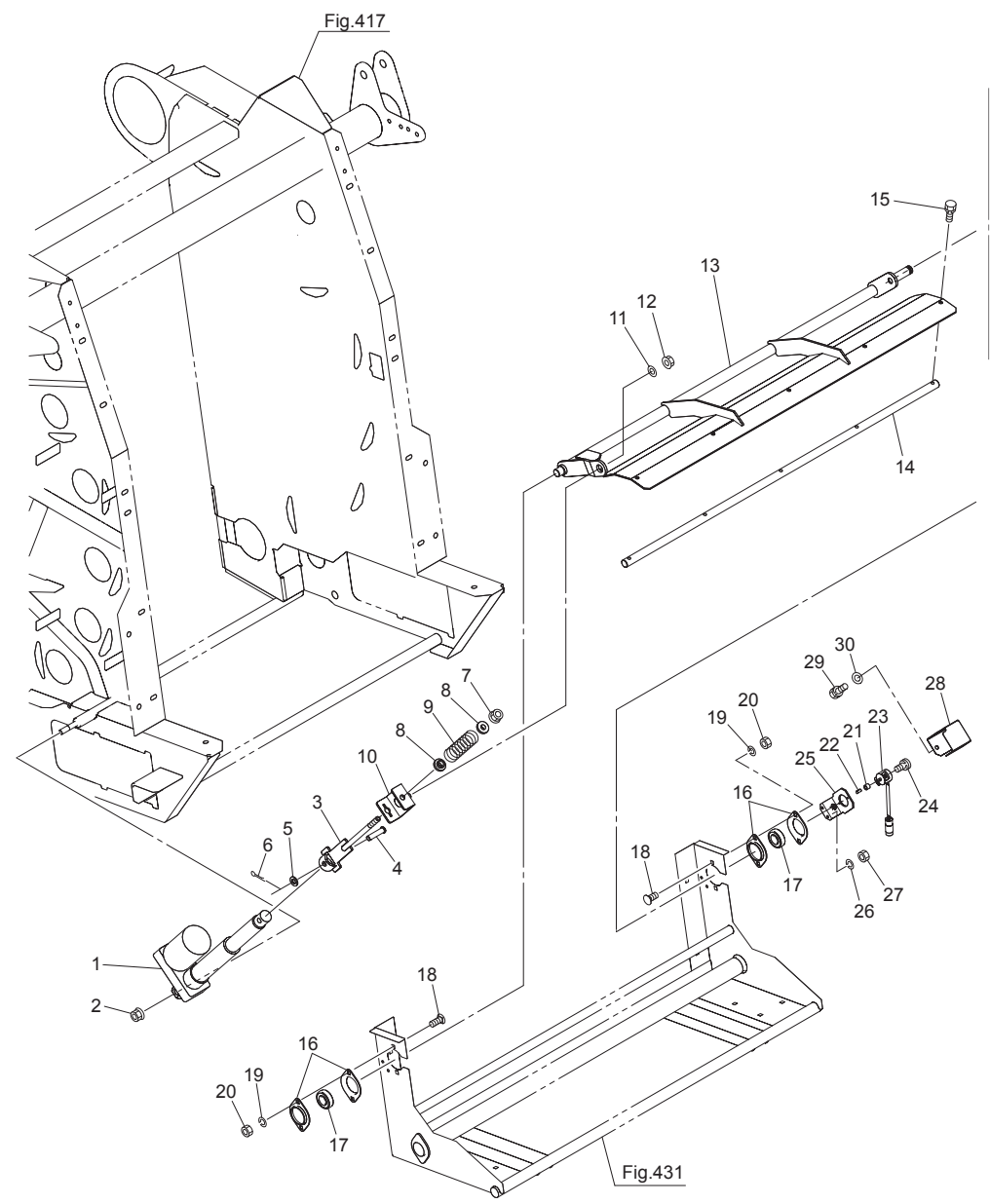
Fig.430. ネットブレーキ
