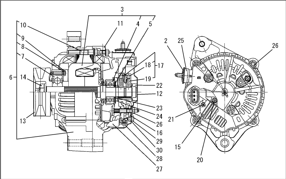
Fig.18. ジェネレータ
