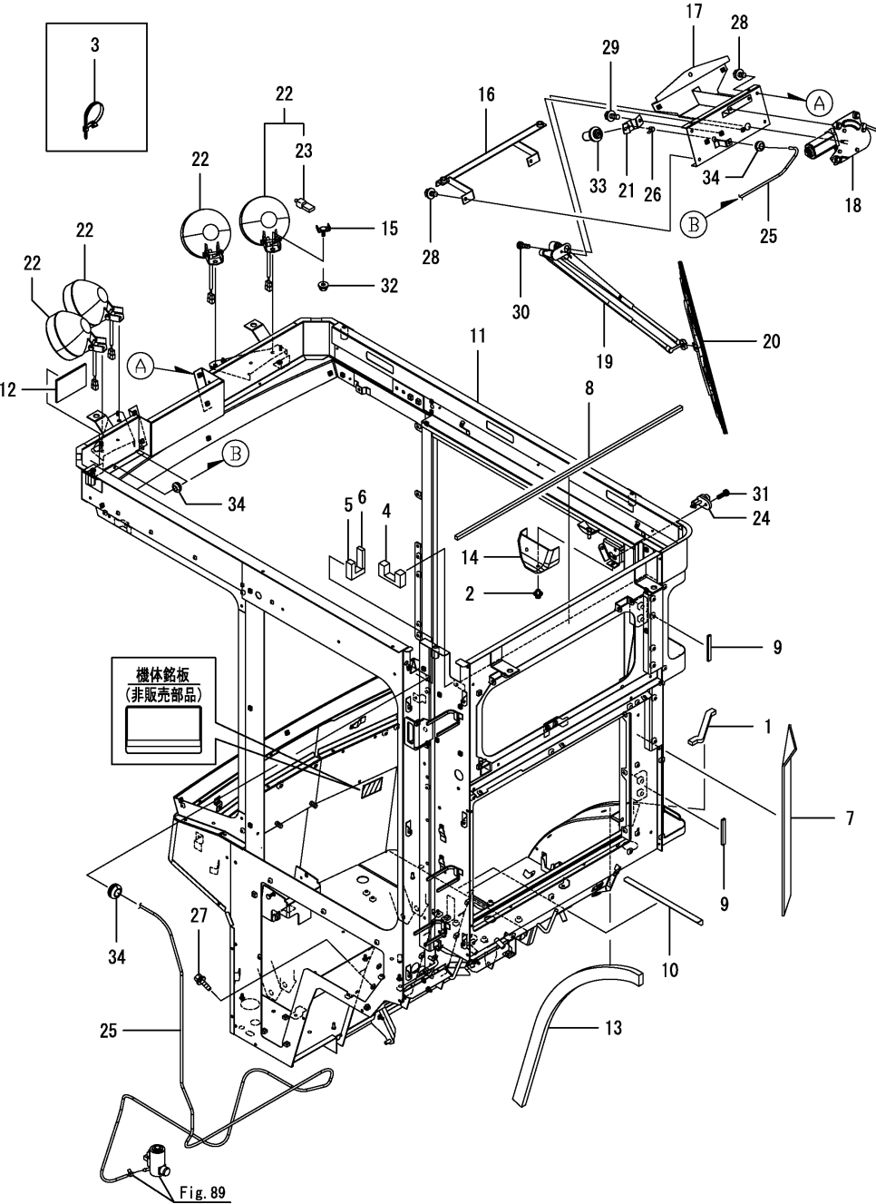
OCNP6-M03520 キャビン部 Fig.88. キャビン(本体)
