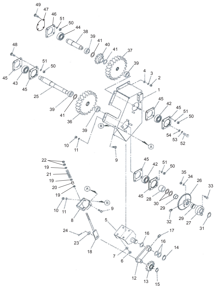
Fig.411. 駆動; 3
