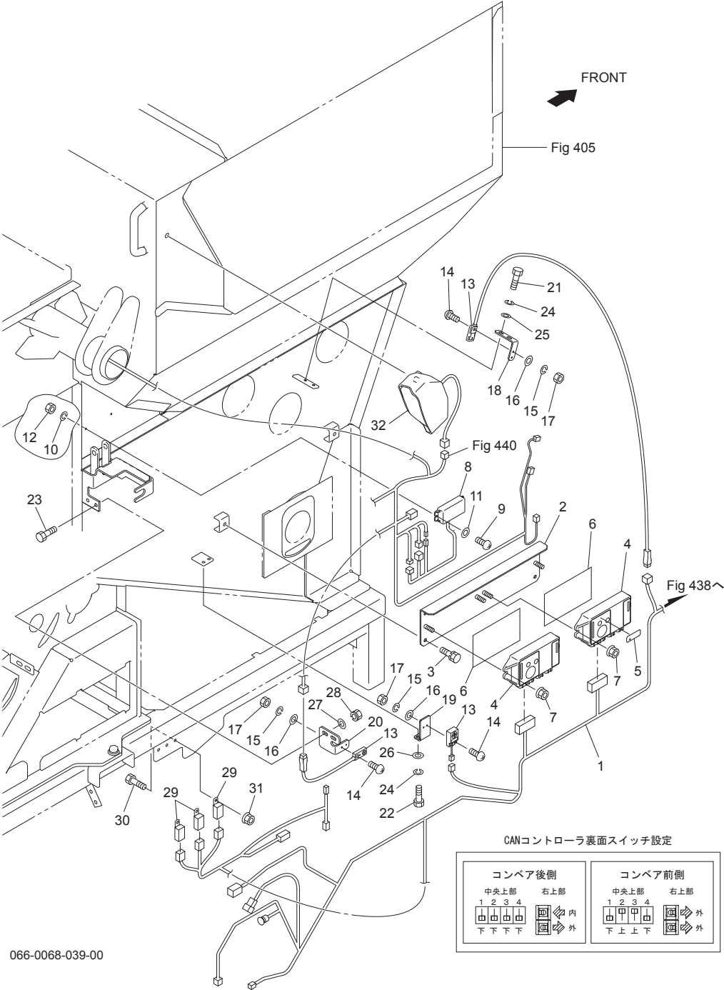
Fig.440. 電装(2)
