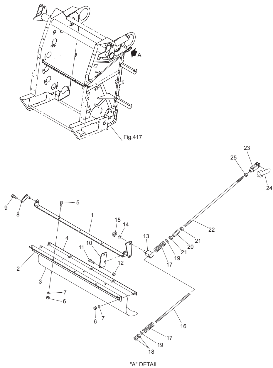
Fig.423. コボレ止め
