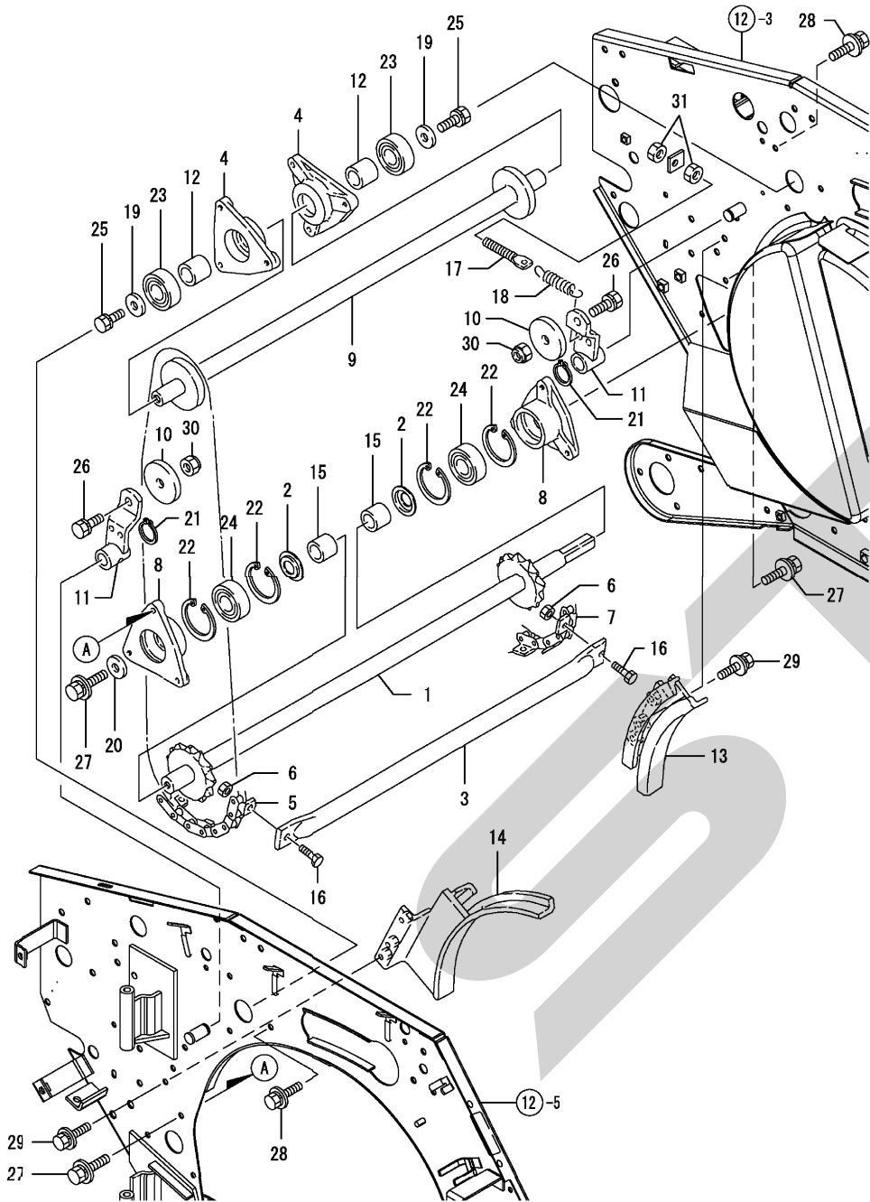
Fig. 13. 上チャンバー
