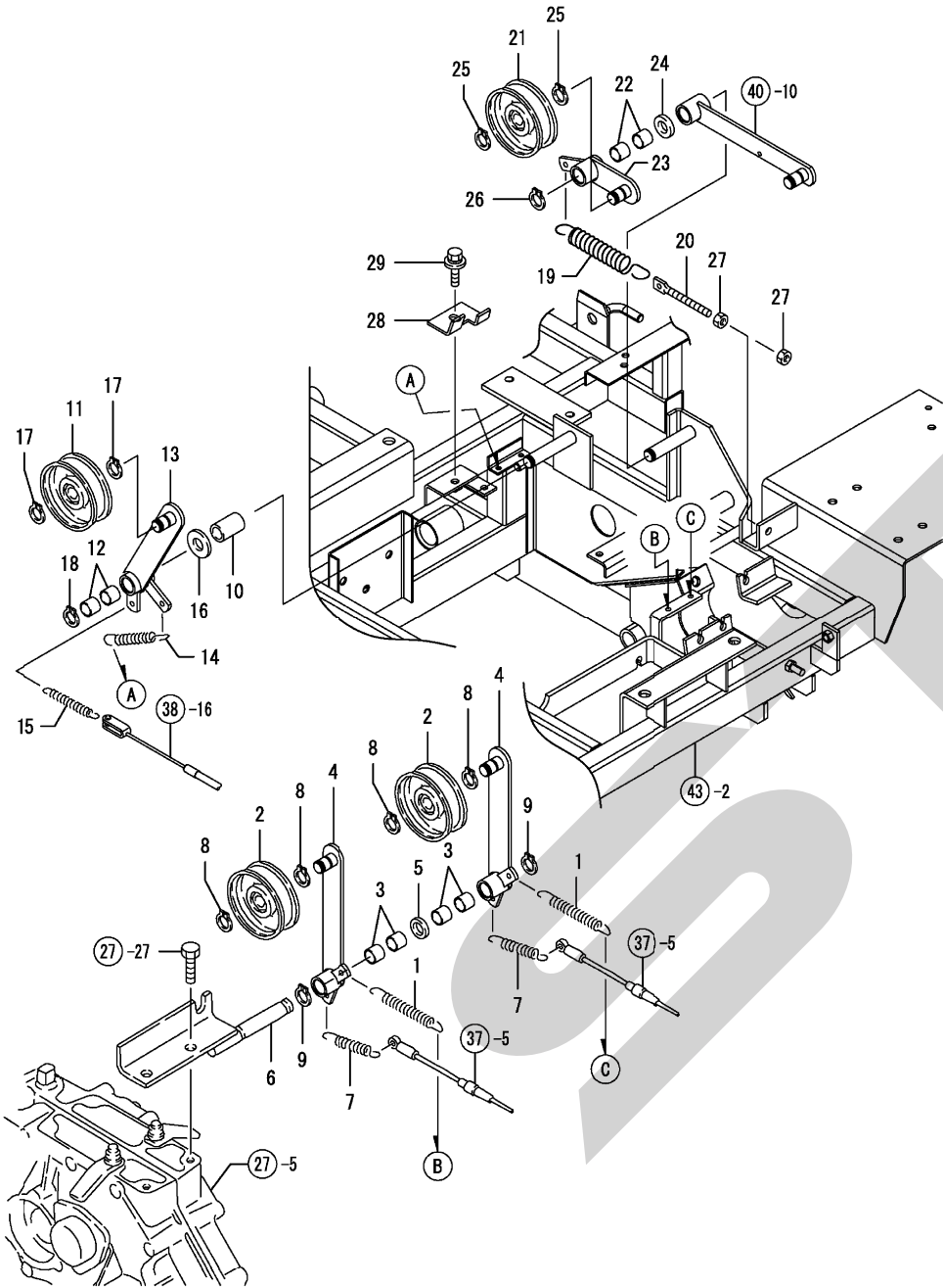
Fig. 26. テンション, 駆動ベルト
