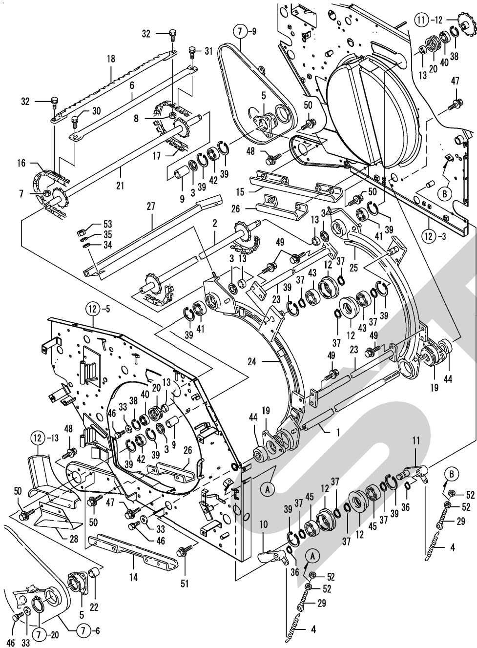
Fig. 14. 下チャンバー
