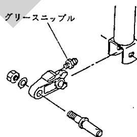
8. ローリンクブラケット
