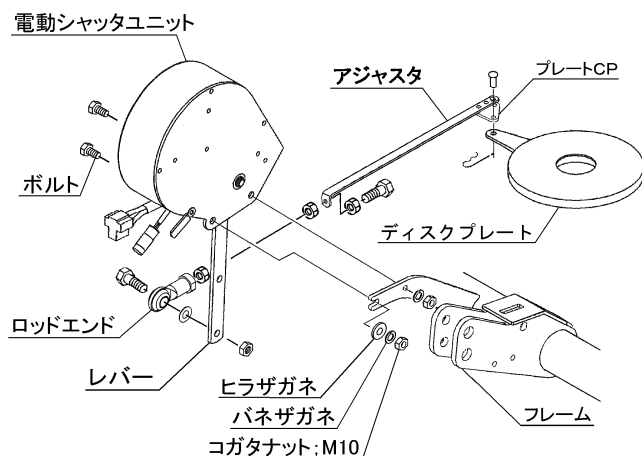
[MBC451P～、MBC601P～、MBC1201P～] スパウトタイプ
