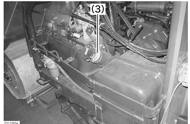
右側面図（カバーを外した状態）
