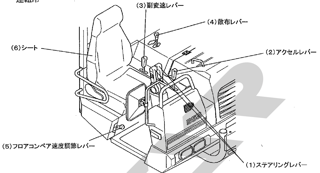
運転席
