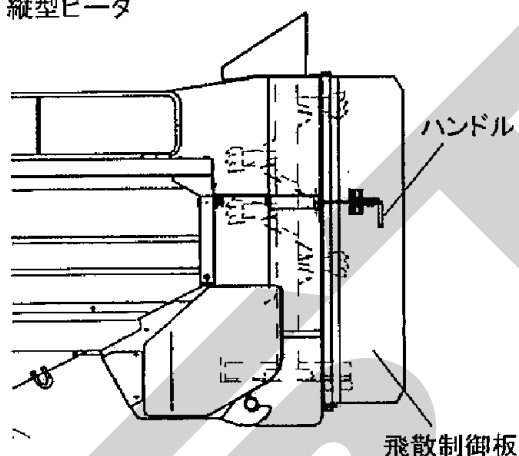
縦型ビータ
