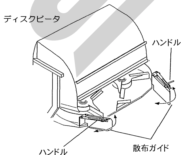
散布ガイド（ディスクビータ 仕様）
