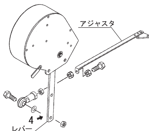
MBC453SE, 453SE-0L MBC603SE, 603SE-0L MBC1203SE
