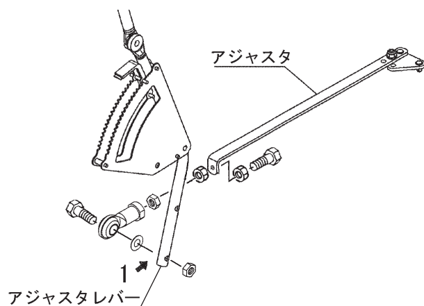
MBC453SM, 453SM-0L MBC603SM, 603SM-0L
