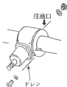
4. トラニオン
