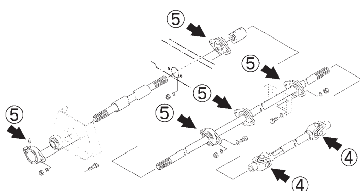
PIC軸関係
