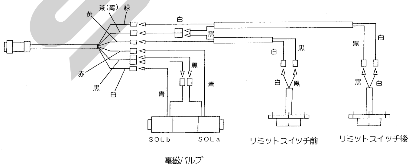
電気配線図
