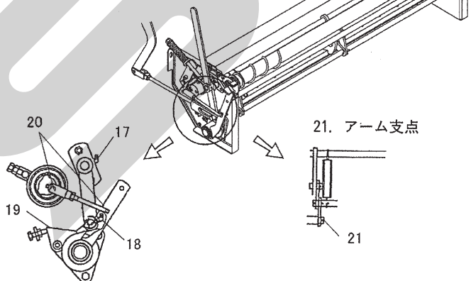
17. ハウジング 18. ラッチ 19. ストップ 20. クランクアーム支点
