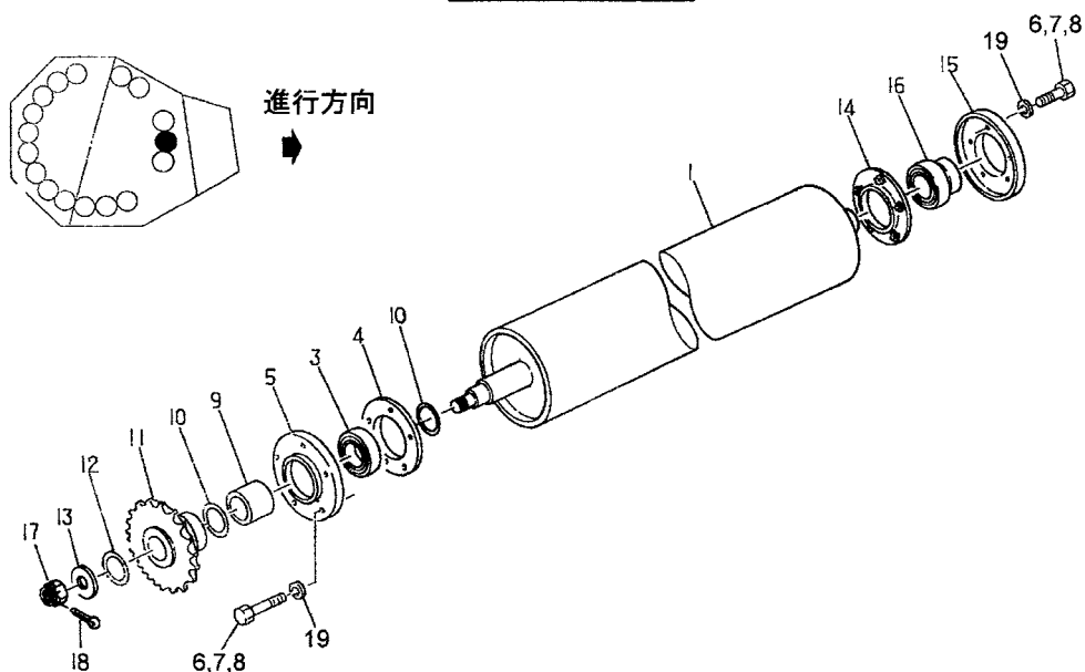
トランスポートローラ; L1
