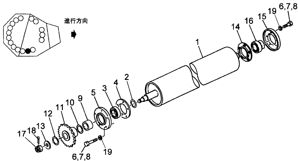
トランスポートローラ；L3
