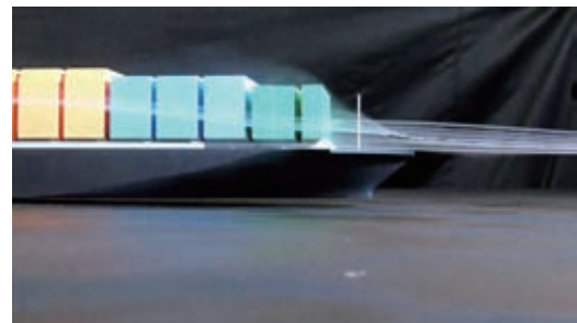
第 7 図 風洞試験における船首まわりの気流の様子 Fig. 7 Air flow around bow in wind tunnel test
