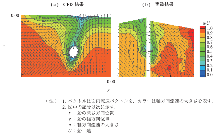
第 3 図 ツインスケグまわりの流れの CFD と実験結果との比較 (プロペラ位置断面) Fig. 3 CFD results for flow around a twin-skeg hull compared with experimental data ( Propeller section )
