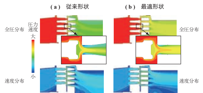
第 12 図 従来形状および最適形状の流れ場比較 Fig. 12 Comparison of flow distribution for original and optimal shape
