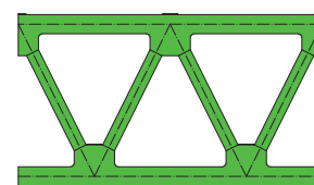
基本パネル 〈パネル長：4m〉
