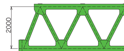
端部パネル 〈パネル長：5m〉
