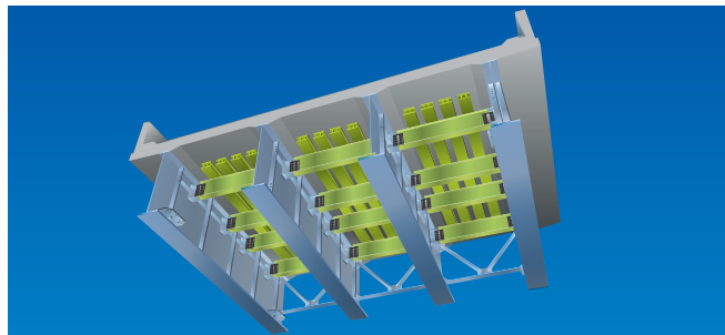
FSグリッド(床版延命化技術)
