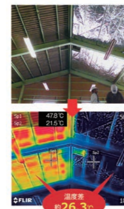
温度差 約26.3℃
