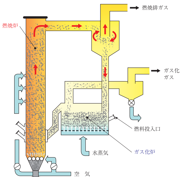
二塔式ガス化炉の構造と原理
