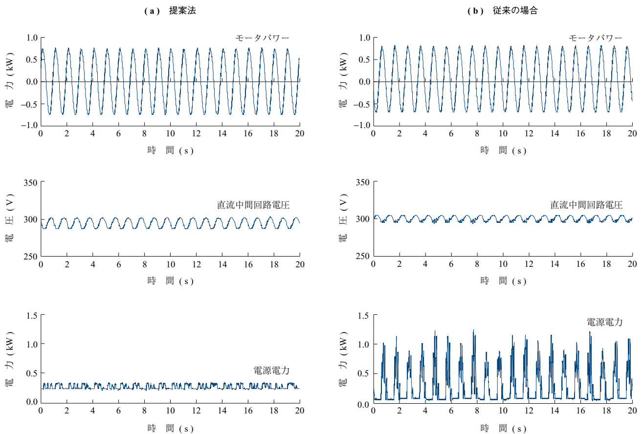
第 11 図 一次側電力の実測結果による比較 Fig. 11 Comparison of measured primary side electric power
