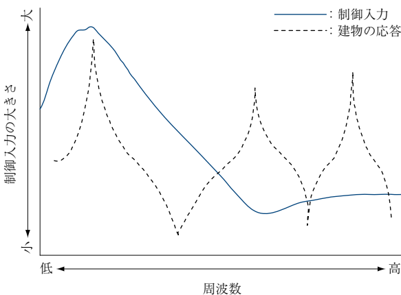
第 2 図 制御器の概念 Fig. 2 General idea of controller
