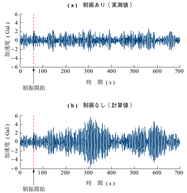
第7図 2009年の台風19号での制振効果 Fig. 7 Control performance during Typhoon No. 19 in 2009
