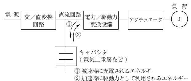
第10図 回生電力再利用の基本概念 Fig. 10 General idea of electric power regeneration for reuse
