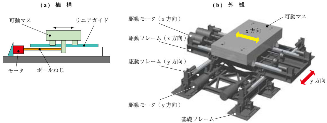
第 1 図 レール型フル・アクティブ式制振装置 Fig. 1 A rail-guided fully active mass damper system
