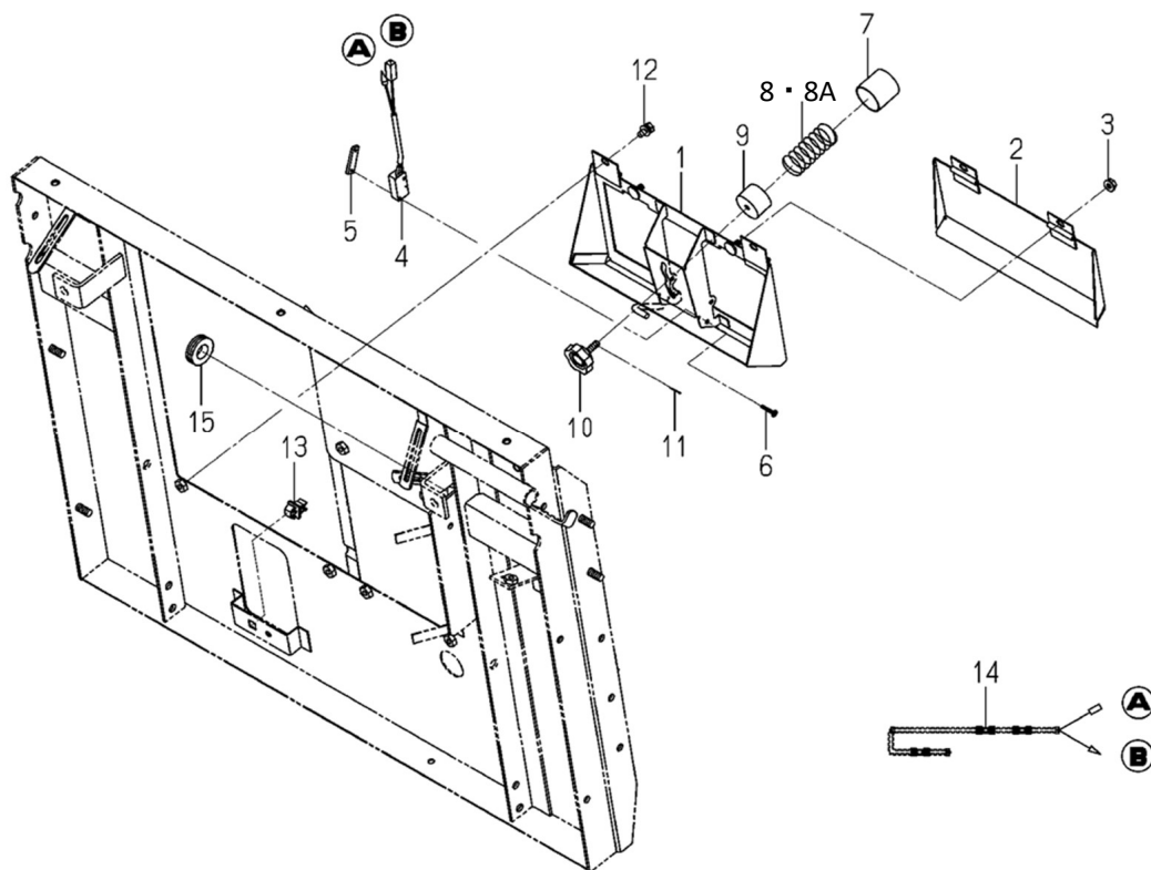
FIG.409 センサー SENSOR SYSTEM
