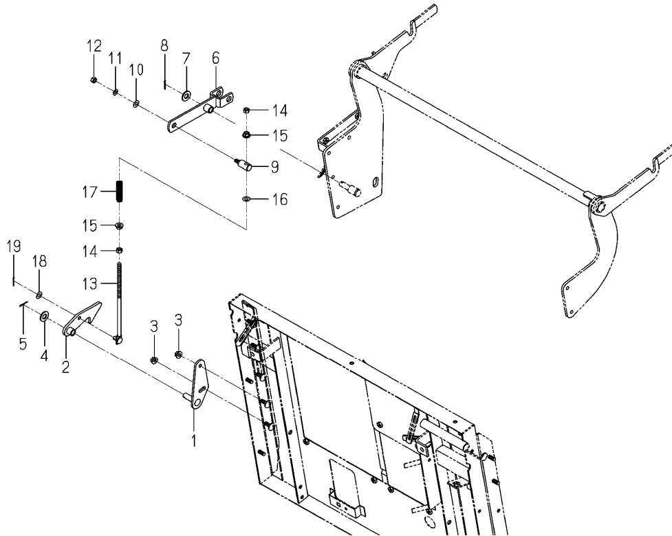
FIG.404 ロックシステム LOCK SYSTEM(A TYPE)
