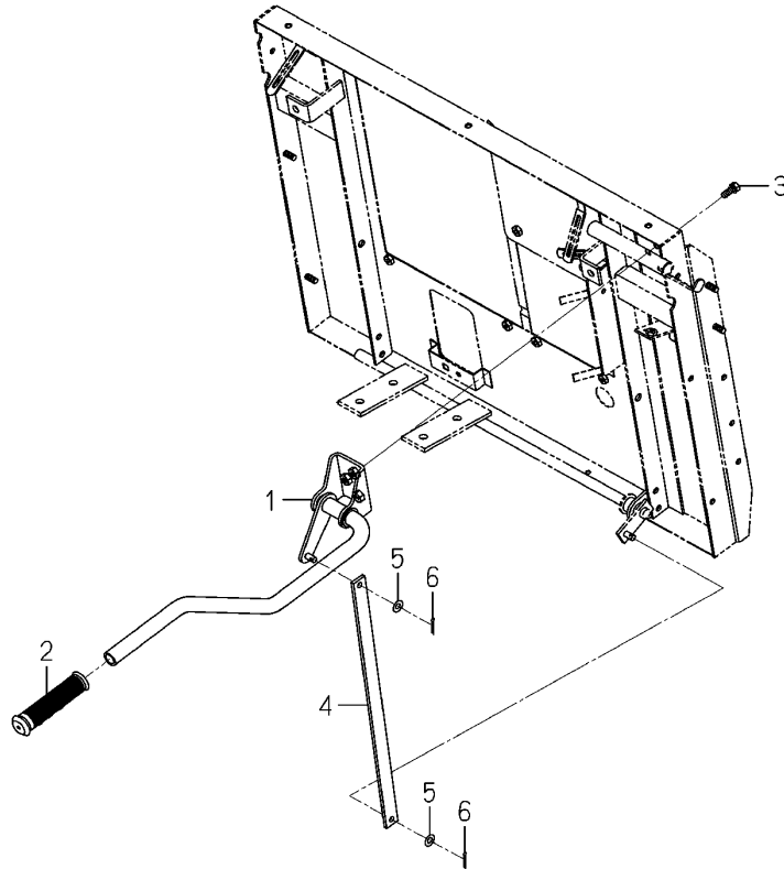
FIG.408 レバー LEVER(CLEANER)SYSTEM
