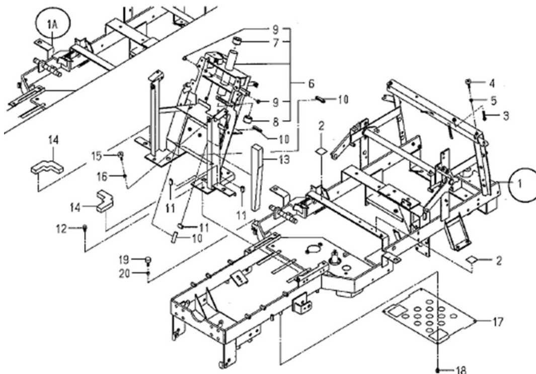
FIG.221 フレーム FRAME(MAIN)SYSTEM
