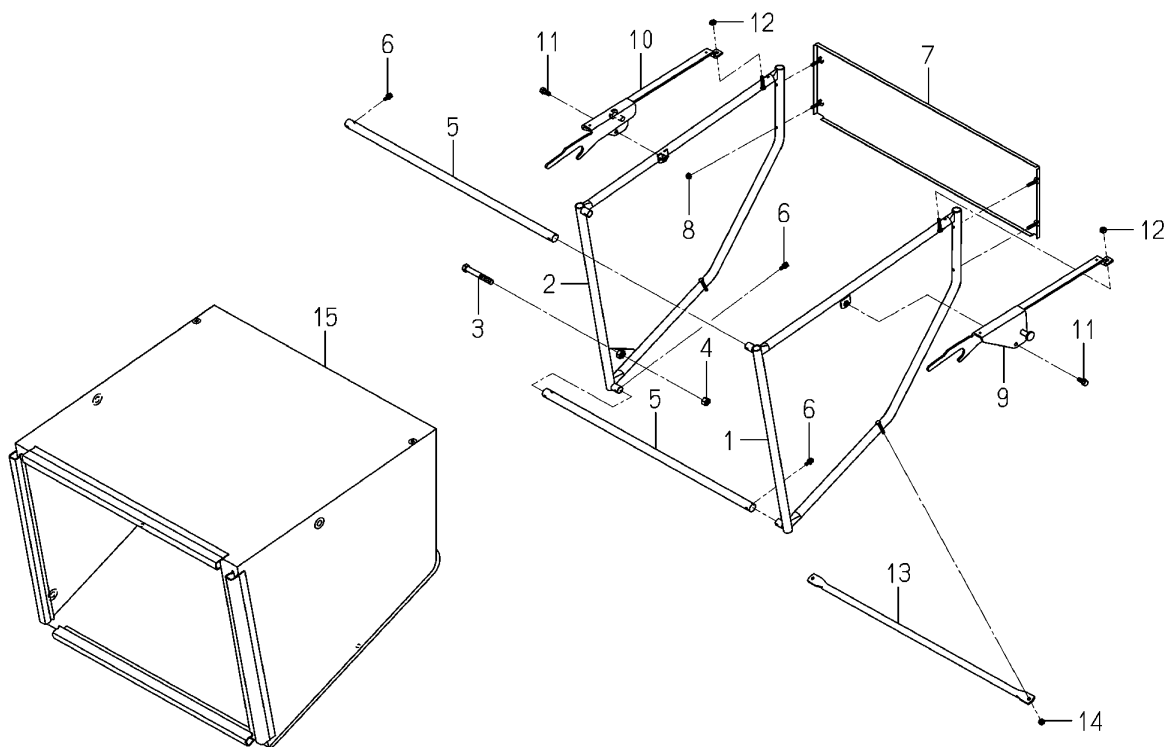
FIG.406 コンテナ CONTAINER SYSTEM
