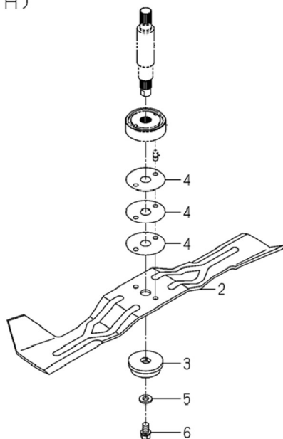
FIG.304-1 ブレード BLADE SYSTEM 適合機種：#125 ~ 号機
