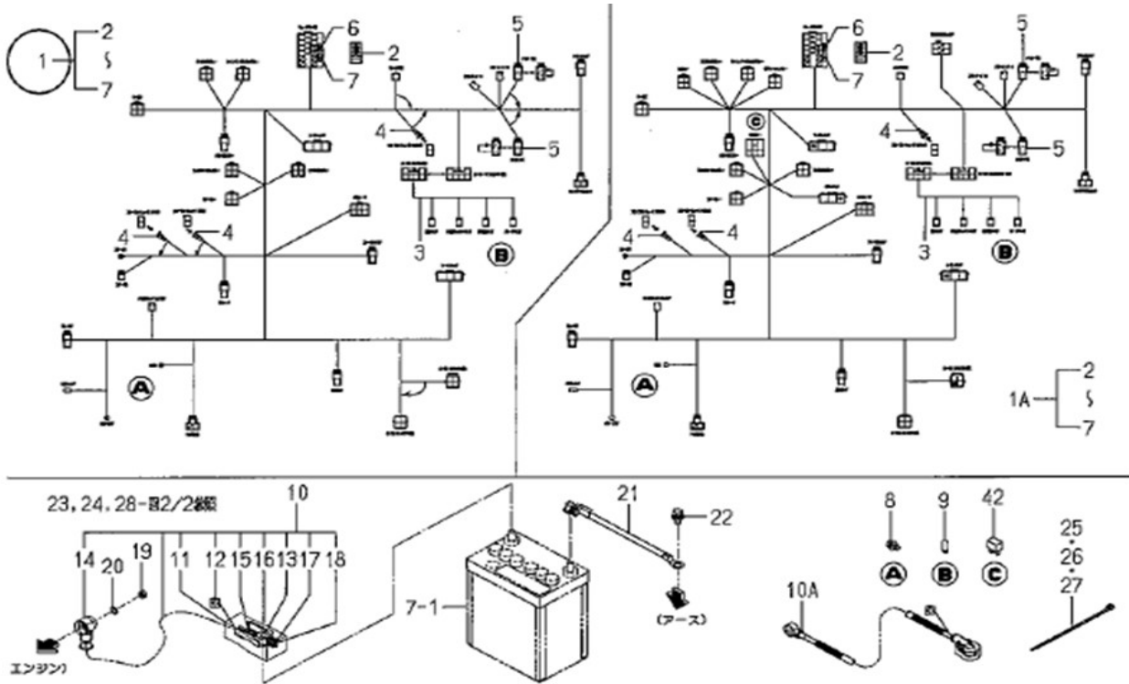
FIG.236 ハーネス (図1/2) HARNESS SYSTEM
