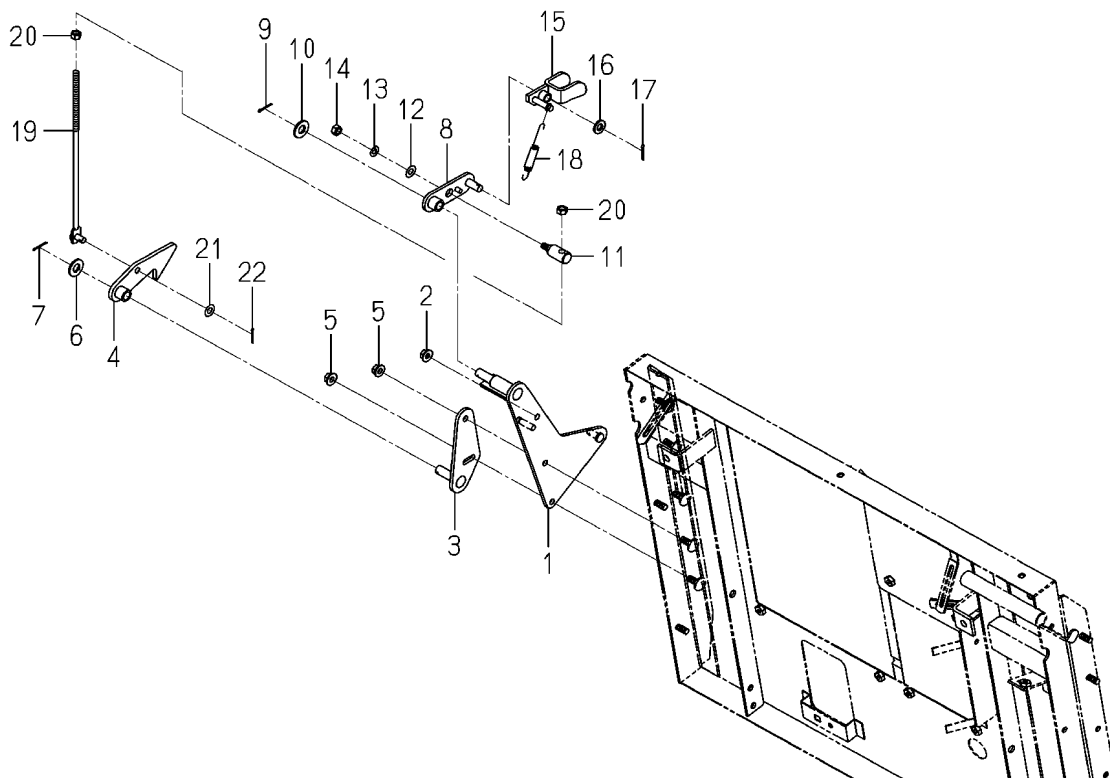
FIG.402 ロックシステム LOCK SYSTEM(EXCEPT A TYPE)
