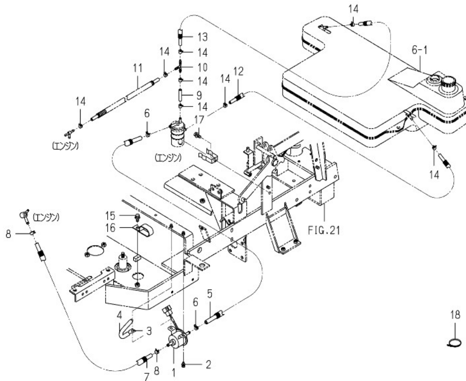
FIG.205 ポンプ PUMP(FUEL)SYSTEM
