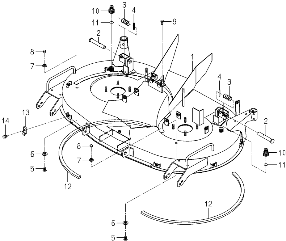
FIG.305 デッキ DECK(MOWER)SYSTEM
