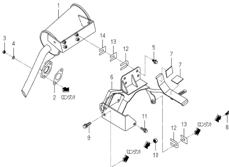
マフラ MUFFLER SYSTEM
