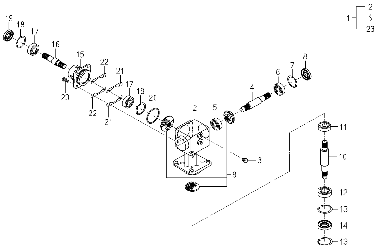
FIG.313 ケース CASE(BEVEL)ASSY(REPAIR)(1/2)
