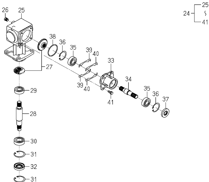
FIG.313 ケース CASE(BEVEL)ASSY(REPAIR)(1/2)
