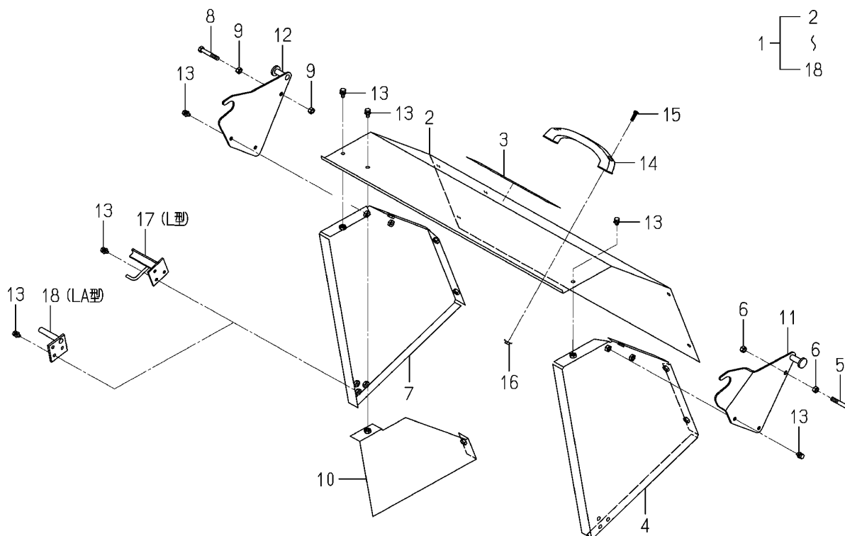
FIG.415 デフレクタSET(オプション) DEFLECTOR SET(OPTION)
