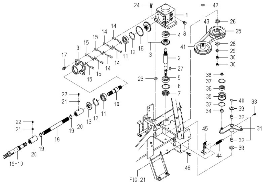
FIG.210 メタル METAL(COUNTER)SYSTEM
