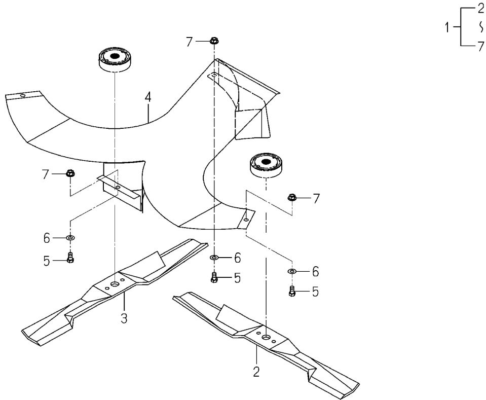
FIG.314 マルチング MULCHING(OPTION)
