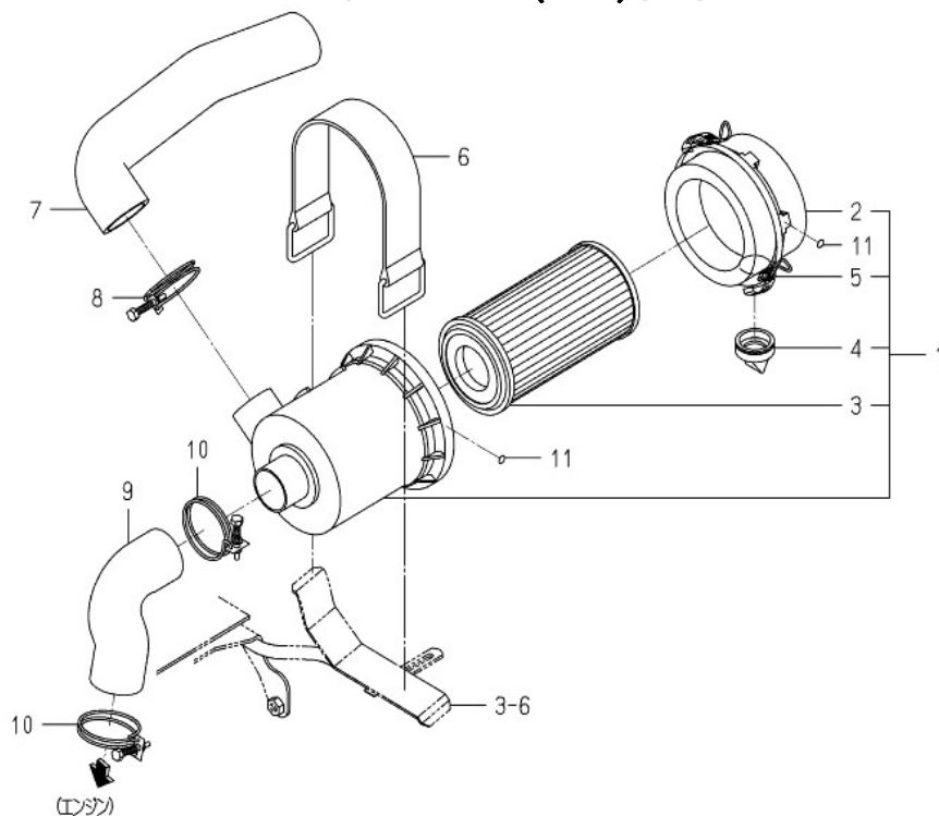
FIG.204 クリーナ CLEANER(AIR)SYSTEM
